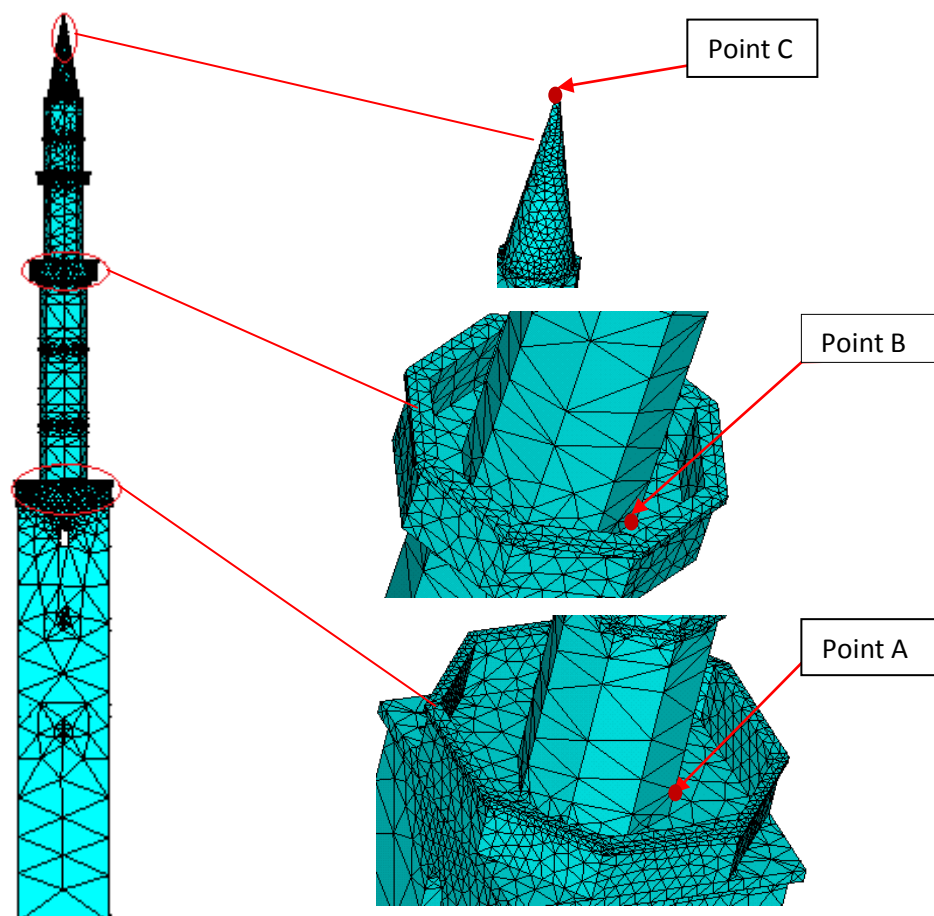
Figure 5.6 : Positions des 3 points de référence.
