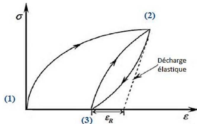
Figure 2.6 : L'effet caoutchoutique (Patoor et al, 2006b).
