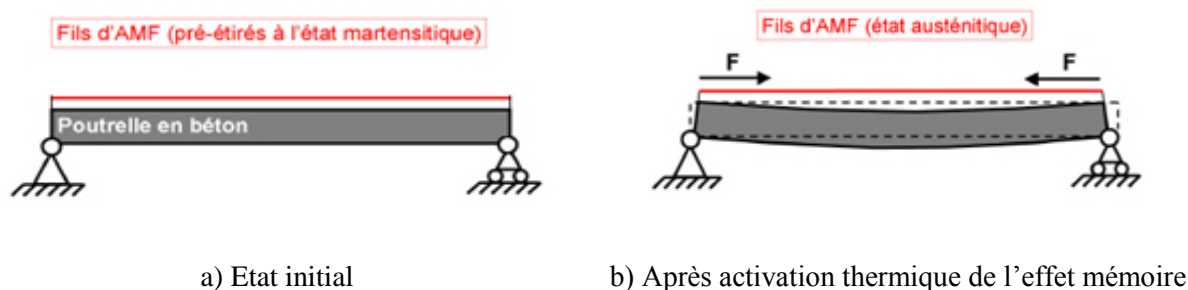
Figure 2.11 : Utilisation des barres en AMF pour créer une précontrainte de flexion dans des poutrelles en béton.
