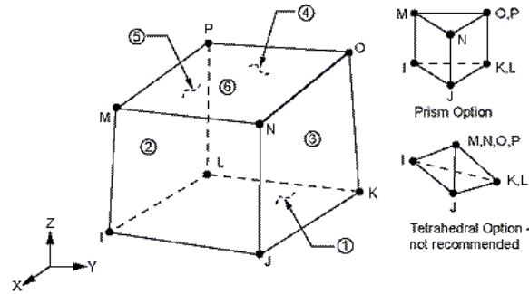
Figure 5.4 : Structure géométrique du SOLID 185.
