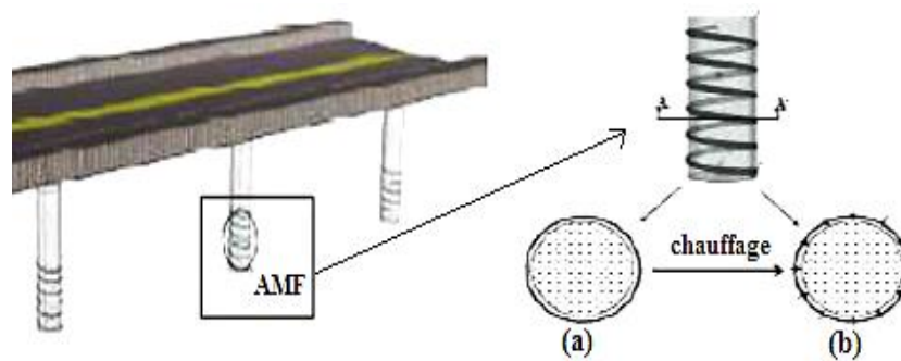
Figure 2.13 : Schéma de précontrainte de cylindres en béton par AMF : a) Avant chauffage. b) Après chauffage.
