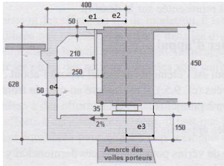
Fig.8.3 : coupe schématique d'une tête de culée
