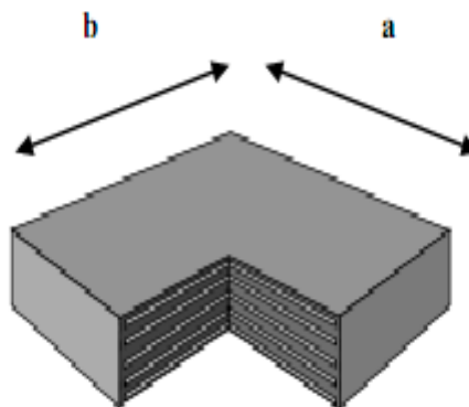
Fig.7.1: Appareil d'appui en néoprène fretté
