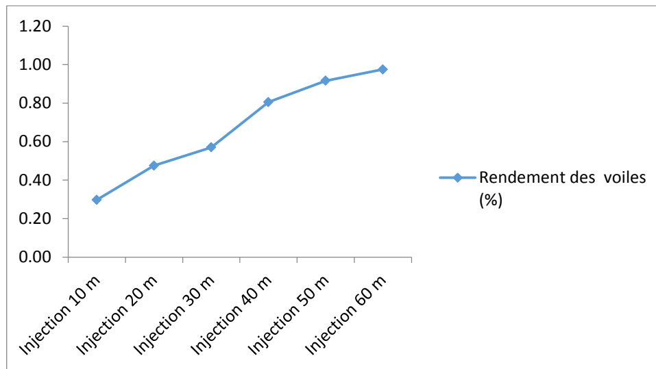
Figure 4.15 : Influence des profondeurs des deux voiles d'injection sur leurs rendements
