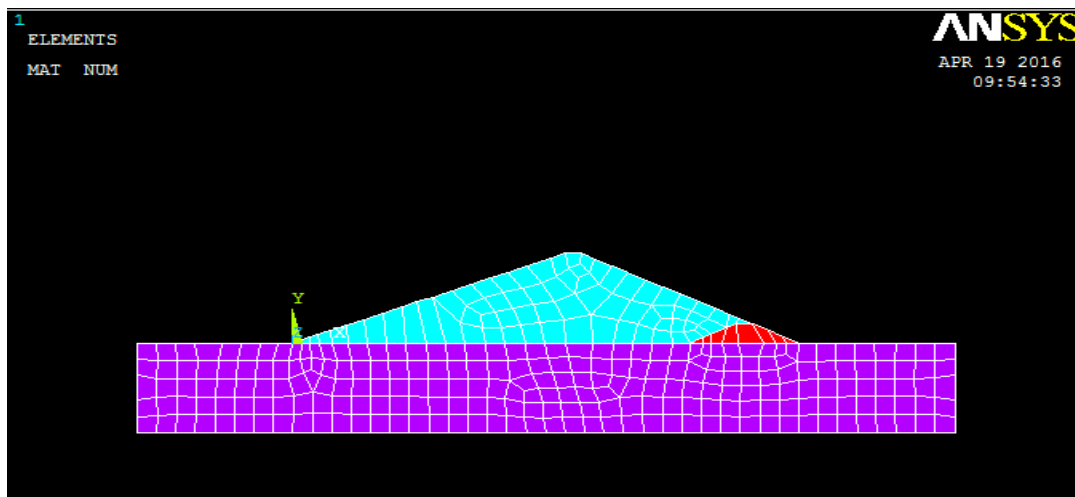
Figure 4.6 : Discrétisation du barrage
