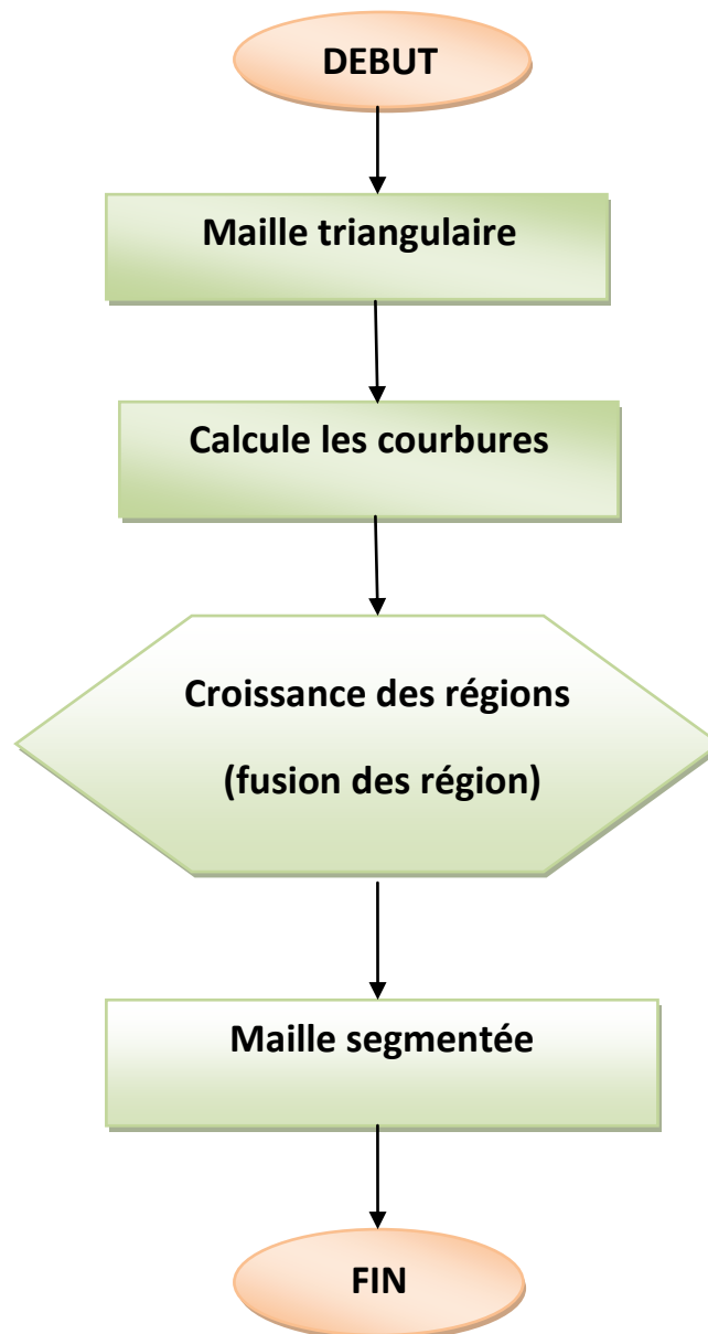
Figure IV.1 : Organigramme de la méthode implémentée.
