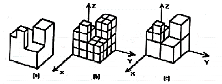
Figure I.9 : Exemple de modélisation par énumération spatiale et arbre octal
