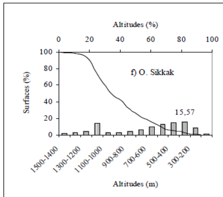
Figure II.3 : Courbe Hypsométrique et histogramme de fréquences altimétriques de sous Bassin de Sikkak [19].
