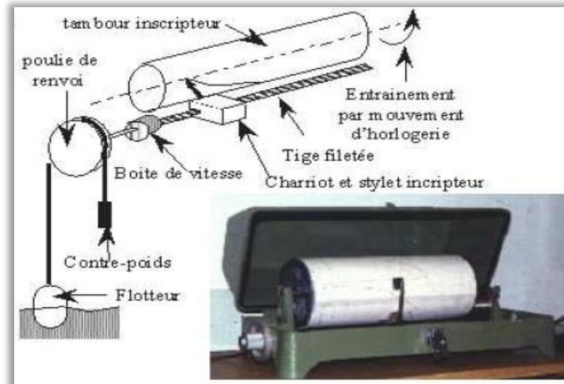
Figure III.5 : Photo d'un limnigraphe à flotteur [27].
