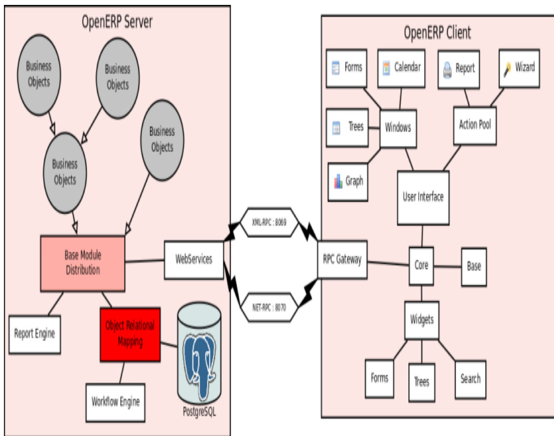
Figure I.1 : l'architecture technique d'ODOO [Open, 2012]
