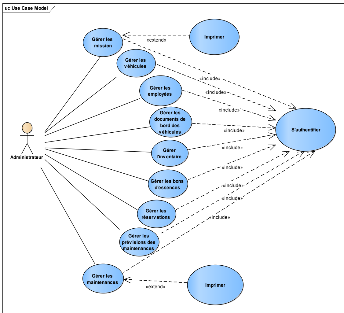
Figure II.1 : diagramme de cas d'utilisation relatif au gestionnaire du parc
