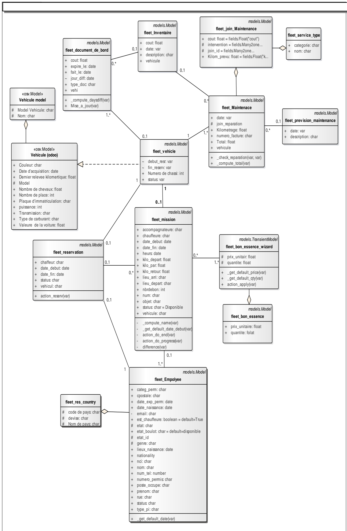
Figure II.8: Le diagramme de classe
