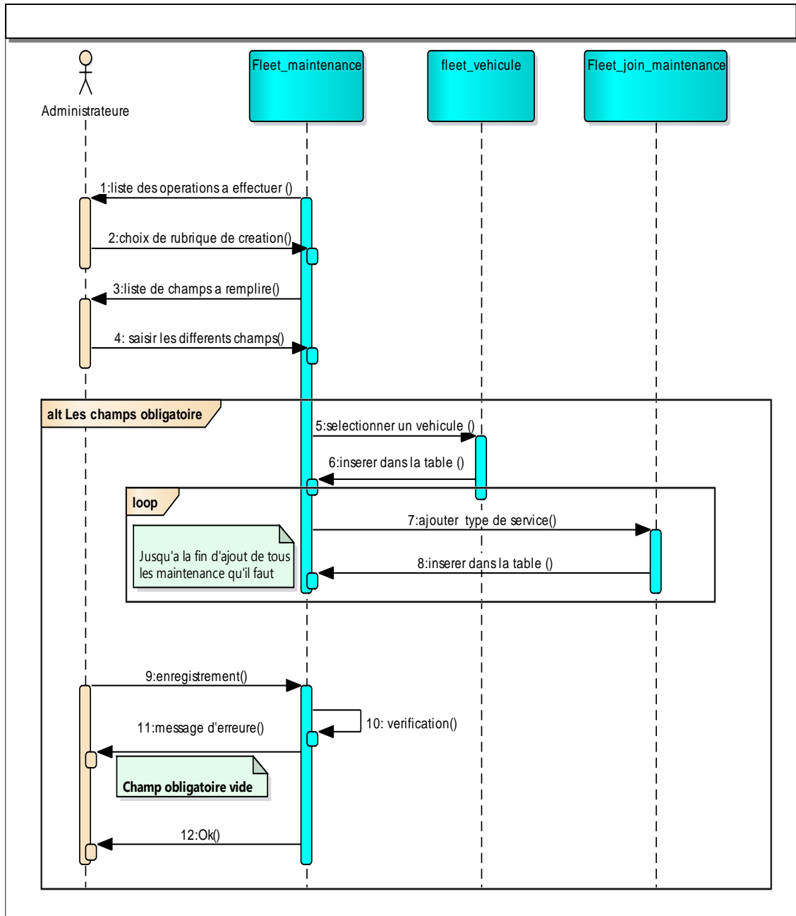
Figure II.6: diagramme de séquence scénario création d'une maintenance
