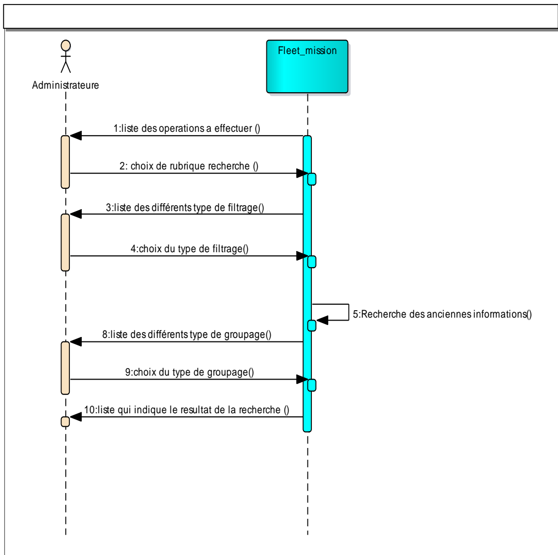
Figure II.3 : diagramme de séquence scénario de modification d'une mission
