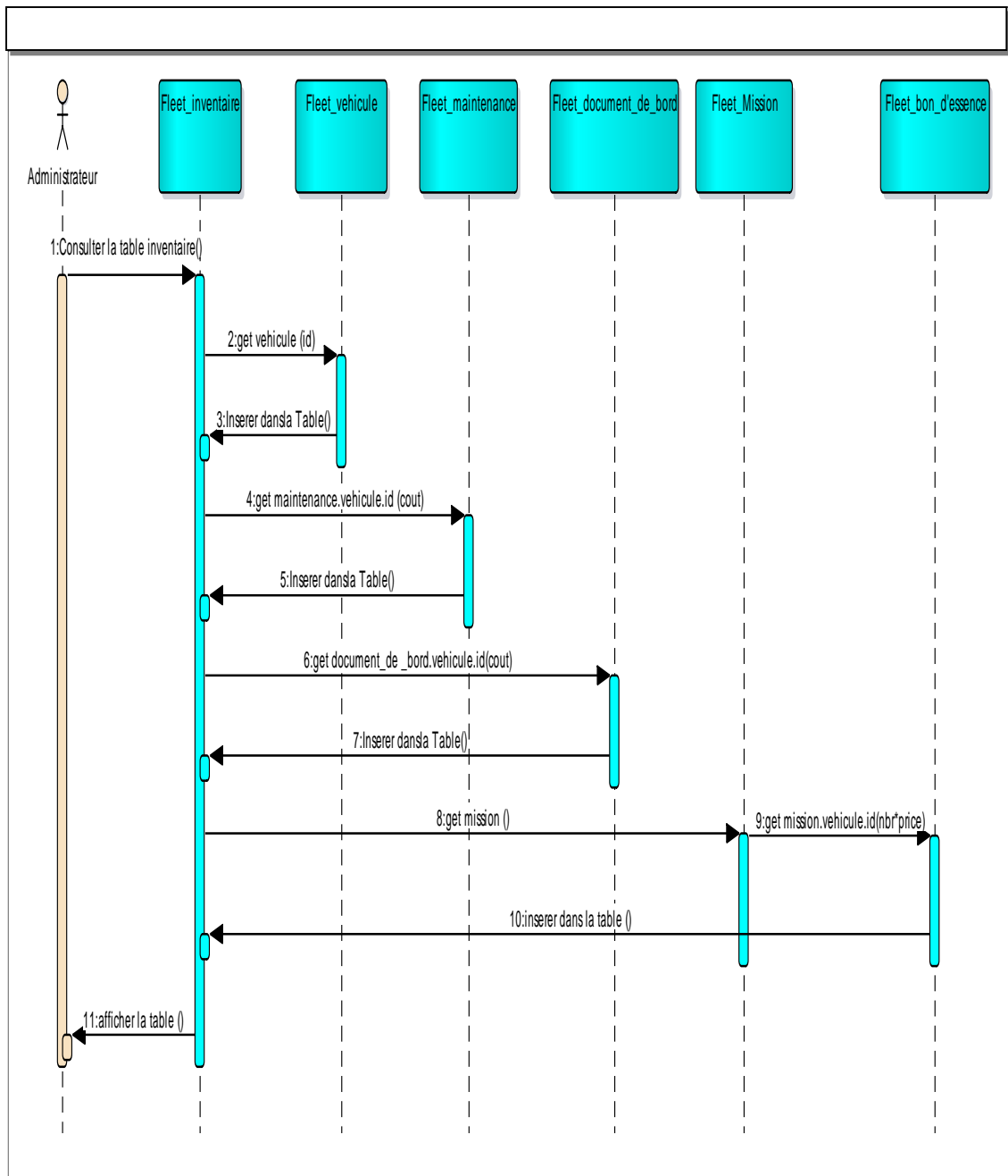
Figure II.5: diagramme de séquence scénario consultation de la table inventaire
