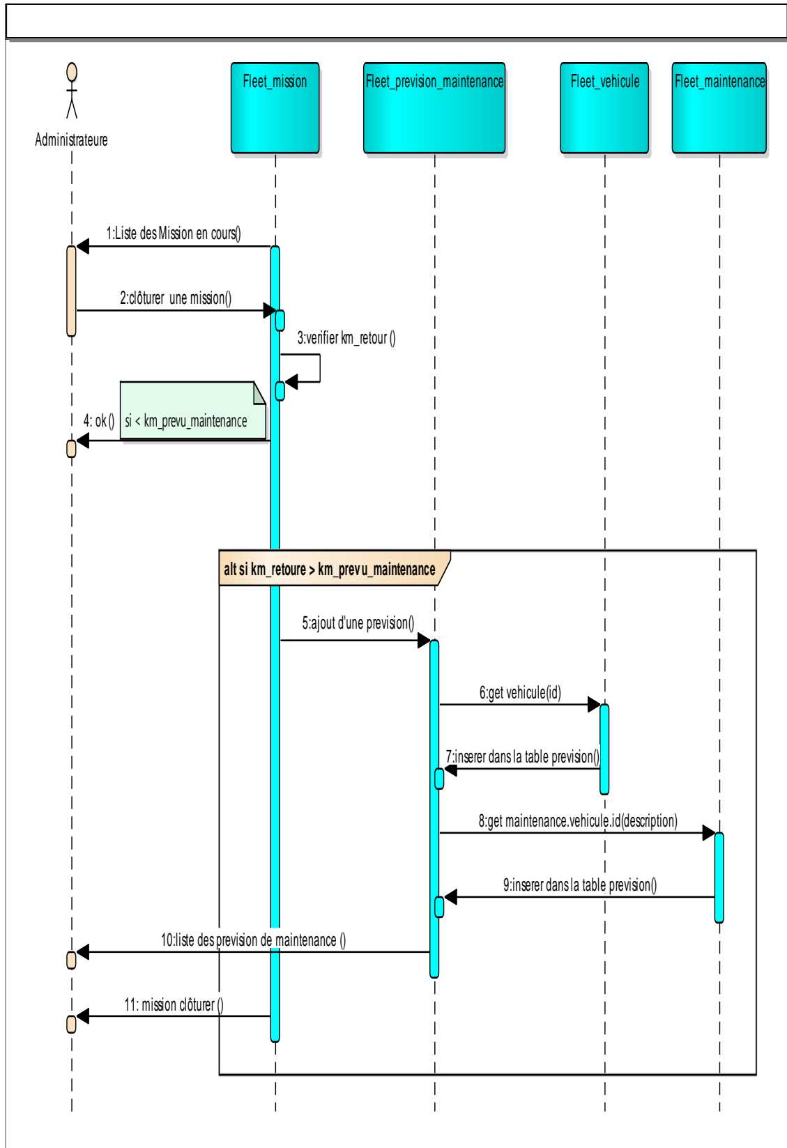
Figure II.7: diagramme de séquence scénario prévision d'une maintenance
