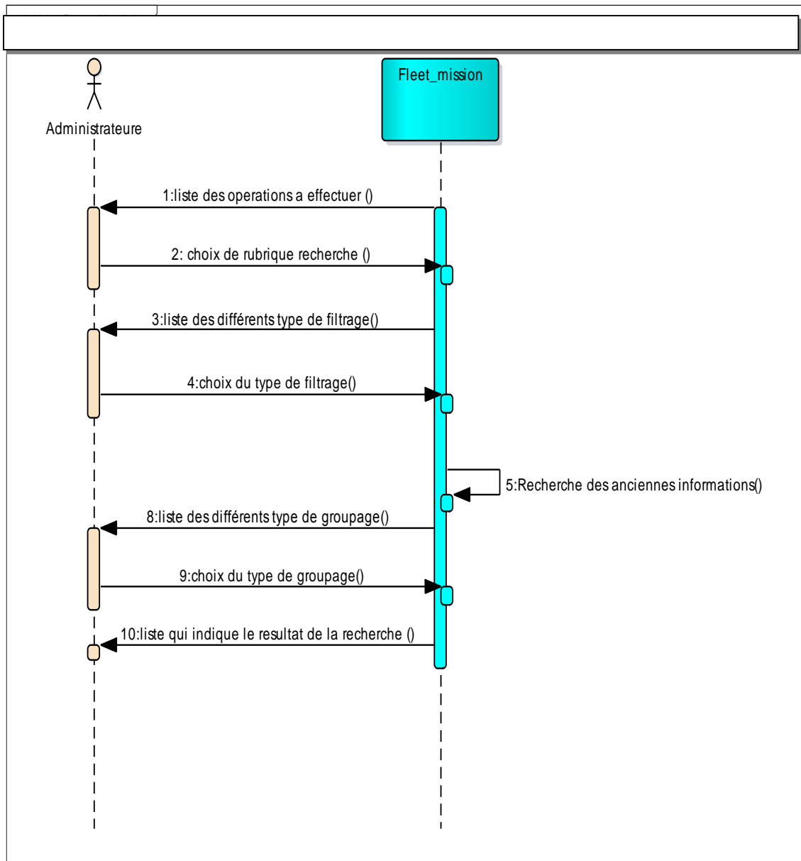
Figure II.4 : diagramme de séquence scénario de recherche d’une mission
