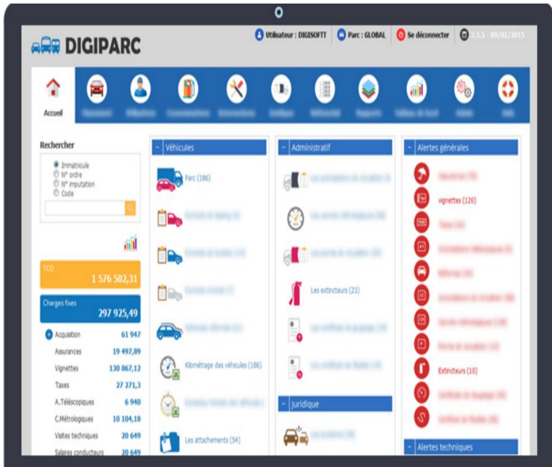
Figure I.6 : interface du module DIGIPARC [6]
