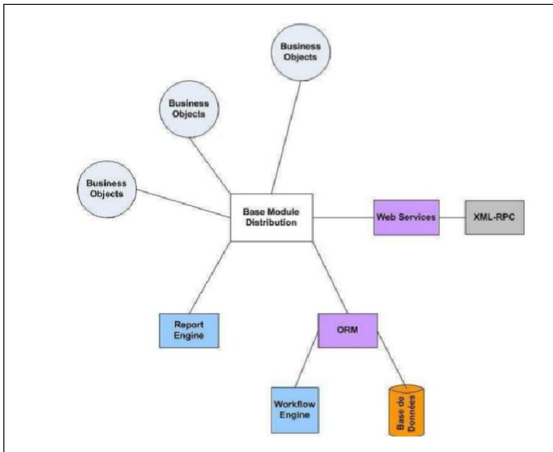
Figure I.2 : les composants d'un serveur ODOO [Open, 2012]
