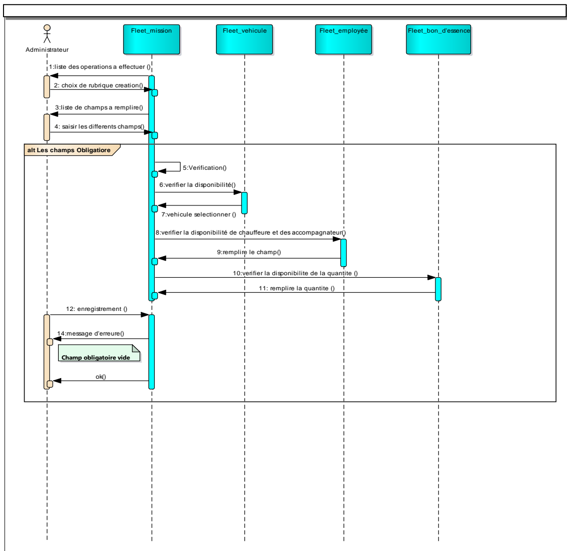
Figure II.2 : diagramme de séquence scénario de création d’une mission
