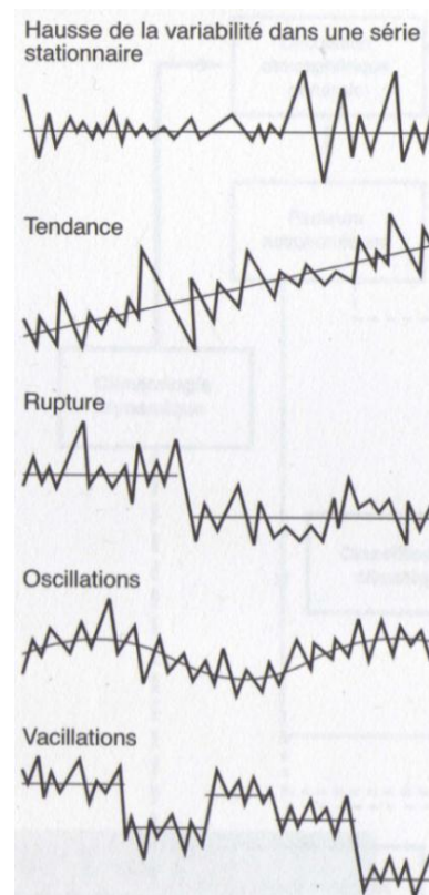
Figure 3. 1 – Variabilité climatique (HUFTY, 2001)
