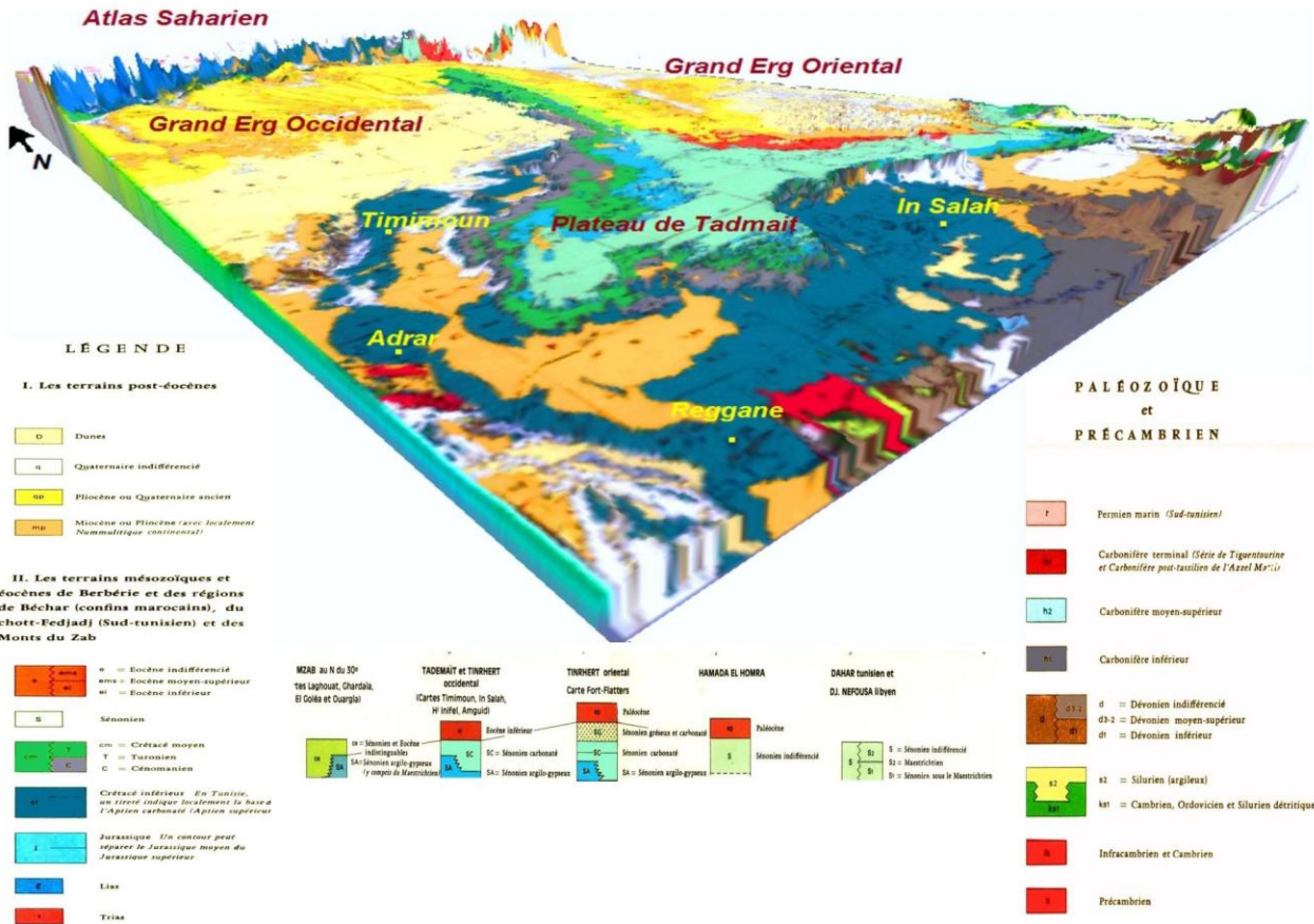
Figure n°5 : Carte géologique de la région d'étude ANRH d'Adrar (In: Benhamza, 2013).
