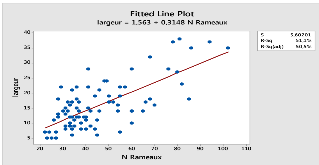
Figure n°21 : Les corrélations linéaires entre les paramètres mesurés de la station d'Adrar.
