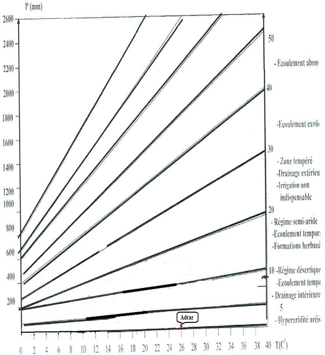
Figure n°4 : Indice d'aridité de DEMARTONNE
