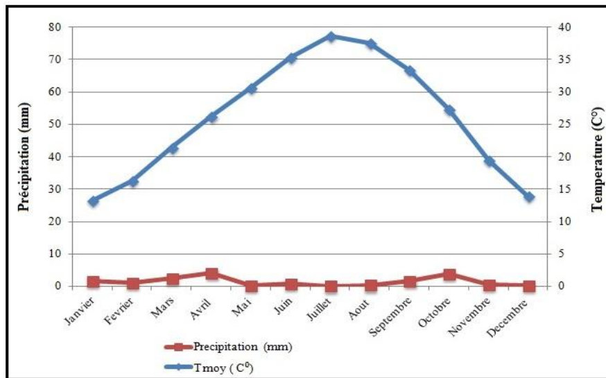
Figure n°2 : Diagramme Ombrothermique de Bagnouls et Gausson de la région d'Adrar (période : 2004 - 2014)
