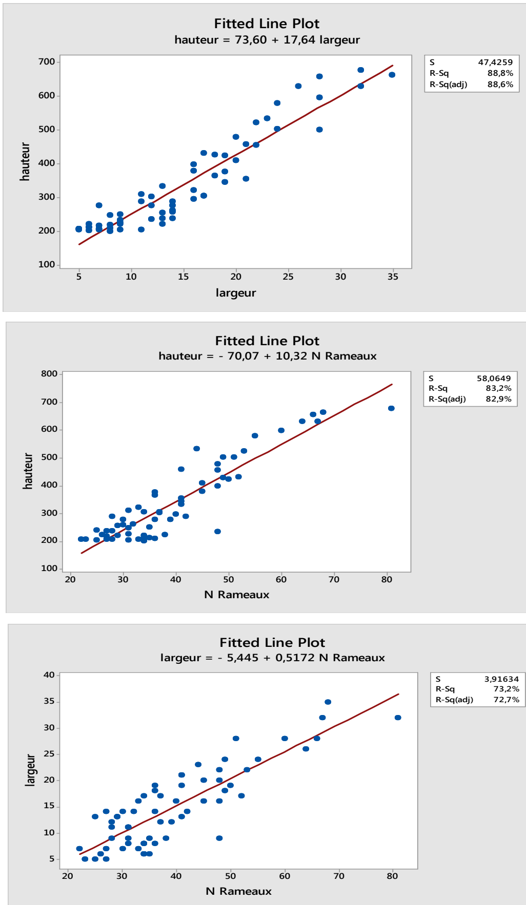
Figure n°20 : Les corrélations linéaires entre les paramètres mesurés de la station de Tamentit.
