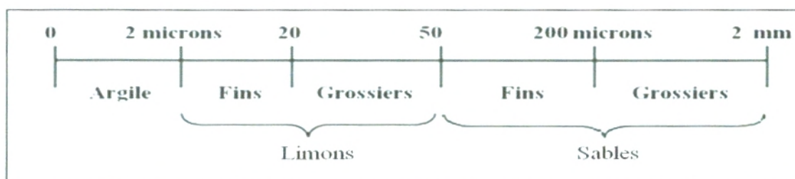
Figure N°14 : L'échelle internationale de la classification de sol
