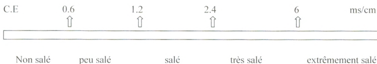
Fig. N°21 : Echelle de salure en fonction de la conductivité de l'extrait aqueux au 1/5 : relation de Richards in AUBERT G.1978
