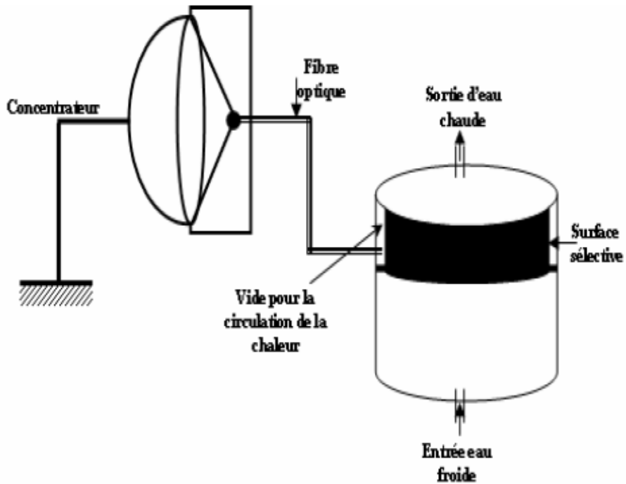
Figure III-1 : Système de production et de stockage d'eau chaude sanitaire
