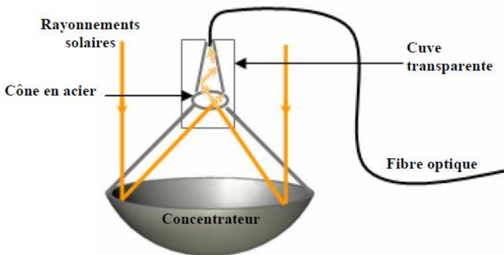
Figure III-2 : Schéma du concentrateur couplé avec une fibre optique
