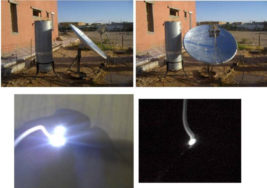
Figure III-3 : Photos du système réalisé opérationnel
