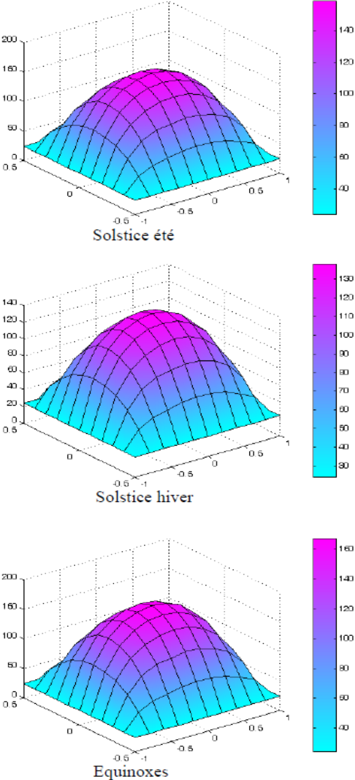
Figure III-6 : Températures atteints sur la surface sélective aux solstices
