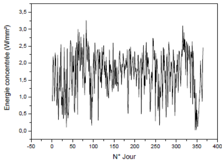
Figure III-5 : Variation journalière du rayonnement direct concentré à la sortie de la fibre optique
