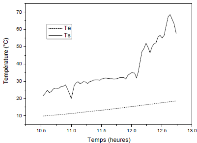
Figure III-7: Variation des températures d'entrée et sortie du système
