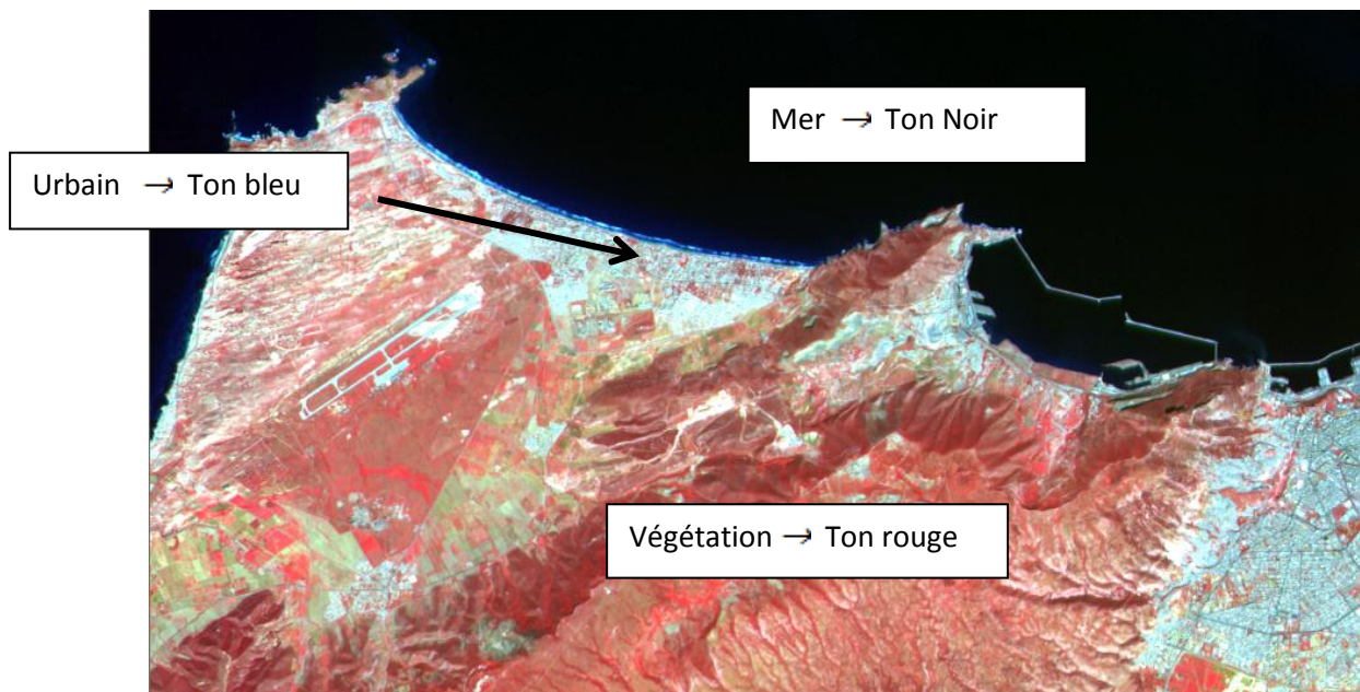
Figure I.7. :Image Spot de résolution 35m (Oran).
