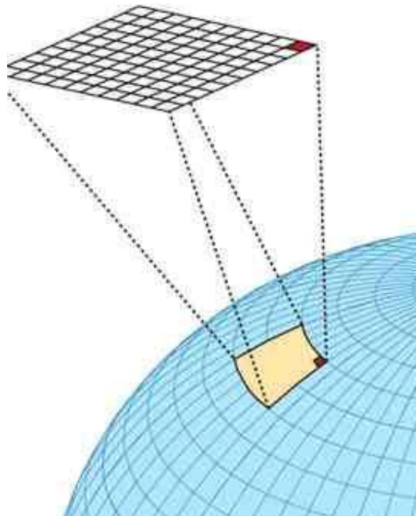
Figure I.6 : Résolution spatiale.[11]
