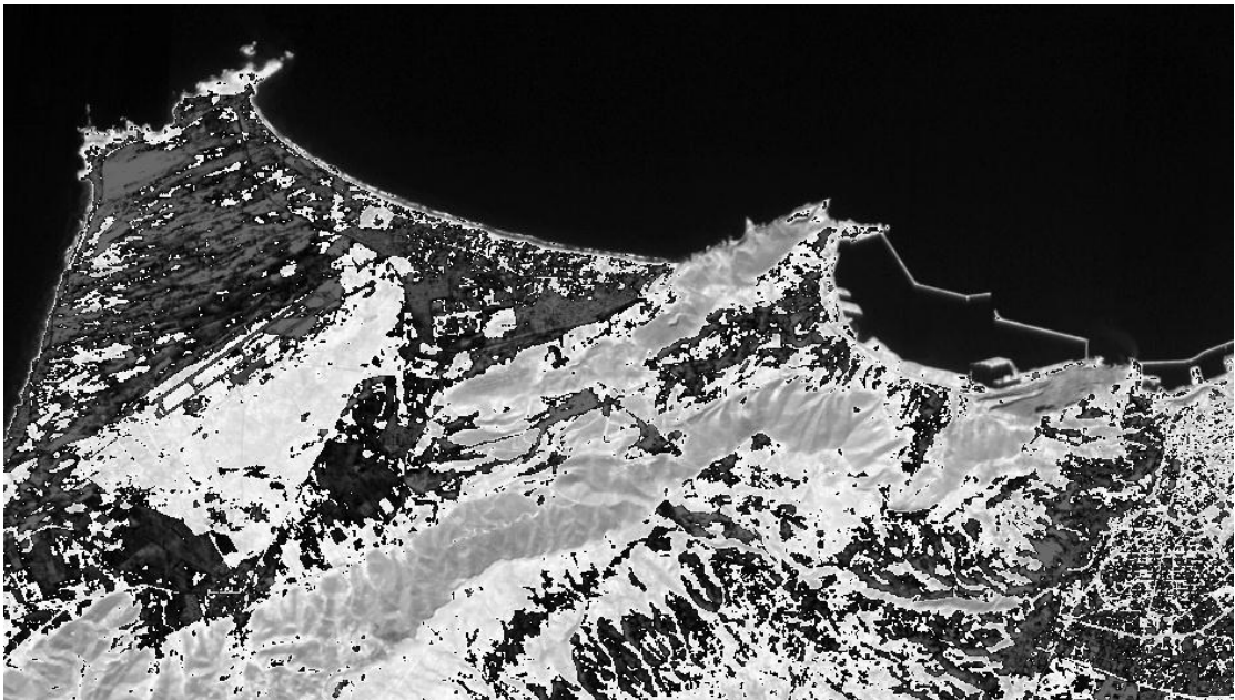
Figure III.16 : Indice de brillance (IB) (Image 2).
