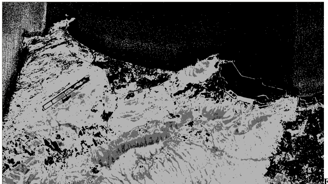
Figure III.18 :Indice de végétation par quotient(RVI) (Image 2).
