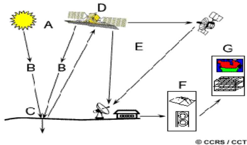
Figure I.4 : étapes de la télédétection.
