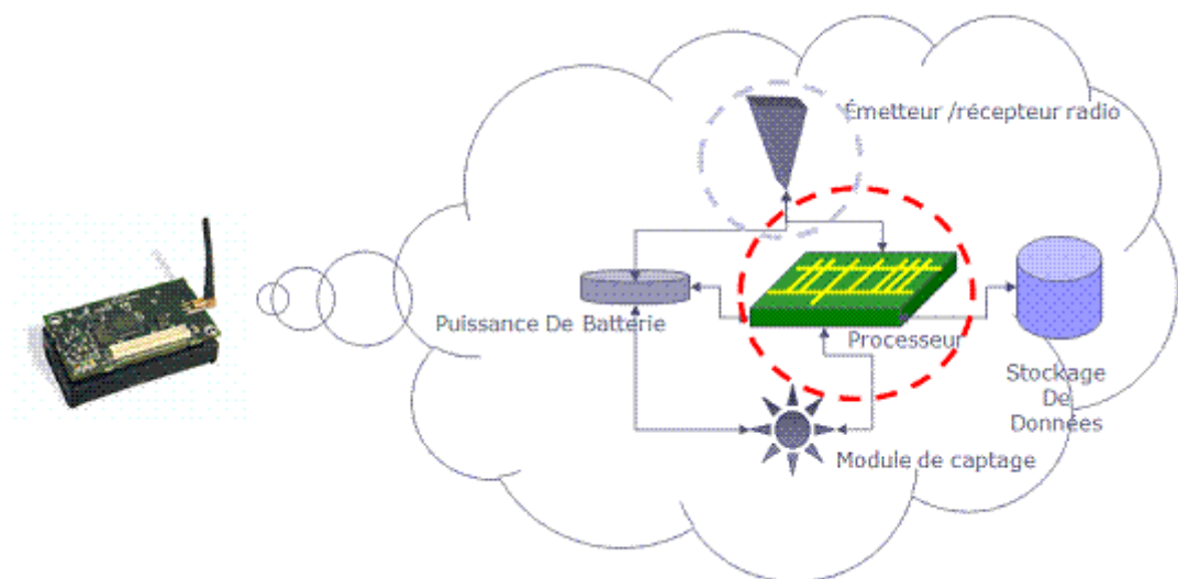
Figure 1. 1 : Anatomie d'un Nœud Capteur
