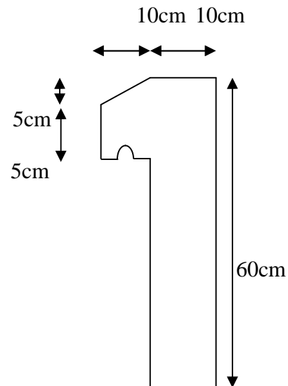
FIGURE 3.7: DIMENSIONS DE L'ACROTÈRE
