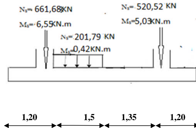
Figure 6.2 : chargement de la semelle filant a L' ELU
