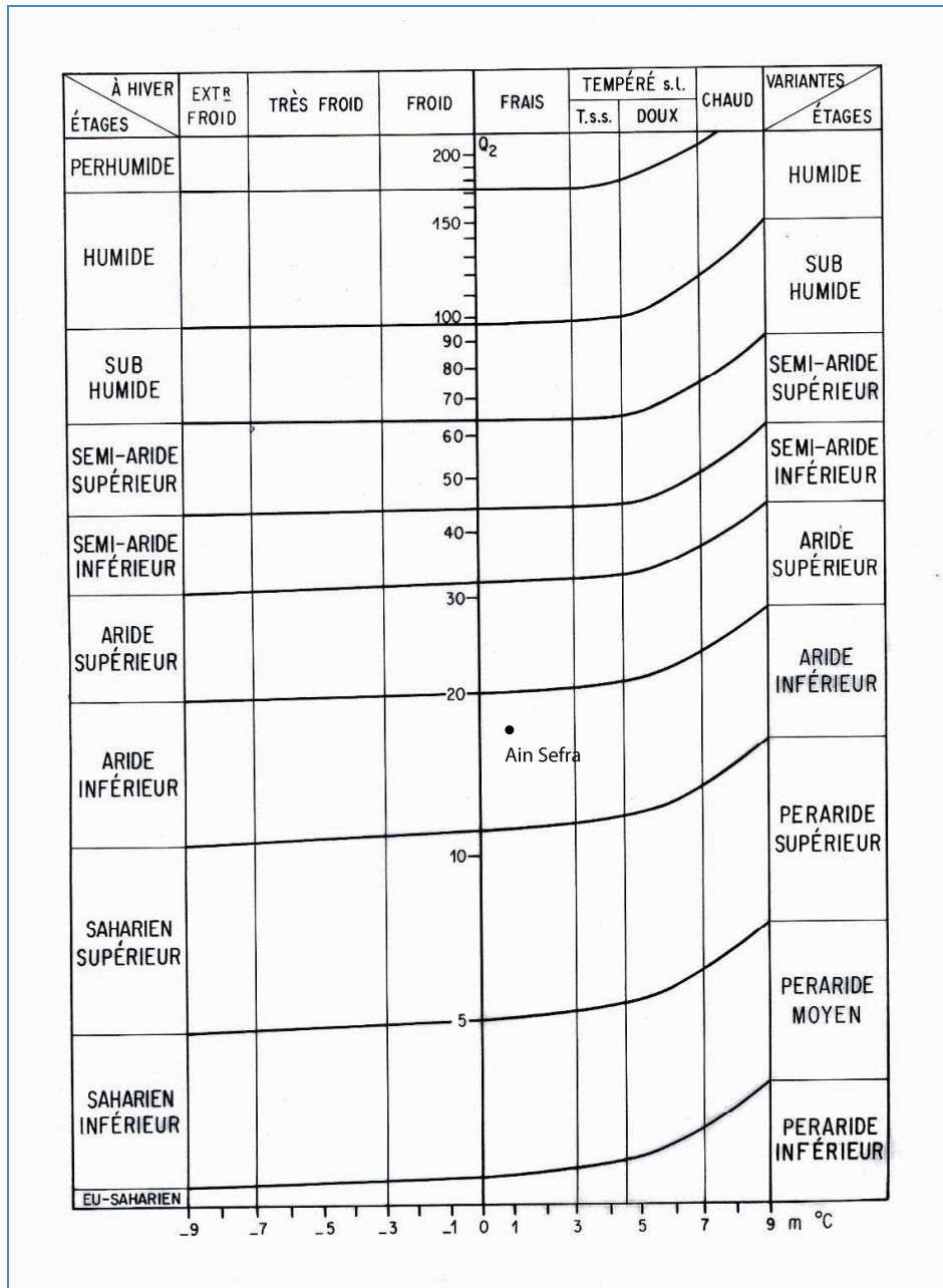
Fig 06: Climagramme du quotient pluviométrique d'Emberger
