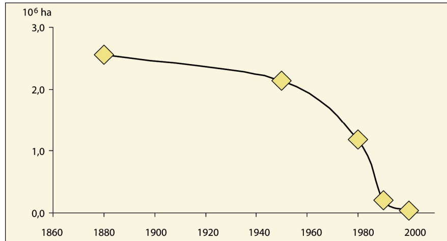
Fig.13 : Évolution estimée des steppes d'alfa (en millions d'hectares) dans les Hautes Plaines (versants exclus) du Sud oranais (Algérie). (AIDOUD A. et al., 2006)
