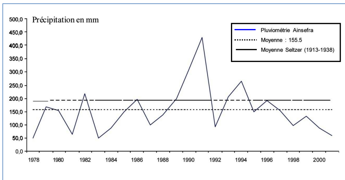
Figure 5 : Précipitations moyennes annuelles à la station d'Aïn sefra (1978-2001).
