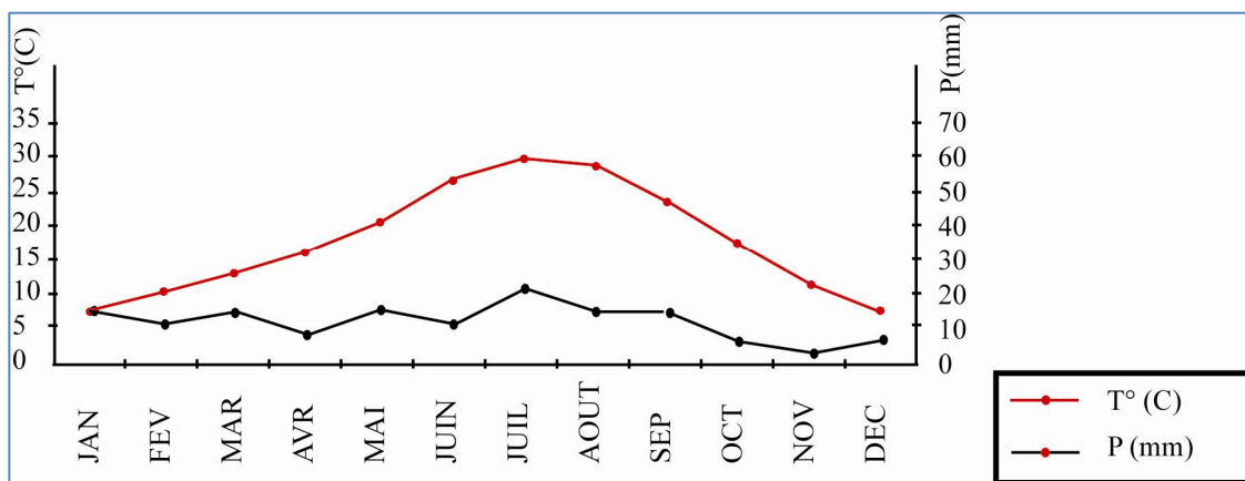
Fig 07: Diagramme ombrothermique de Bagnouls & Gausсен
