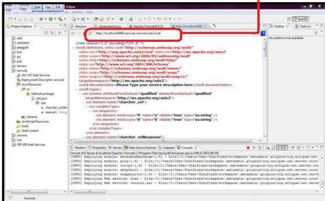
Figure IV.1 : Fichier WSDL
