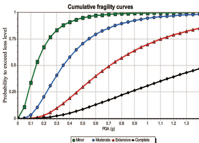
Figure 1. Courbe de vulnérabilité d'un réservoir
