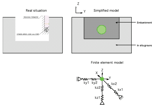
Figure 3. Model du macroélément (ressorts concentrés)
