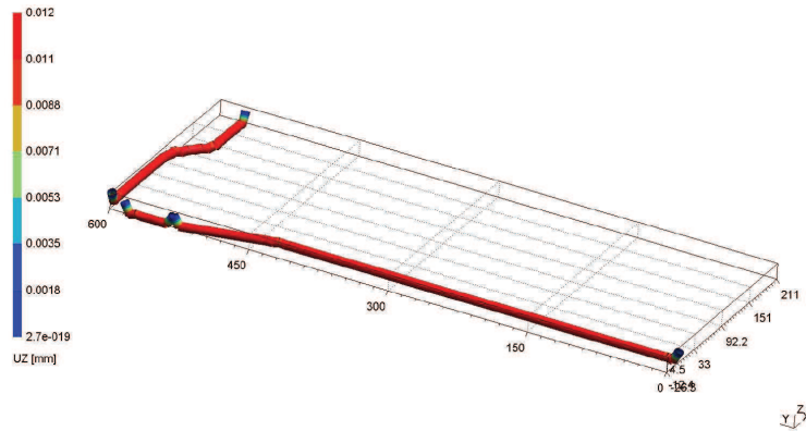
Figure 4. Déplacement relatif sol structure (direction verticale)
