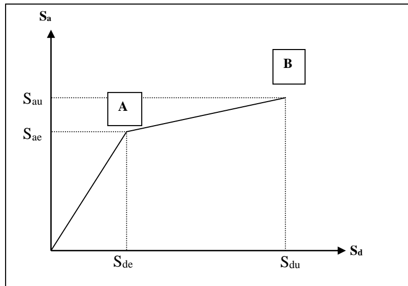
Figure II-3 Forme simplifiée de la courbe de capacité
