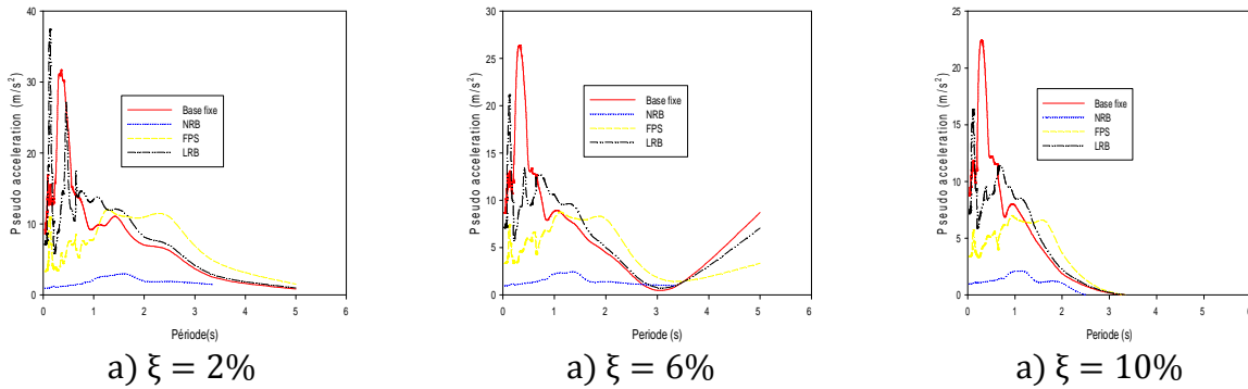
Figure IV.59 : Spectres de réponse en pseudo-accelération à la base d'une structure à base fixe et isolée par des isolateurs de types (LRB, FPS, NRB), sous un chargement de Sylmar.
