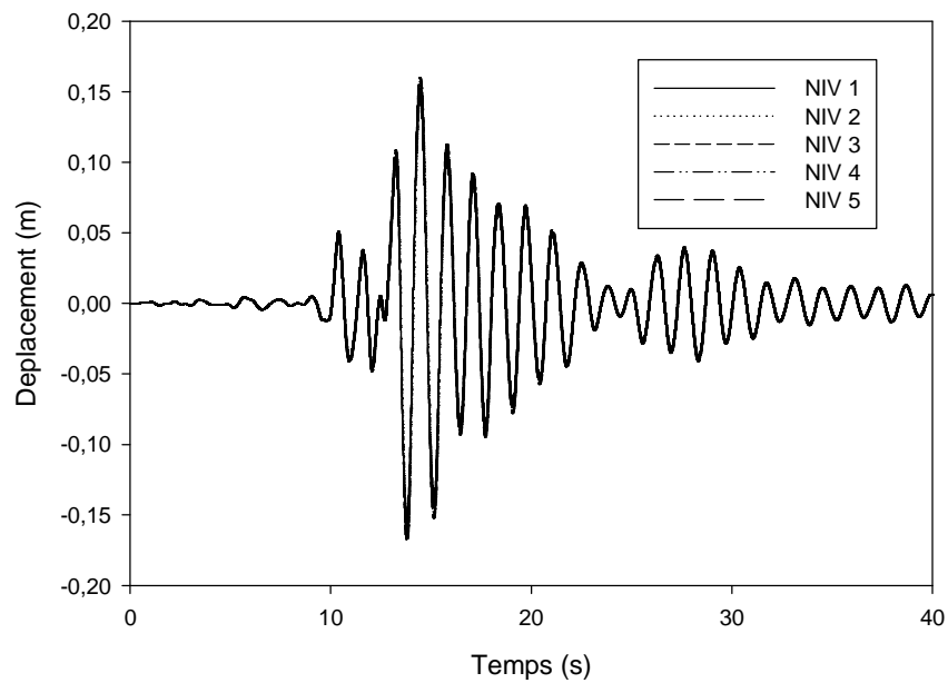
Figure IV.29: Déplacement des différents niveaux d'une structure isolée par des appuis de type NRB pour le séisme de Loma Prieta.
