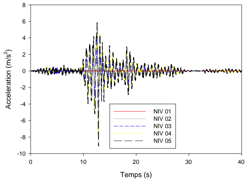
Figure IV.12: Accélération des différents niveaux d'une structure encastrée pour le séisme de Loma Prieta.
