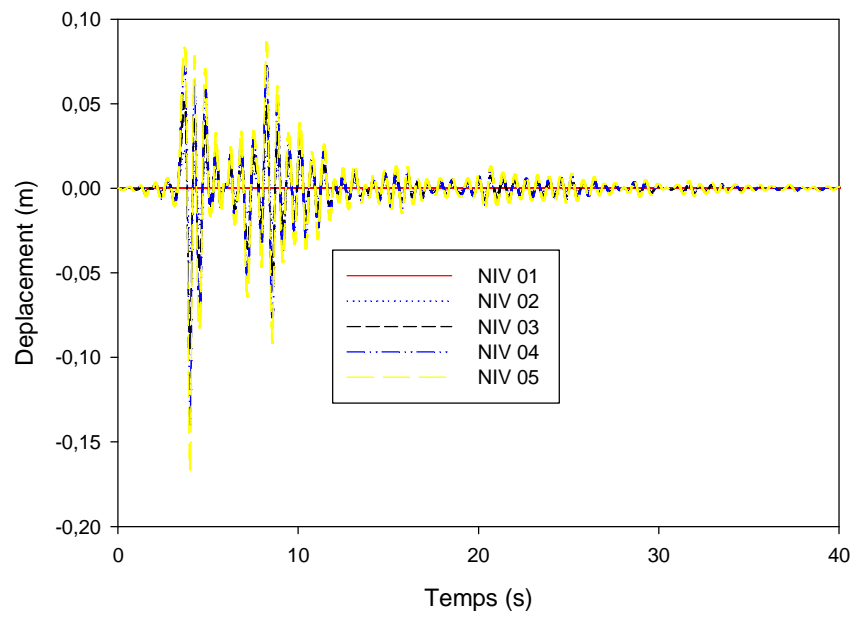
Figure IV.17: Déplacement des différents niveaux d'une structure encastrée pour le séisme de Sylmar.
