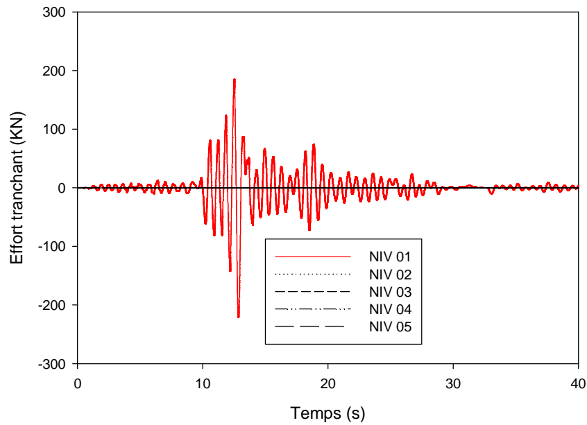
Figure IV.14: Effort tranchant des différents niveaux d'une structure encadrée pour le séisme de Loma Prieta.
