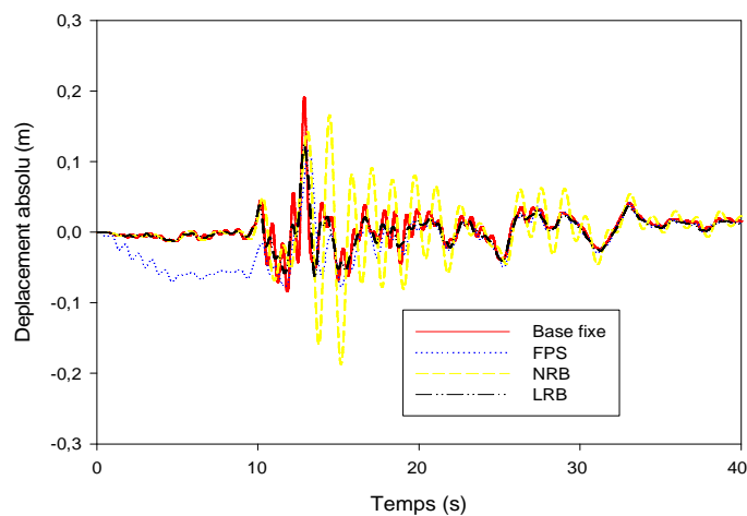
Figure IV.51: Déplacement absolu du dernier niveau pour les différents types d'isolateurs sous le séisme de Loma Prieta.
