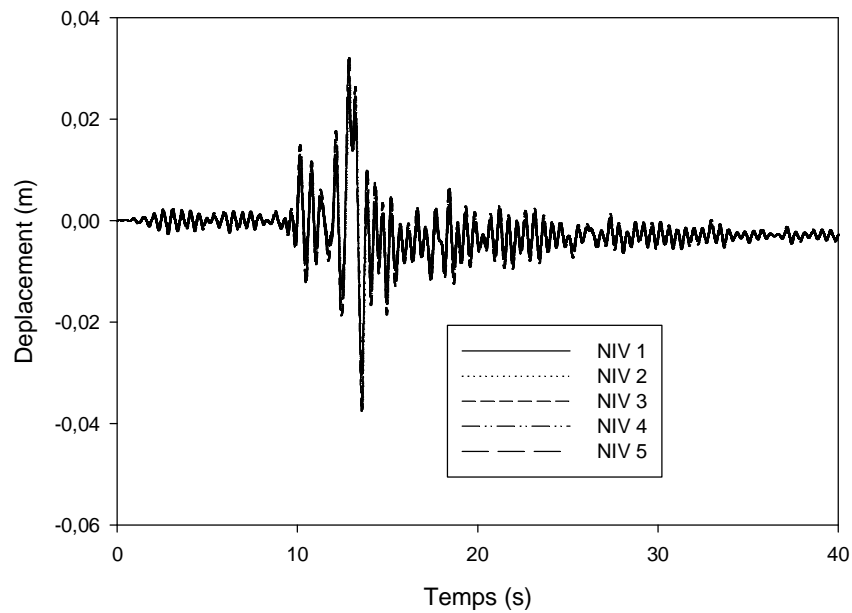
Figure IV.37: Déplacement des différents niveaux d'une structure isolée par des appuis de type LRB pour le séisme de Loma Prieta.
