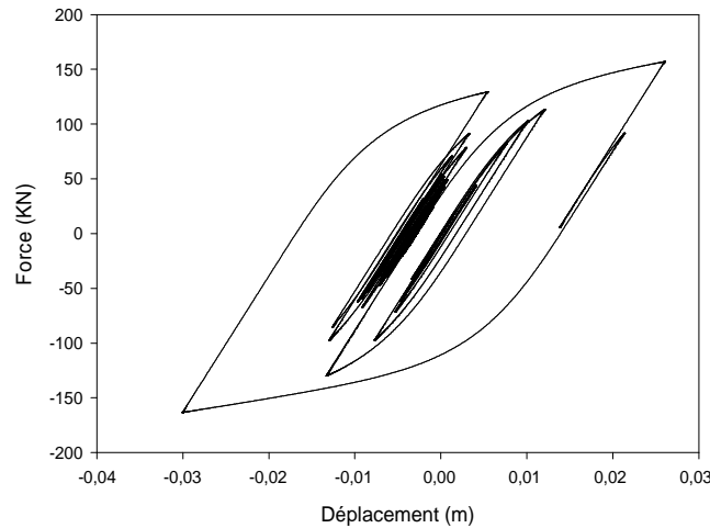
Figure IV.7:Loi de comportement des appuis de type (LRB).
