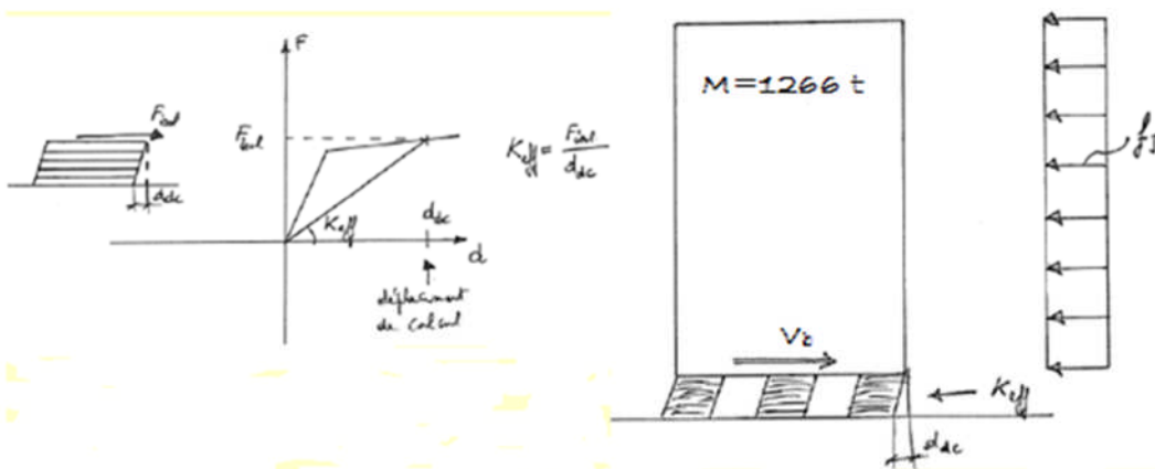
Figure III.7 : Exemple d'un bâtiment isolé à la base.
