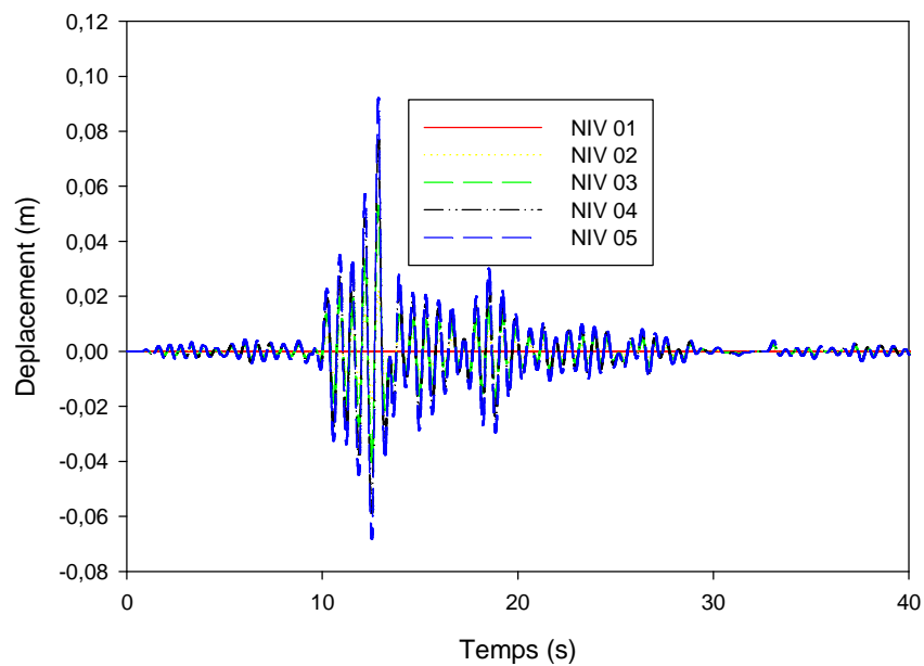
Figure IV.13: Déplacement des différents niveaux d'une structure encastrée pour le séisme de Loma Prieta.
