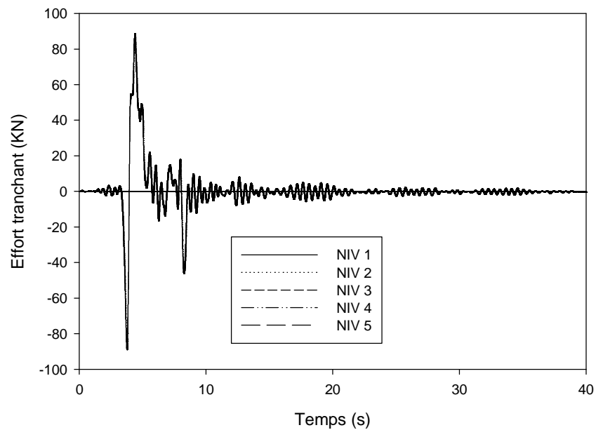
Figure IV.42: Effort tranchant des différents niveaux d'une structure isolée par des appuis de type LRB pour le séisme de Sylmar.
