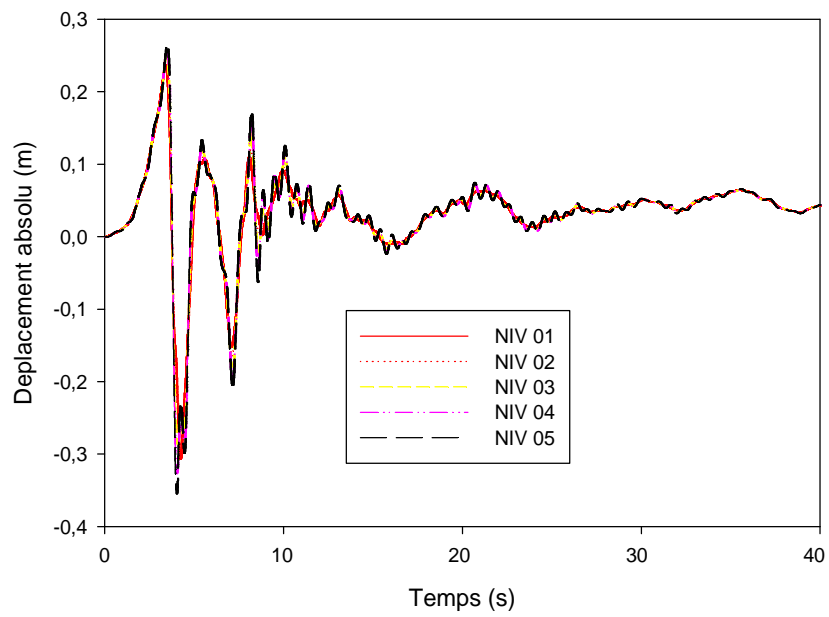
Figure IV.15: Déplacement absolu des différents niveaux d'une structure encastrée pour le séisme de Sylmar.
