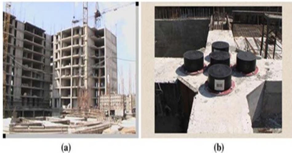
Figure I.16: Bâtiment isolé à la base à Yerevan (Arménie)
