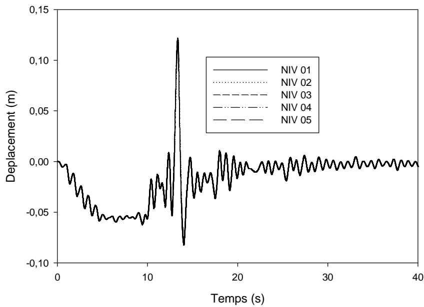
Figure IV.21: Déplacement des différents niveaux d'une structure isolée par des appuis de type FPS pour le séisme de Loma Prieta.
