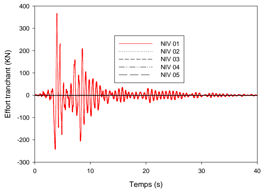
Figure IV.18: Effort tranchant des différents niveaux d'une structure encastrée pour le séisme de Sylmar
