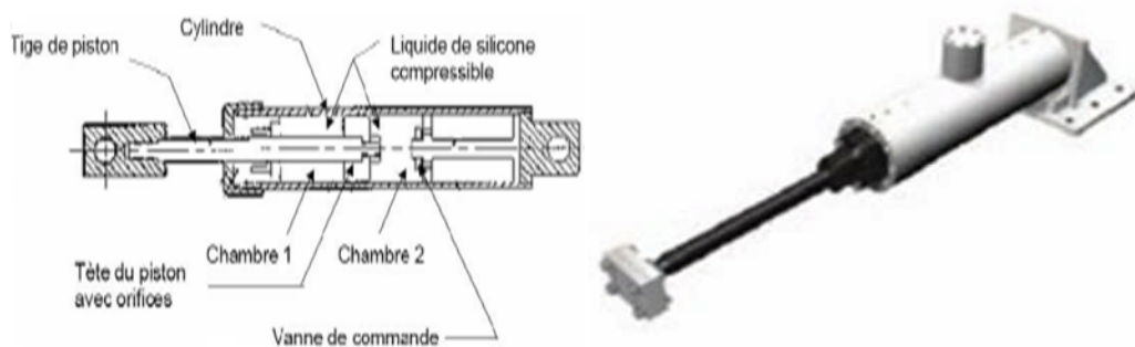
Figure II.2: Amortisseur visqueux.
