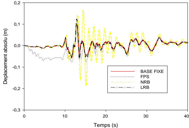
Figure IV.43: Déplacements absolu du premier niveau pour les différents types d'isolateurs sous le séisme de Loma Prieta.
