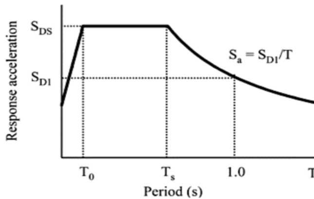
Figure III.3: Spectre de réponse selon l'IBC2003.
