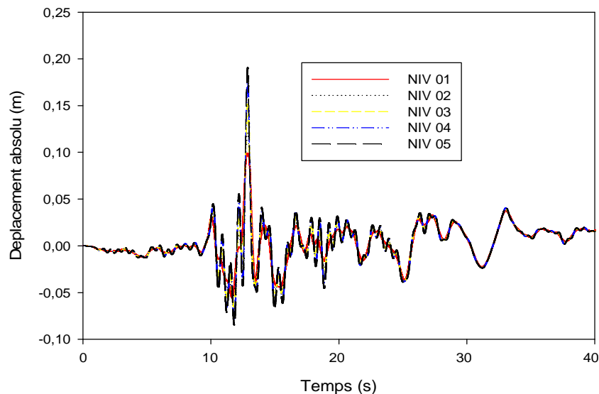
Figure IV.11: Déplacement absolu des différents niveaux d'une structure encadrée pour le séisme de Loma Prieta.
