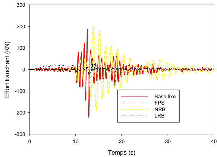
Figure IV.46: Effort tranchant du premier niveau pour les différents types d'isolateurs sous le séisme de Loma Prieta.
