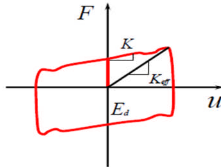
Figure II.8:Loi de comportement des appuis de type (FPS)
