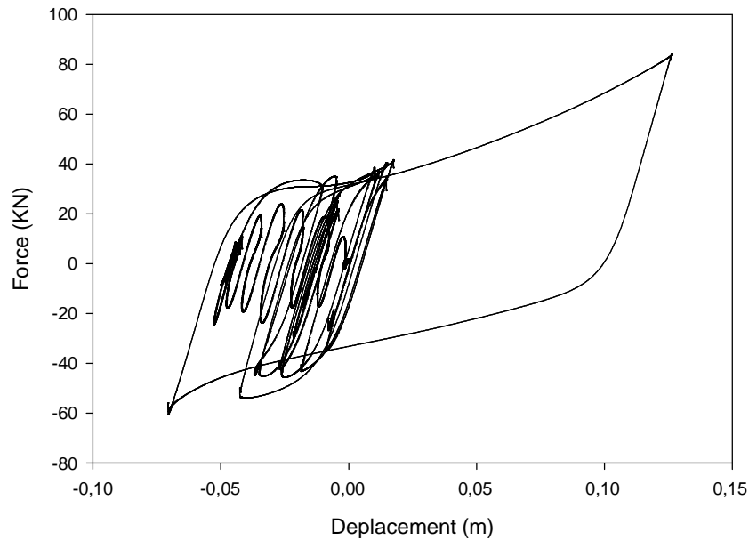
Figure IV.8: Loi de comportement des appuis de type (FPS).
