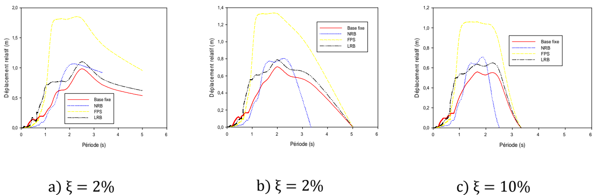
Figure IV.60 : Spectres de réponse en déplacement relatif à la base d'une structure à base fixe et isolée par des isolateurs de types (LRB, FPS, NRB), sous un chargement de Sylmar.
