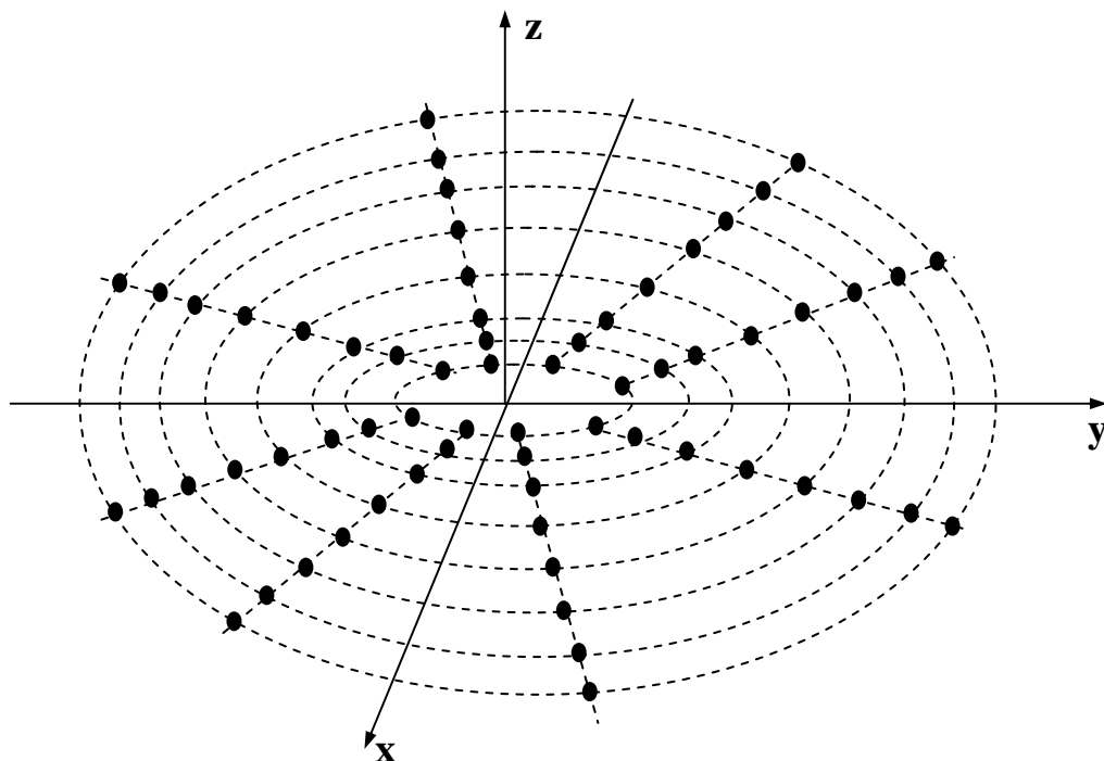
Figure V.13 : Réseau circulaire
