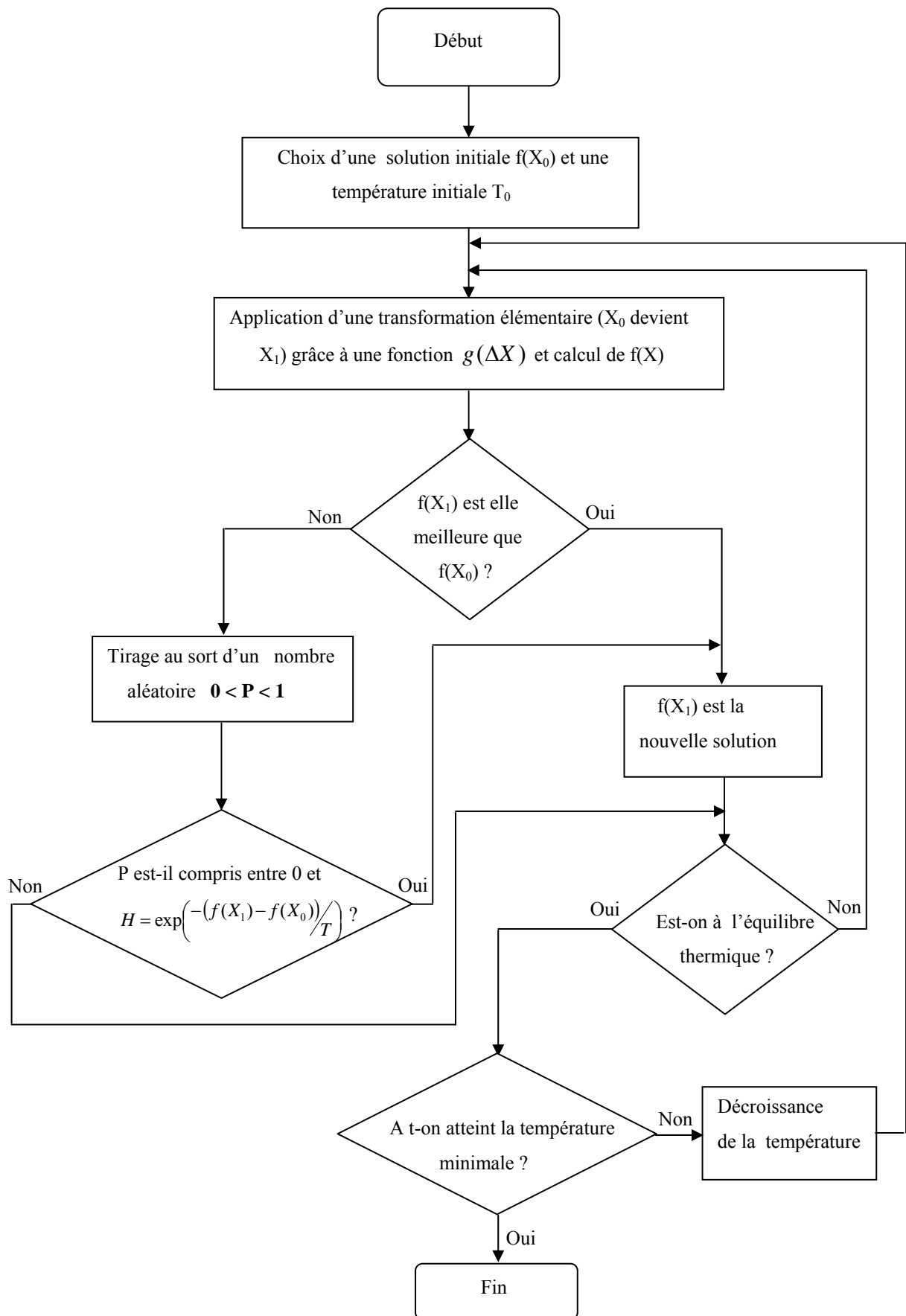
Figure IV.3 : Algorithmme du recuit simulé
