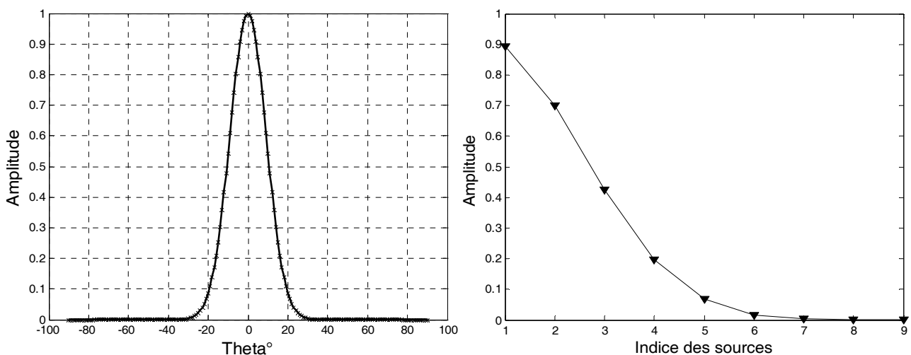
(a) : Diagrammes de rayonnement
