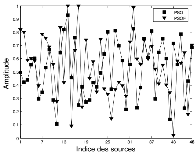
(d) : Amplitude optimisées par PSO et PSOF
