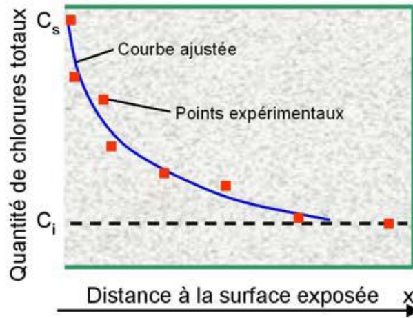
Figure I.11 Profil en chlorures dans le béton après immersion [DEB, 2008]
