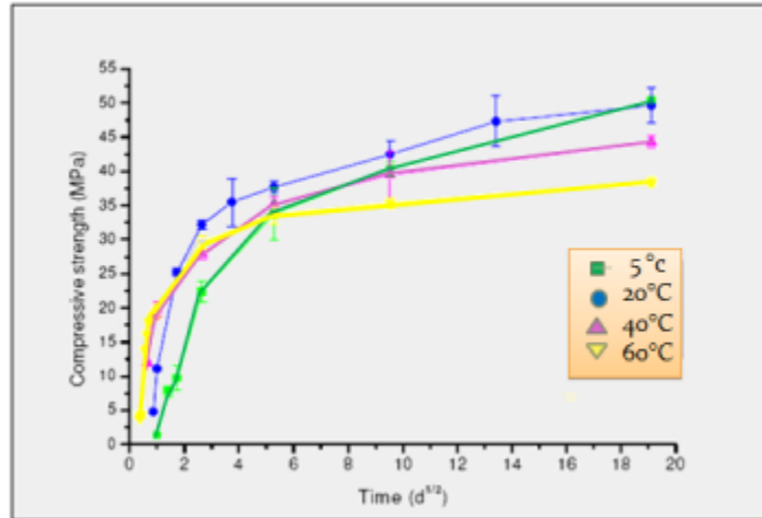
Figure I.18. Développement de résistance des bétons en fonction de la température [GAL, 06]
