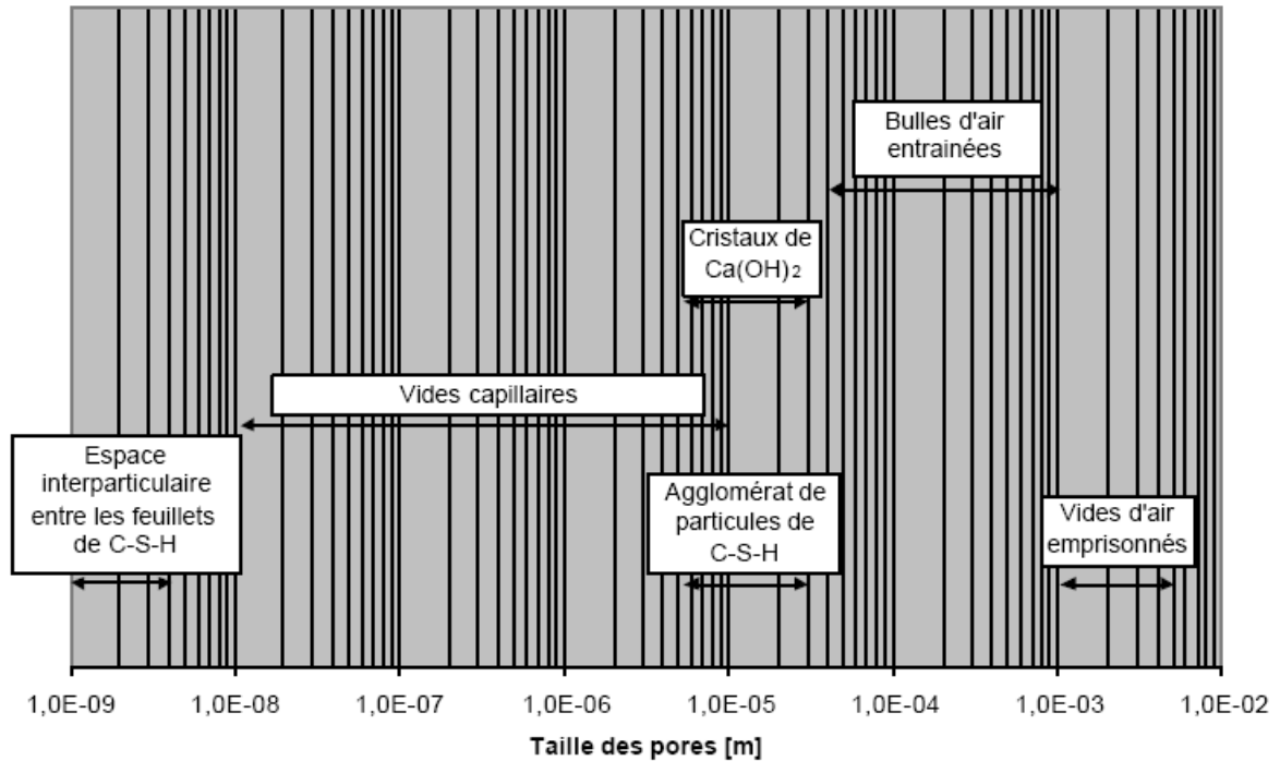
Figure I.3 Dimension des pores et solides dans la pâte de ciment hydraté [MEH, 91 cité par NUG, 02].
