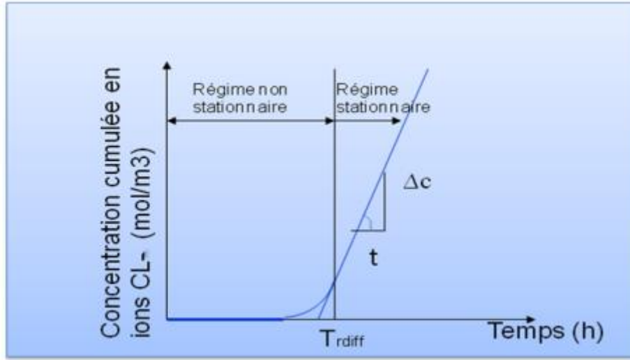
Figure I.9. Evolution de la concentration cumulée en ions chlores dans le compartiment aval en fonction du temps [NUG, 02]
