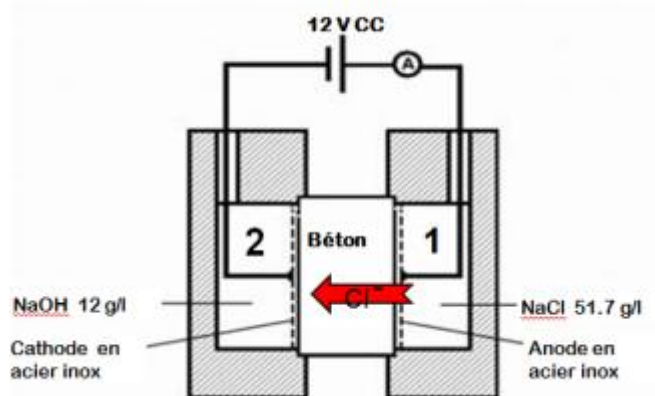
Figure II.23 Schéma de principe d'une cellule de migration selon NT BUILD 355 [BUI, 97]
