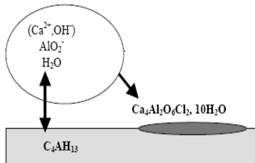
Figure I.15 Mécanisme de formation du monochloro-aluminate [HYV, 09].
