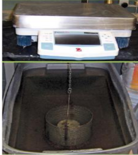
Photo II.1 Principe de la pesée hydrostatique
