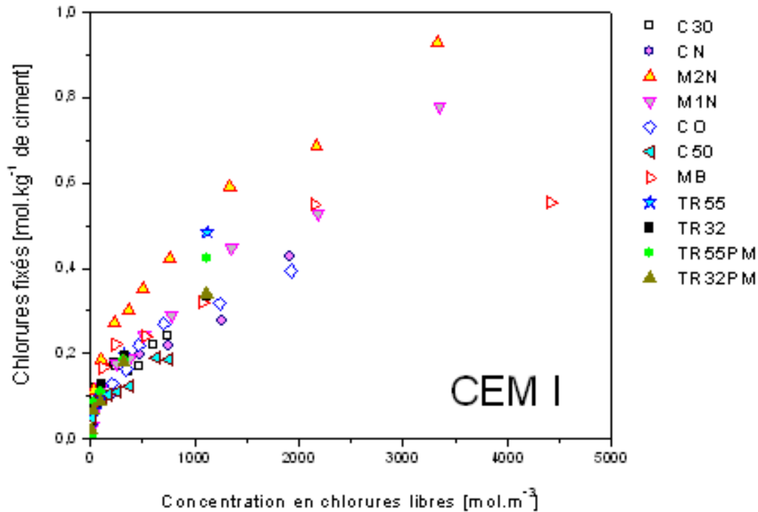
Figure I.14: Synthèse des isothermes d'interaction obtenues sur différents matériaux à base de ciment CEM I (pâtes de ciment : C30, C50 et CN, CO [mortiers M1N, M2N, MB ; bétons TR55, TR32, TR55PM, TR32PM) [QNGU, 07].
