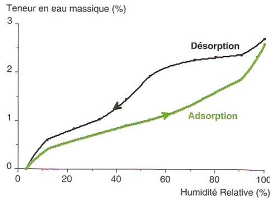
Figure II.7 Isotherme de désorption et d'adsorption de la vapeur d'eau d'un béton à hautes performances (à T= 23 \pm 0,1^{\circ} C ) [LCPC, 02]
