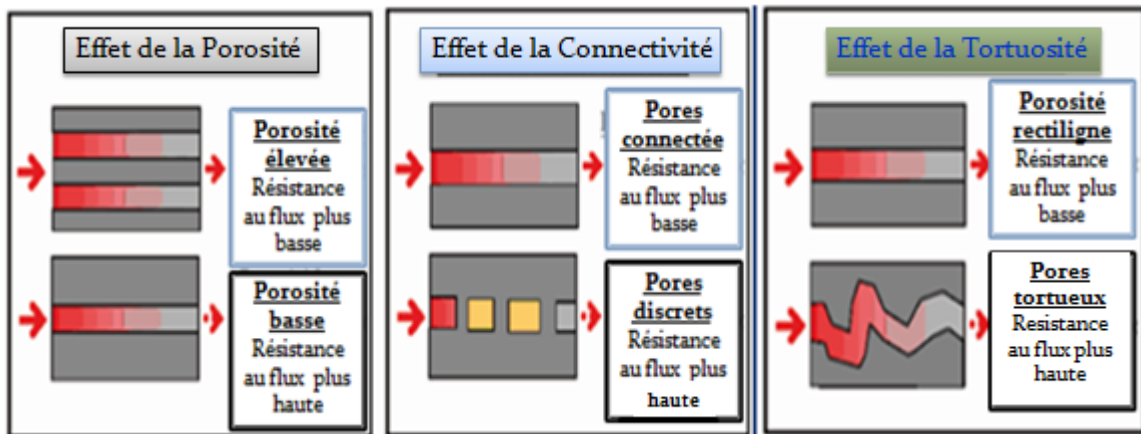
Figure I.5 Effet des paramètres influençant la perméabilité (d'après SCRIVENER, 2001 cité par CHO, 06 ).
