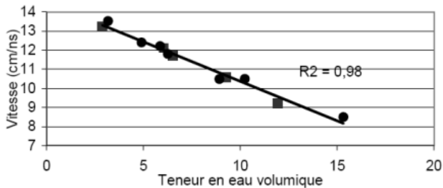
Figure II.34 Variation de la vitesse de l'onde directe en fonction de la teneur en eau volumique [BAL, 07].
