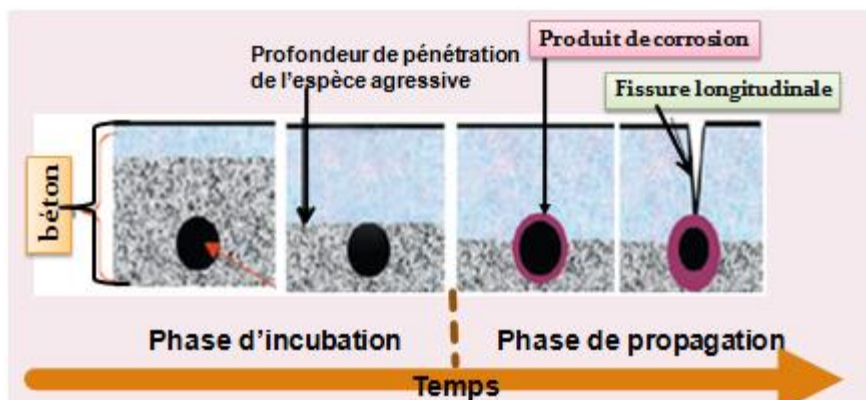
Figure 1. Corrosion des armatures du béton armé. Schématisation de l'évolution des dégradations du béton et de l'acier [BAR, 05]
