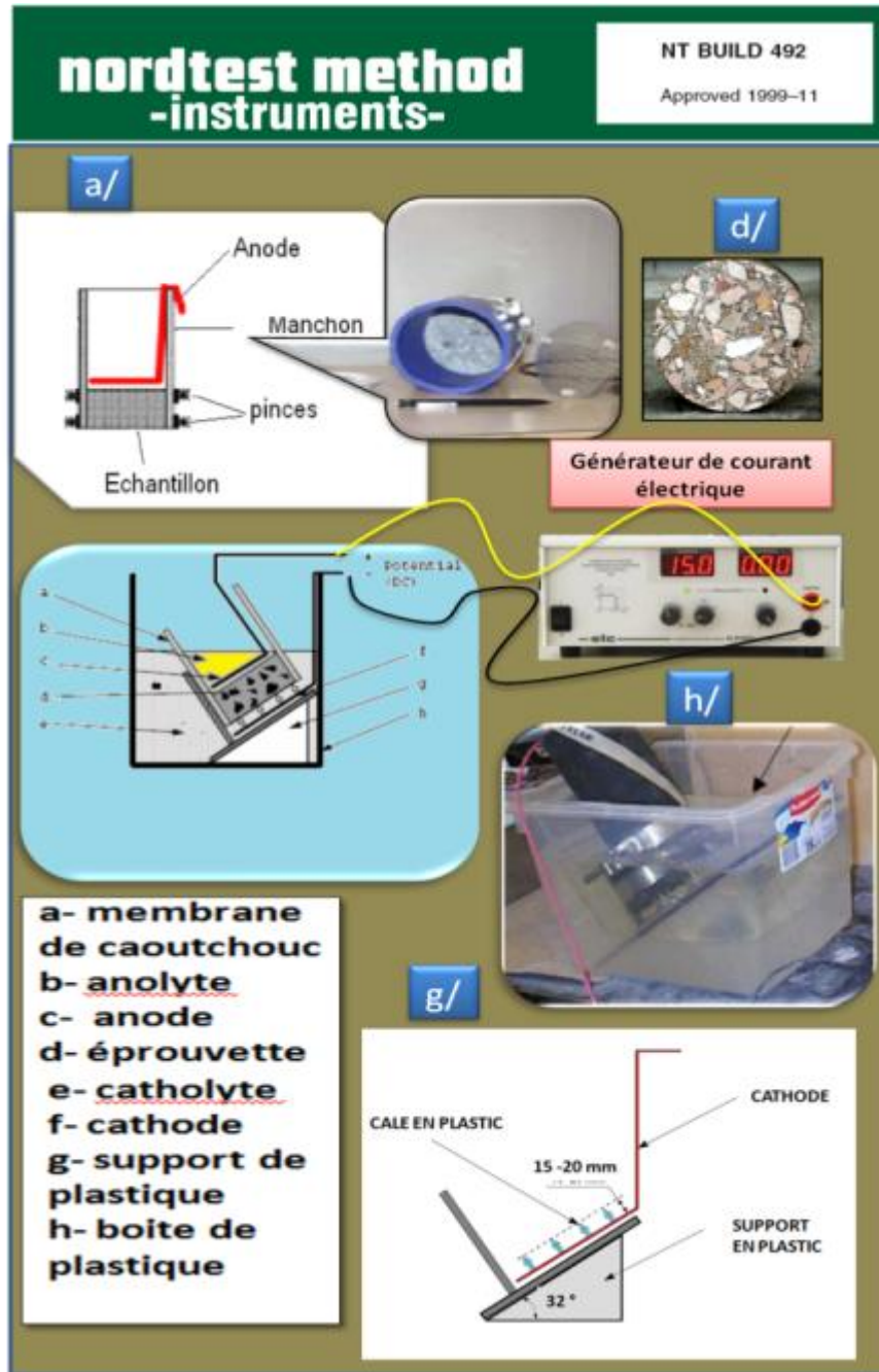
Figure II.26 Matériel utilisé pour l'essai de migration selon la norme NT BUILD 492 [BUI, 99]
