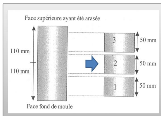
Figure II.1 Extraction des disques d'une éprouvette
