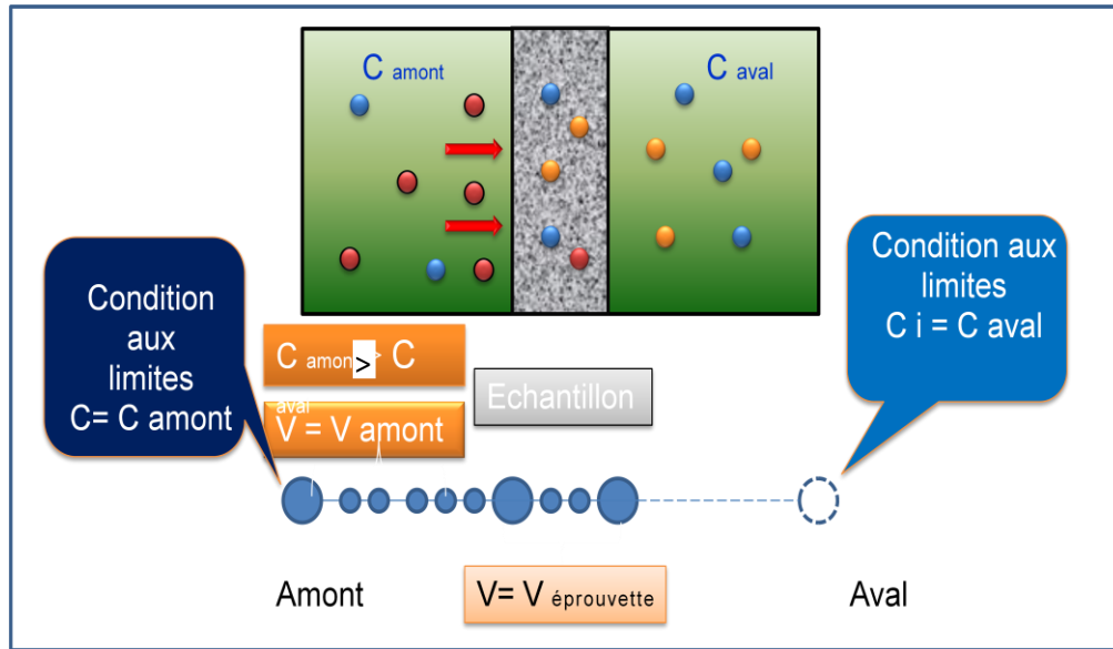
Figure II.9 Principe des essais de diffusion des ions [QNGU, 07]
