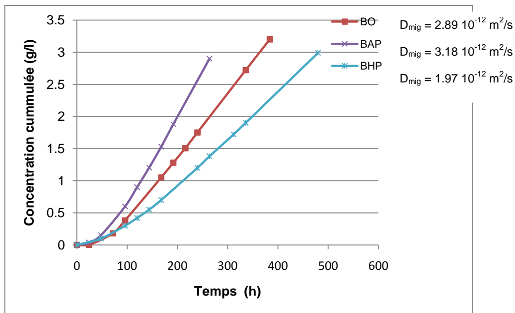
Figure II.21 Evolution de la concentration des ions chlorures en fonction du temps dans le compartiment aval en fonction de la nature du béton sur la diffusion [TOU, 09].
