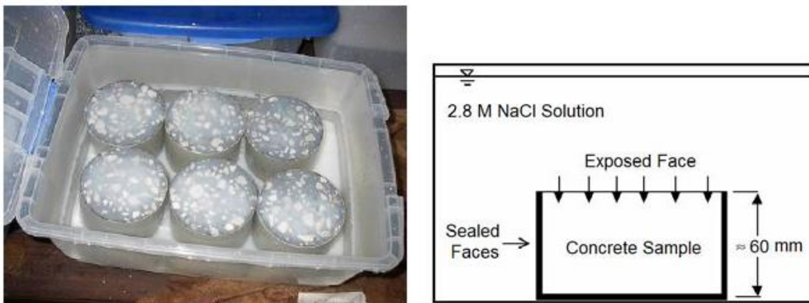
Figure II.14 Essai d'immersion d'éprouvettes de béton selon NT Build 443 [VIR, 07]
