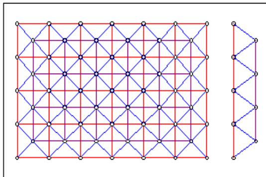
Figure 20: Plan de couverture en forme plane
