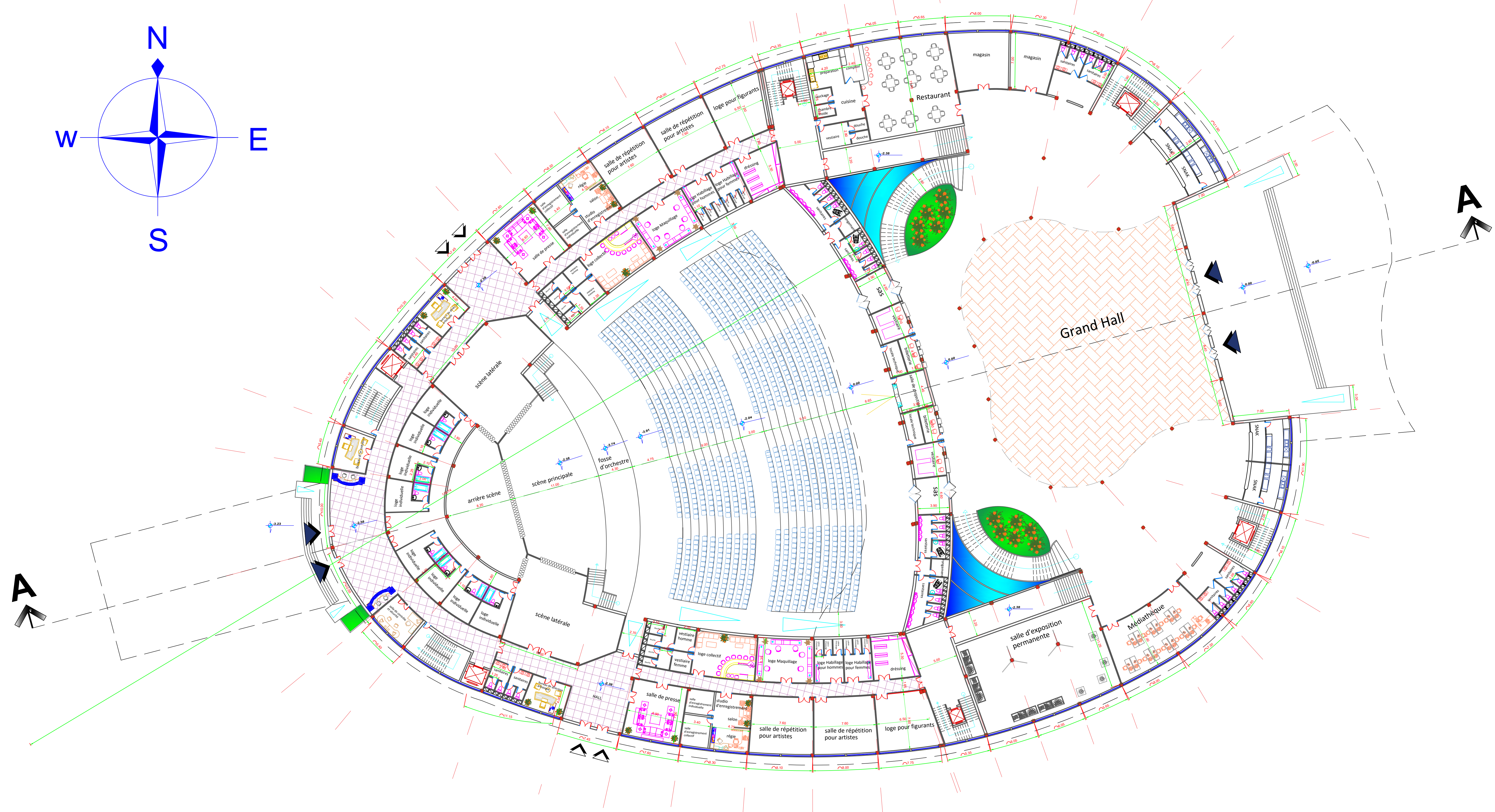
PLAN R.D.C ECH: 1/200
