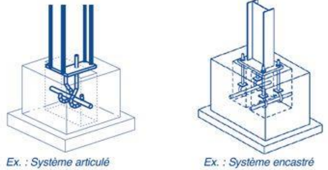
Figure 121: Exemple de poteau métallique avec fondation en béton armé.
