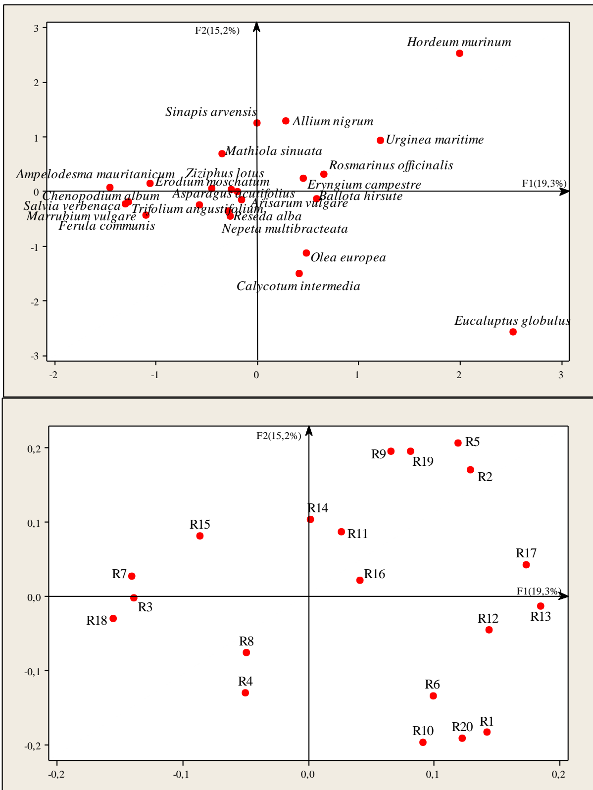
Figure 17 : Plan factoriel (F1x F2) de la répartition des espèces végétales de la station I selon les relevés.
