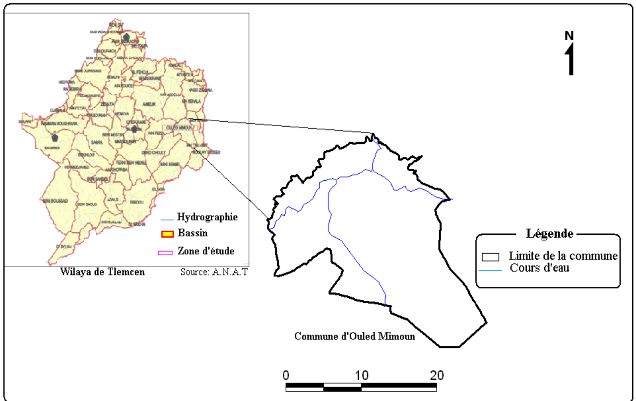
Figure 08 : Situation hydrographique de la wilaya de Tlemcen et la commune d'Ouled Mimoun
