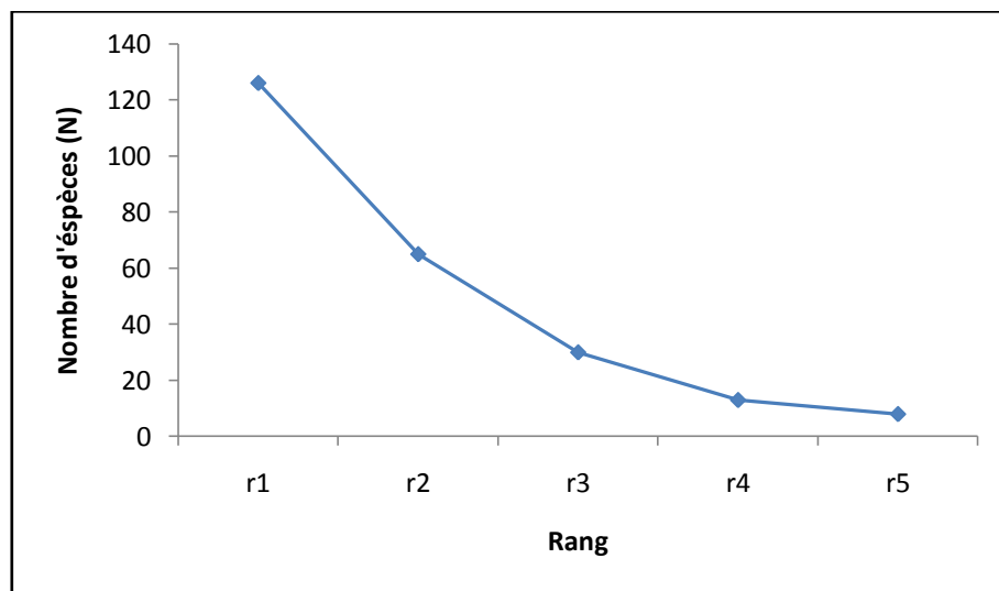
Figure 22 : Représentation graphique du modèle de Mac Arthur des espèces de la Station I.
