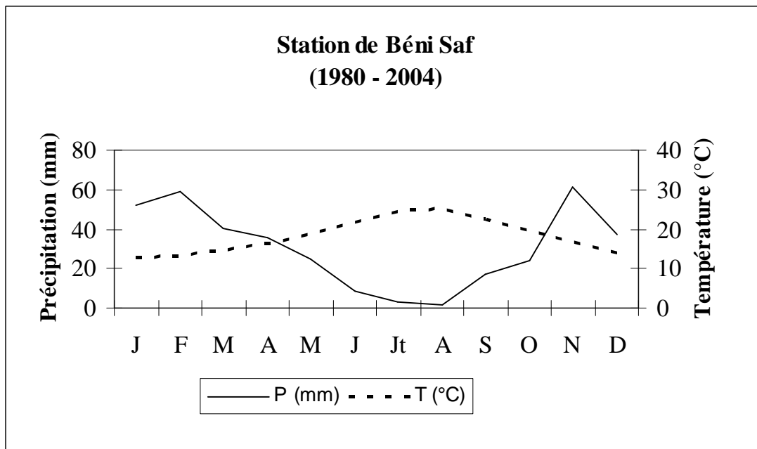
Figure 19 : Diagramme ombrothermique de Bagnouls et Gausсен
