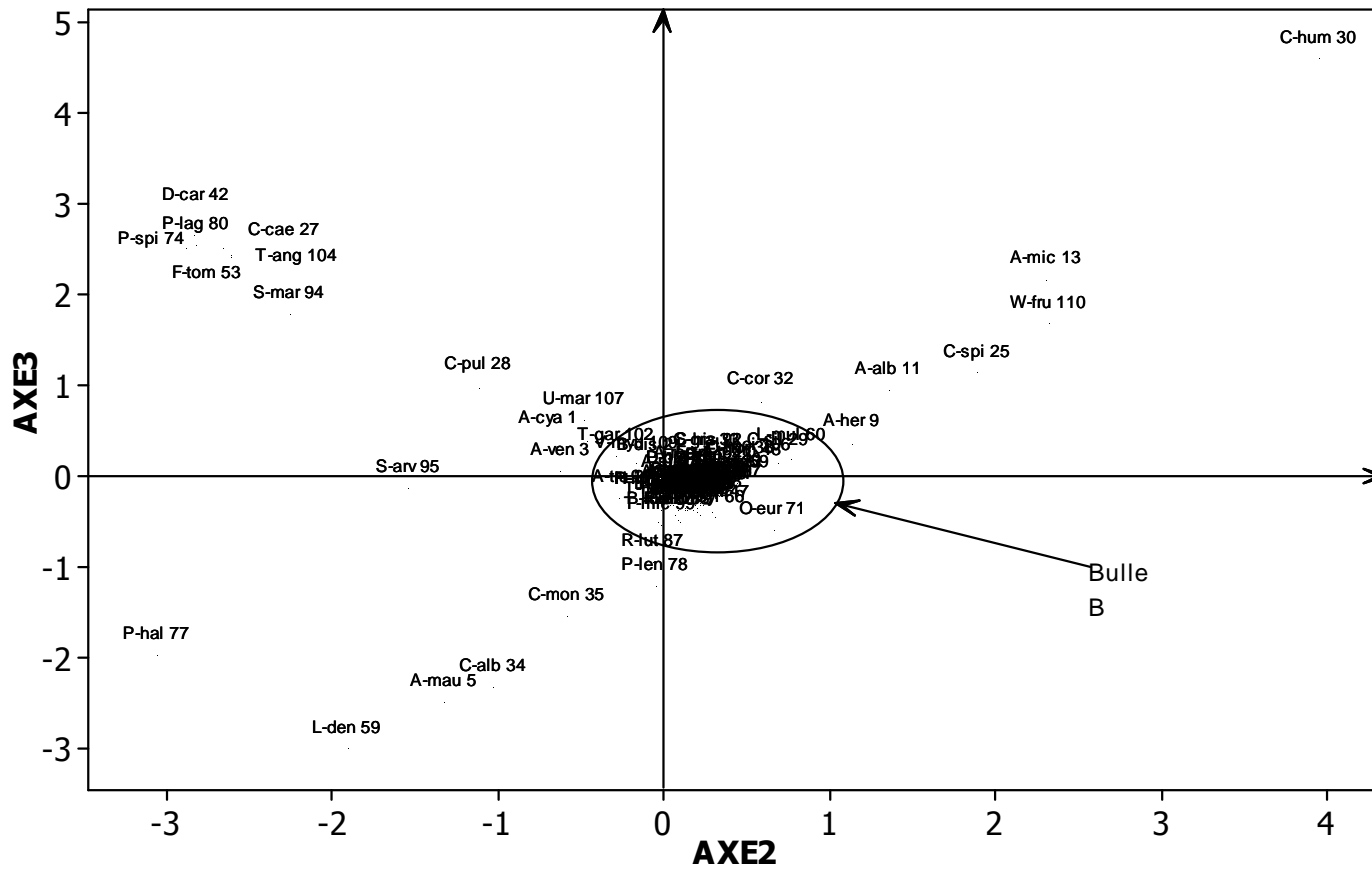
Figure 30 : Plan factoriel des espèces (axe 3 – axe 2)
