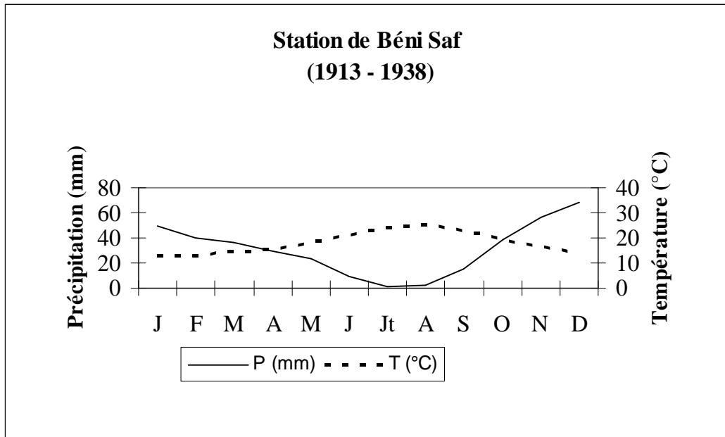
Figure 18 : Diagramme ombrothermique de Bagnouls et Gausсен
