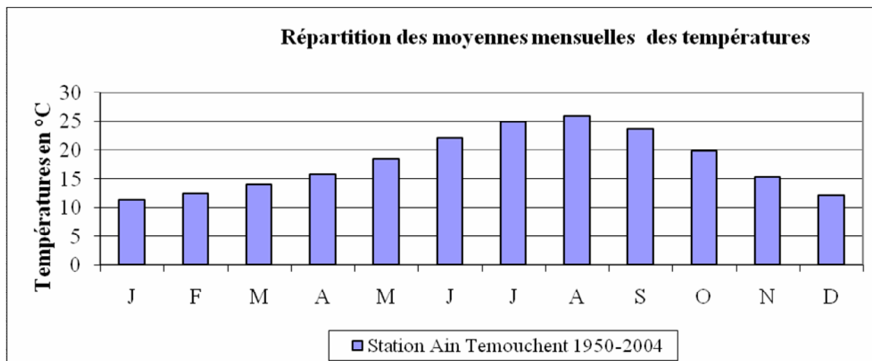
Figure 17 : Températures moyennes mensuelles station Ain Temouchent (1950-2007)
