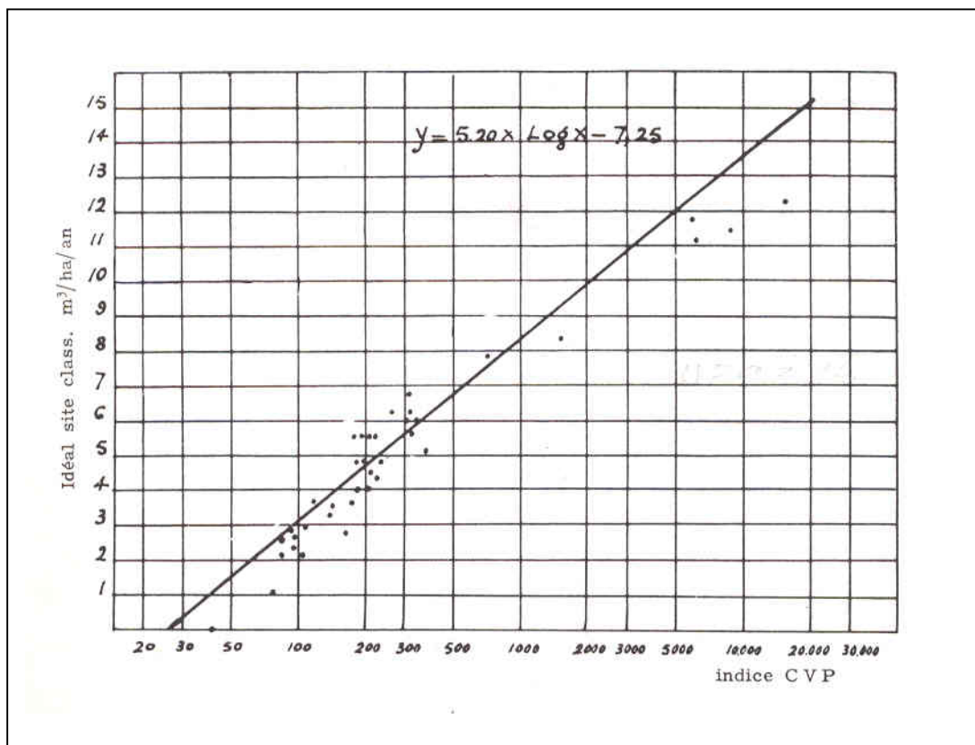
Figure 23 : Relation entre l'indice CVP et la productivité potentielle
