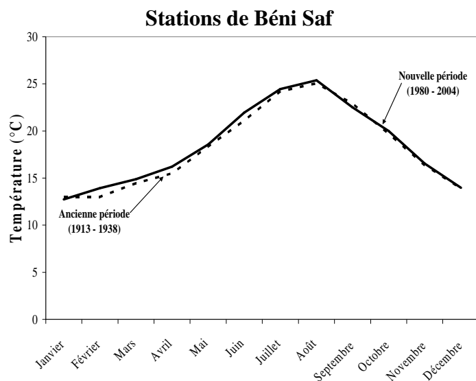
Figure 14 : Moyennes des températures mensuelles durant l'ancienne et la nouvelle période
