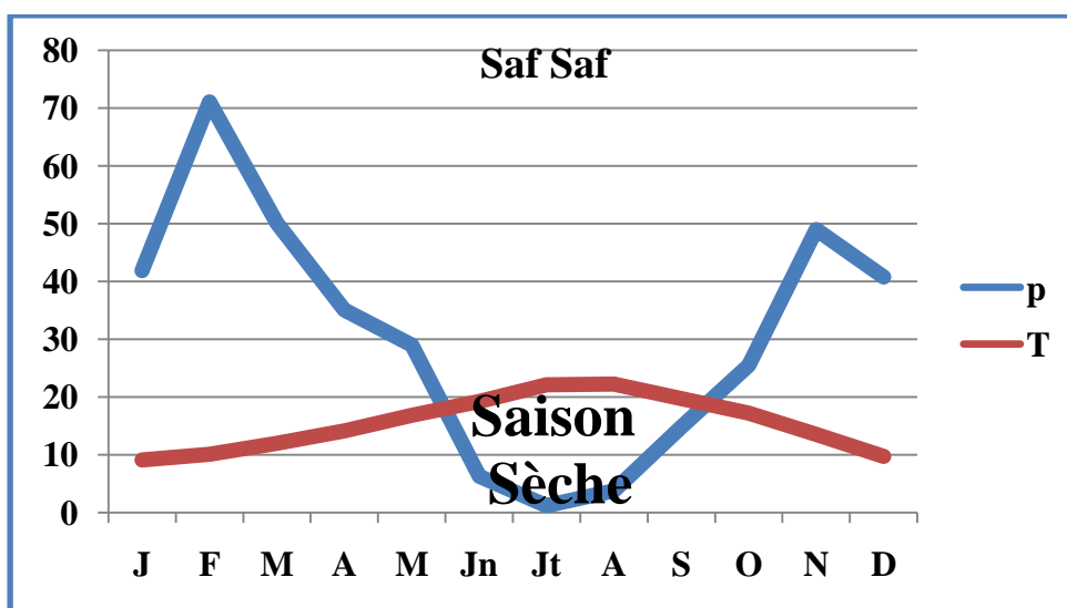
Figure n°15: Diagramme ombrothermique de Bagnouls et Gausson de la station de Saf Saf (1980/2008).
