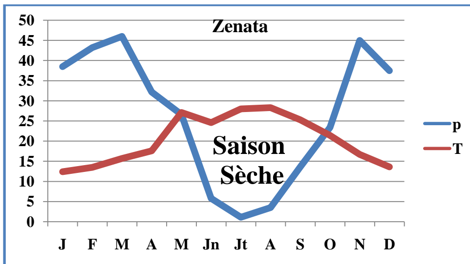
Figure n°14 : Diagramme ombrothermique de Bagnouls et Gausson de la station de Zenata (1980-2008).
