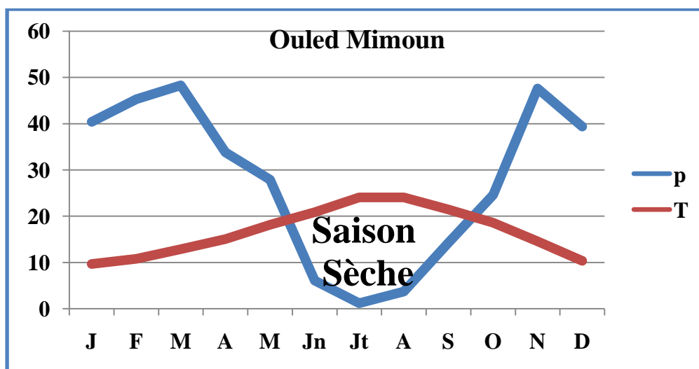
Figure n°16 : Diagramme ombrothermique de Bagnouls et Gausson de la station d'Ouled Mimoun (1980/2008).
