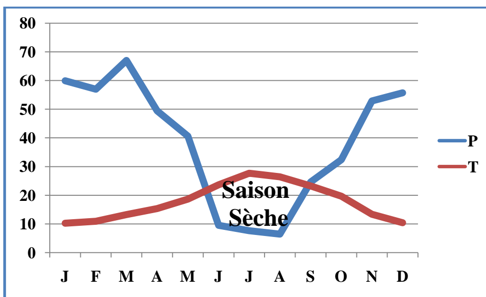
Figure n°17 : Diagramme ombrothermique de Bagnouls et Gausson de la station de Beni Bahdel (1970/2010).
