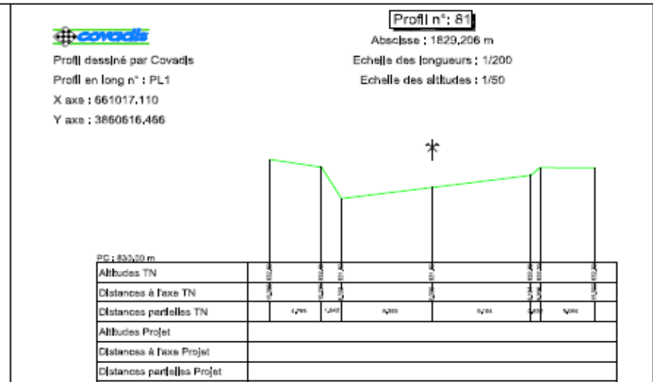
Figure IV.40 : Profil en travers section 81
