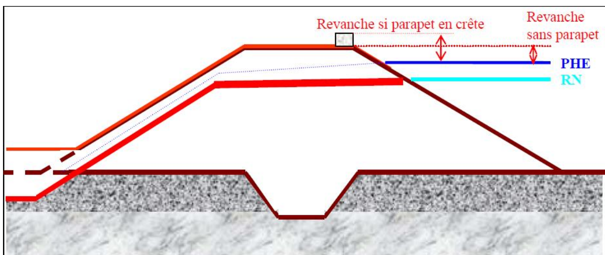
Figure II.11 : Définition des cotes RN, PHE et de la revanche (Naaim et al, 2010).
