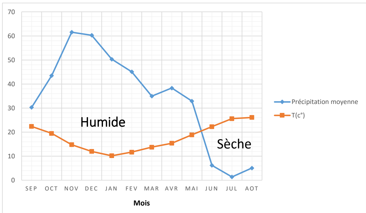
Figure III.26 : Courbe pluviométrique-thermique de la région d'étude.
