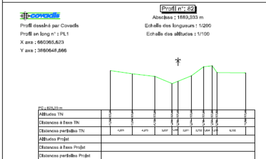
Figure IV.41 : Profil en travers section 82
