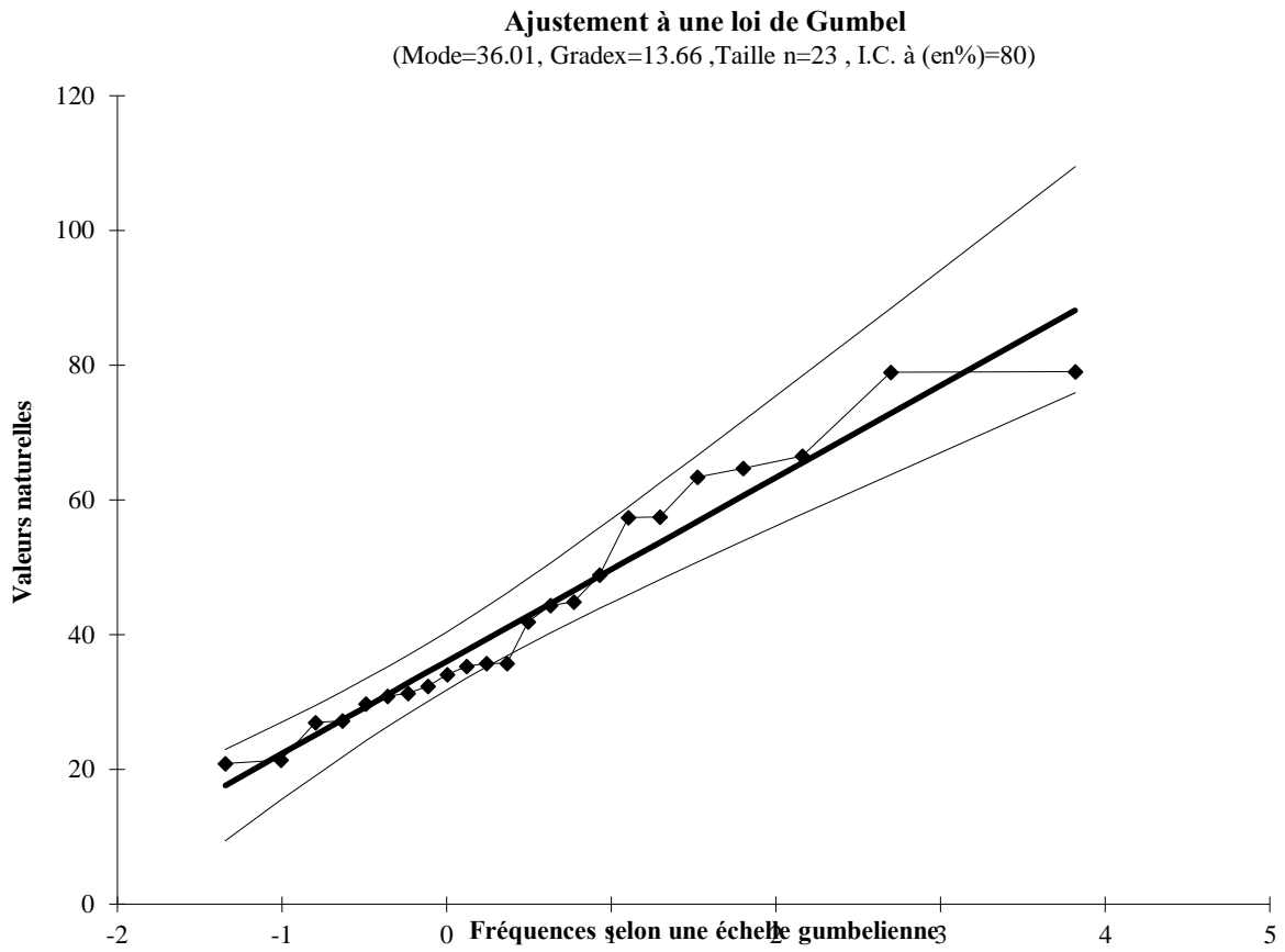
Figure IV.1 : Ajustement de pluies maximum journalier Loi Gumbel
