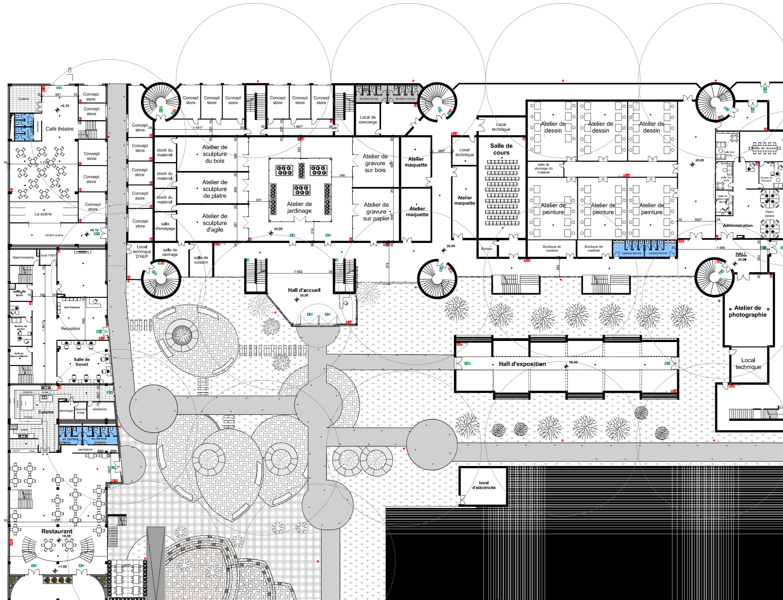
Plan de protection contre incendie
