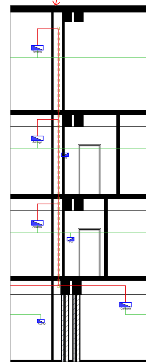
Détail sur la colonne montante (la gaine seche)
