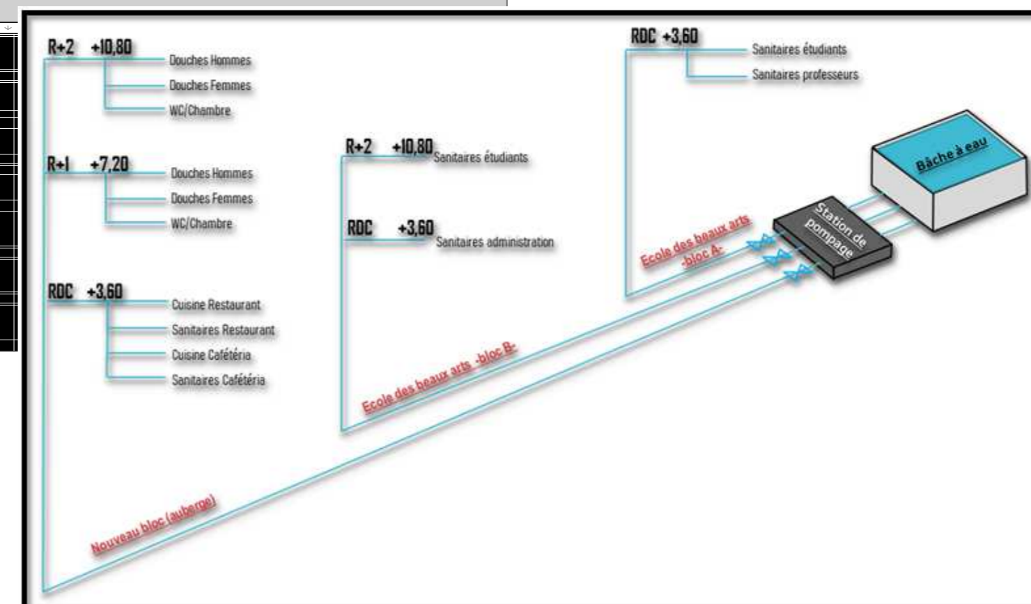
Synoptique de la distribution d'eau potable dans le bâtiment.
