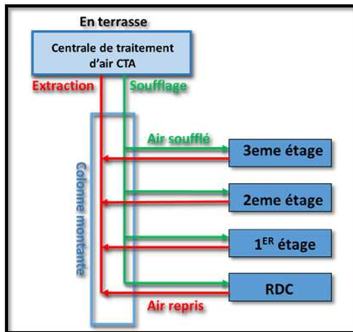
Schéma explicatif du principe du système de climatisation
