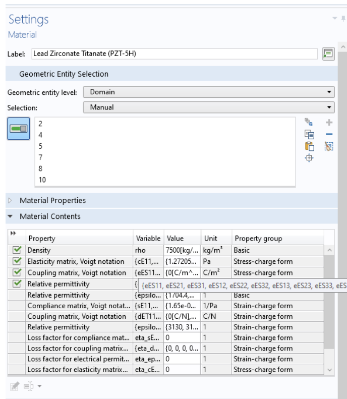
Figure 2.12 Paramètres d'un matériau piézoélectrique dans COMSOL Multiphysics
