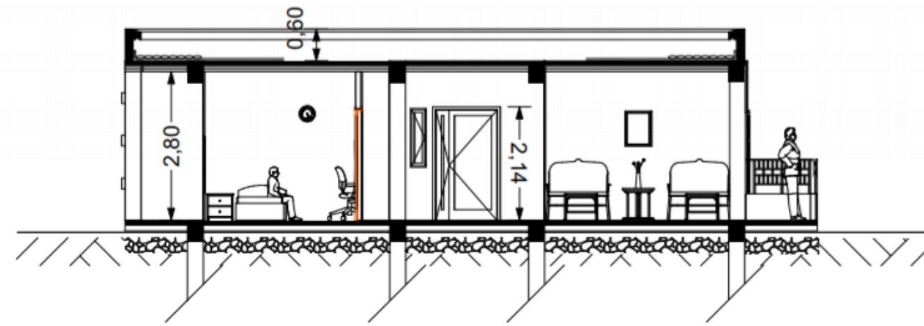
coupe AA
