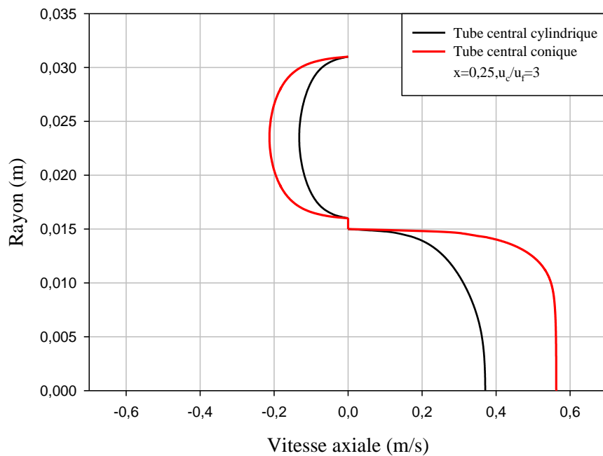
Fig. V. 6. Profil de vitesse axiale à x=L/2 pour un rapport de vitesse u_c/u_f=3
