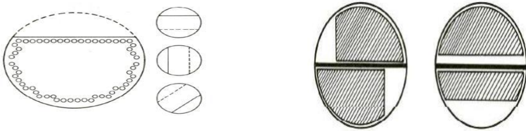
Figure I.13 : Chicanes transversales et longitudinales
