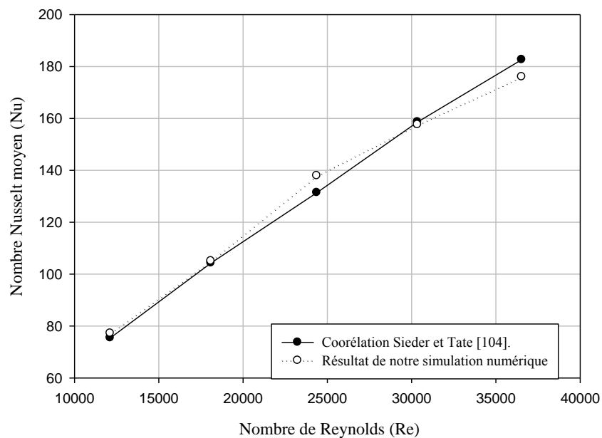
Fig. V. 3. Validation de la présente étude avec les corrélations empiriques de Sieder et Tate [104]. (Espace annulaire)
