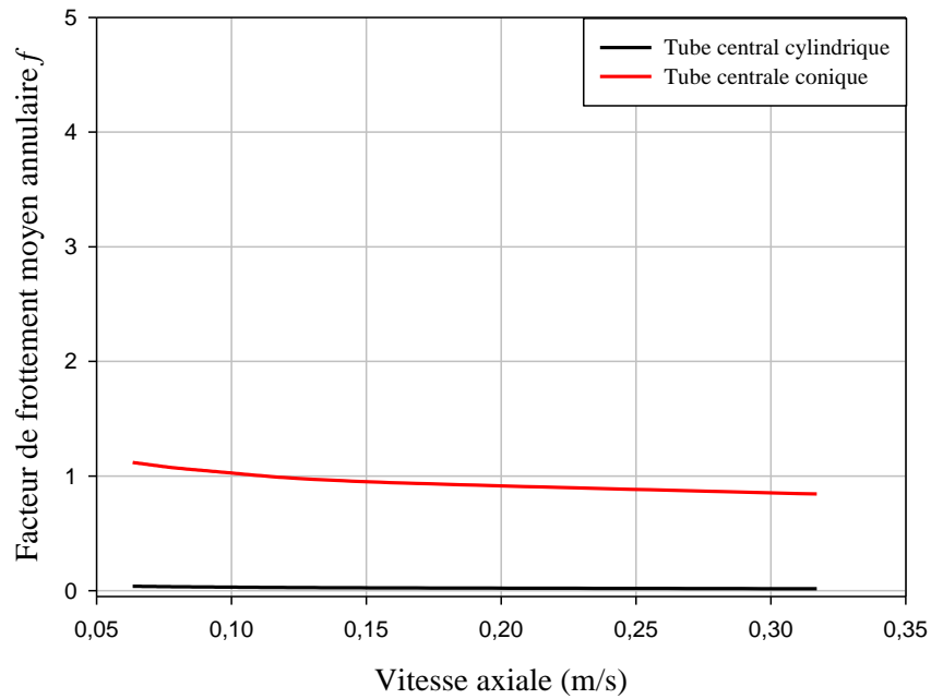
Fig. V. 12. Facteur de frottement moyen annulaire
