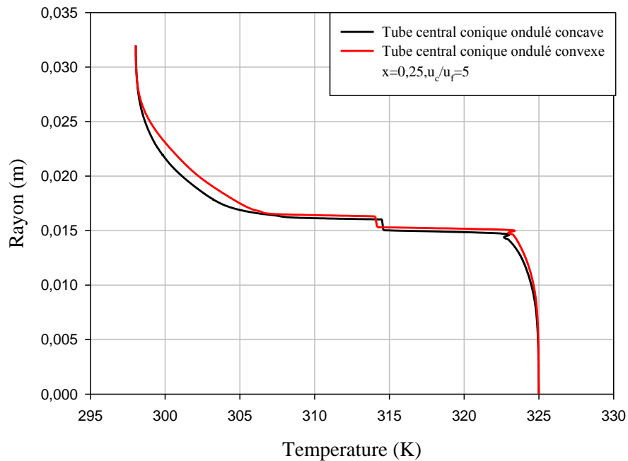
Fig. V. 29. Profil de température pour u_c/u_f=5 étudié dans la section x=0,25 pour les deux arrangements (concave-convexe).
