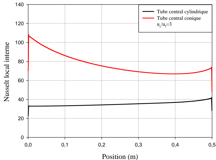
Fig. V. 16. Distribution du nombre de Nusselt local le long de la paroi intérieure du tube centrale conique.
