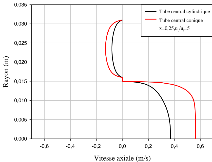
Fig. V. 5. Profil de vitesse axiale à x=L/2 pour un rapport de vitesse u_c/u_f=5 .
