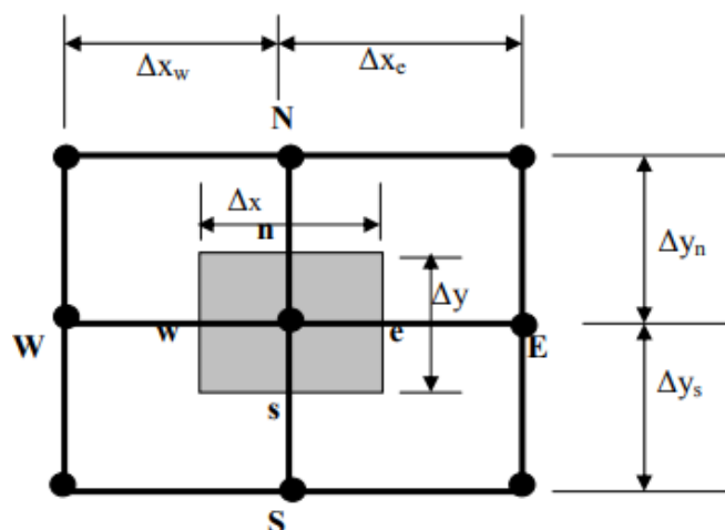
Fig. IV.1: Volume de contrôle bidimensionnel
