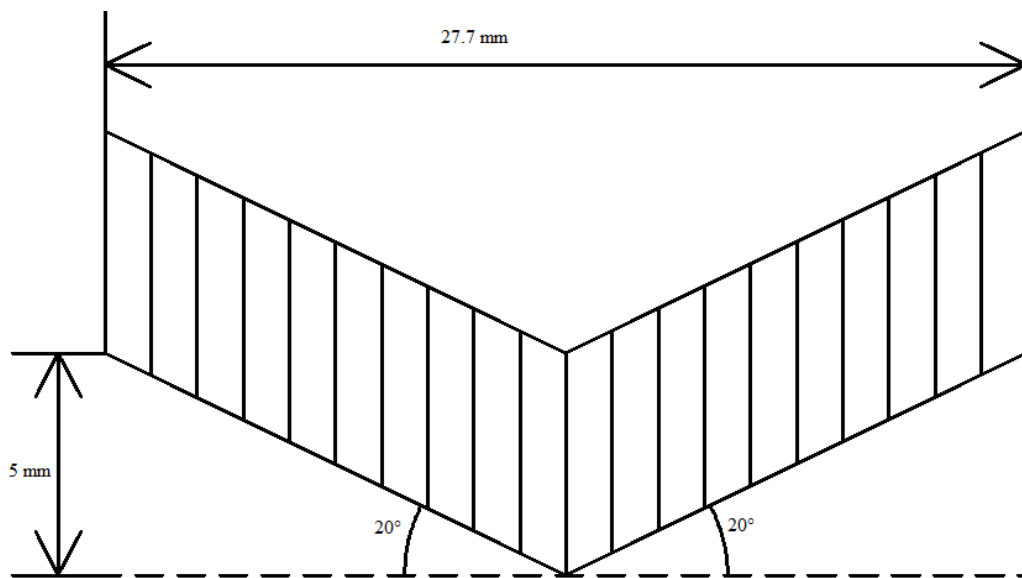
Fig. III.10. La forme d'une ondulation concave
