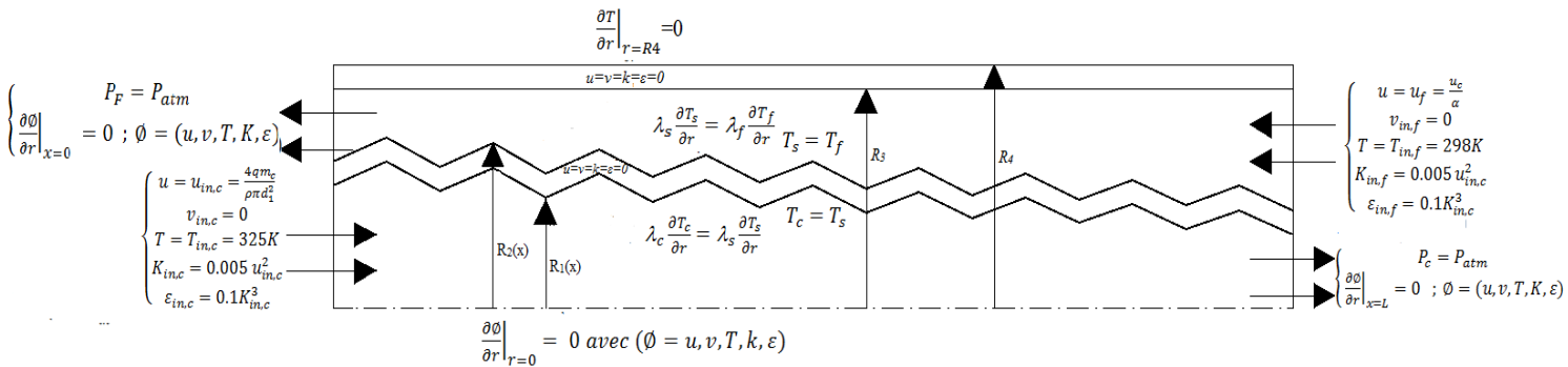
Fig. III.7. Echangeur de chaleur à tubes concentrique à paroi interne ondulée convexe
