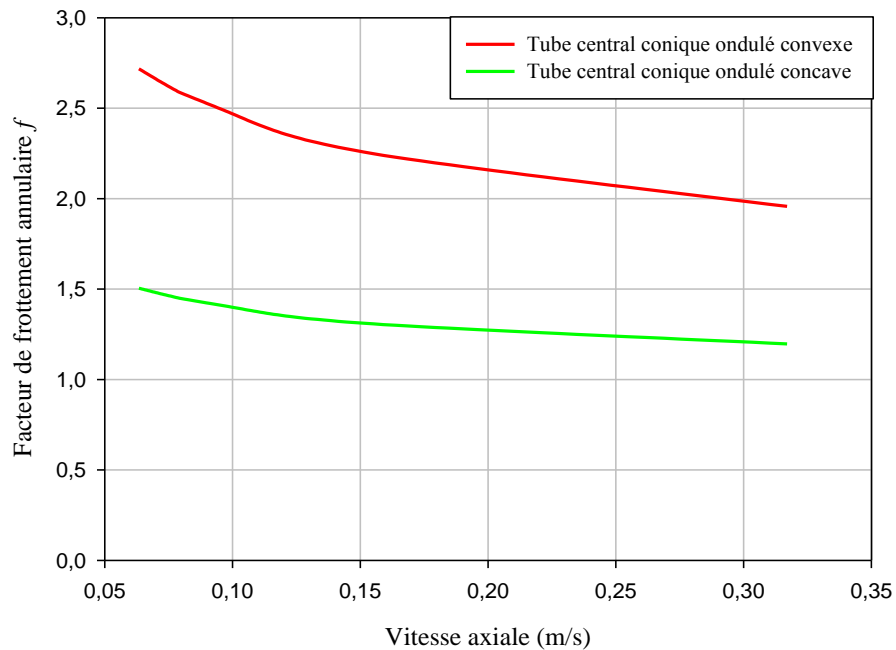
Fig. V. 27. Facteur de frottement moyen annulaire pour différents arrangements d'ondulations.
