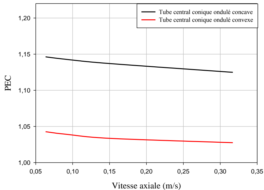
Fig. V. 37. Critère d'évaluation des performances dans le tube annulaire, pour les deux arrangements (concave-convexe).
