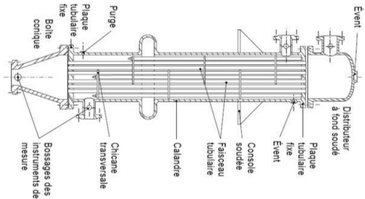
Figure I.16 : .Echangeur a plaque tubulaires fixes
