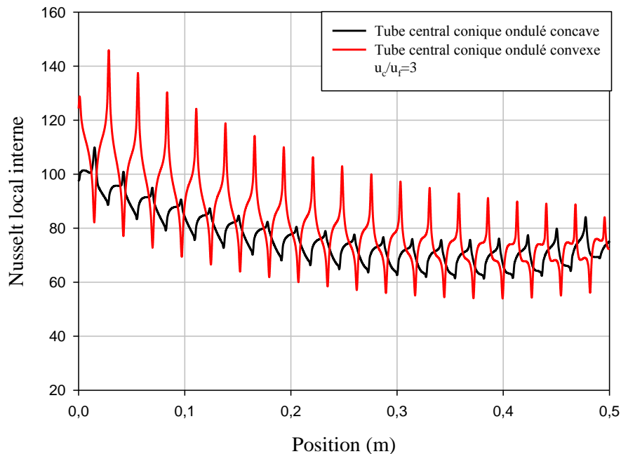
Fig. V. 32. Nusselt local interne pour u_c/u_f=3 pour différents arrangements (concave-convexe).
