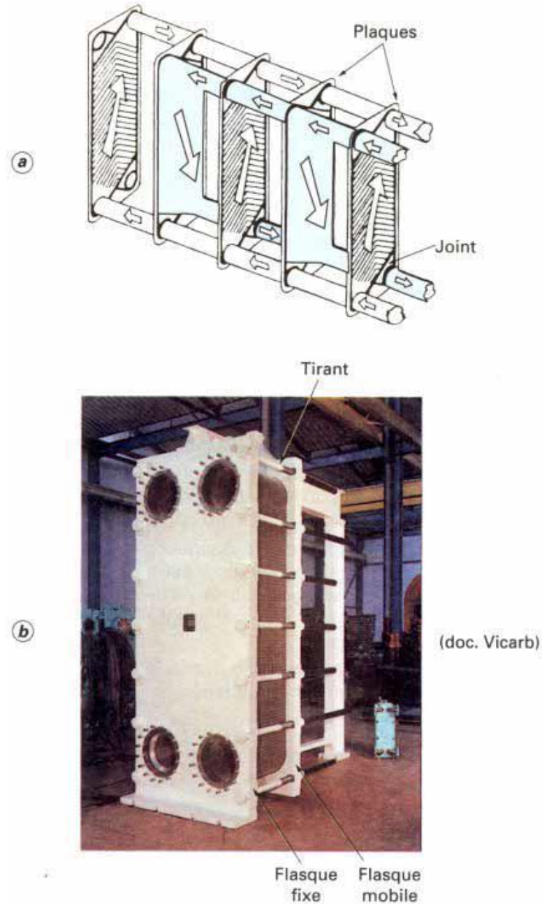
Figure I.20 : Echangeurs à plaques et joint
