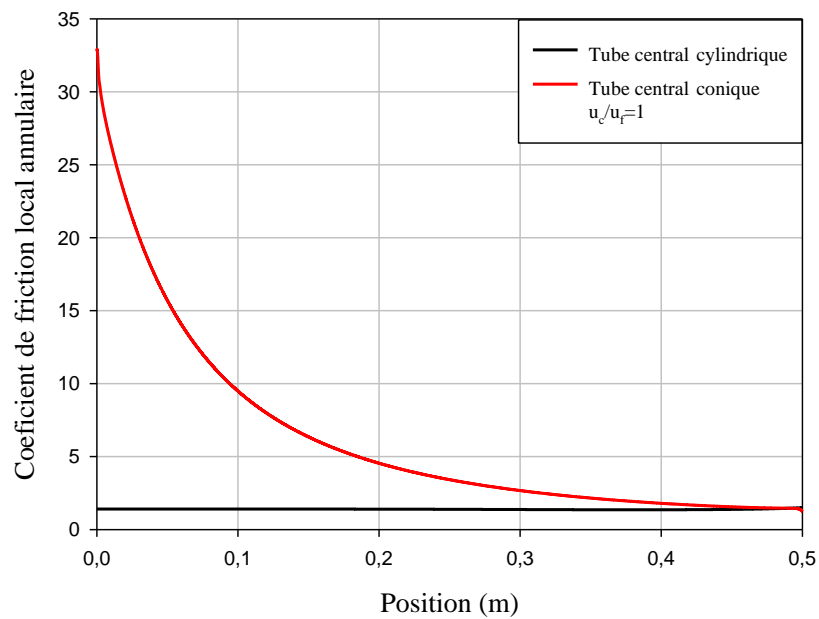
Fig. V. 11. Coefficient de friction local pour u_c/u_f=1 le long de la paroi externe du tube interne pour la géométrie conique et cylindrique
