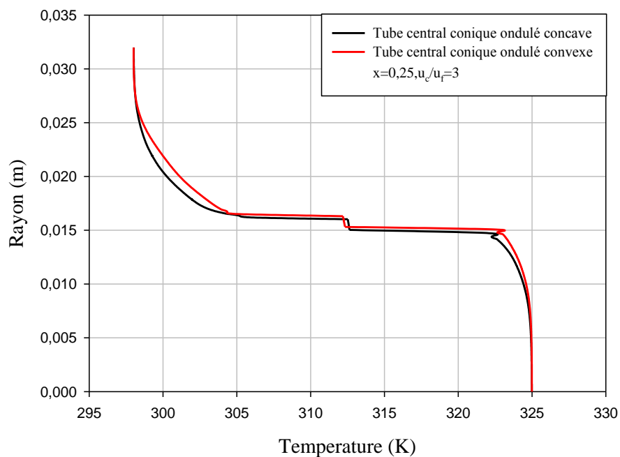
Fig. V. 30. Profil de température pour u_c/u_f=3 étudié dans la section x=0,25 pour les deux arrangements (concave-convexe).
