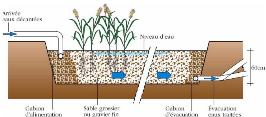
Figure 0.3: Coupe représentative d'un filtre à écoulement horizontal [71].
