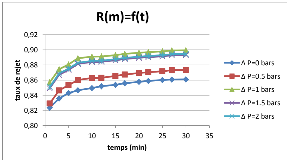
Figure VI.56: La variation du taux de rejet en fonction de temps ( P_{\text{entrée}}=10,5 bar ; \Delta P = 0 ; 0.5 ; 1 ; 1.5 ; 2 ; C=5 g/L).
