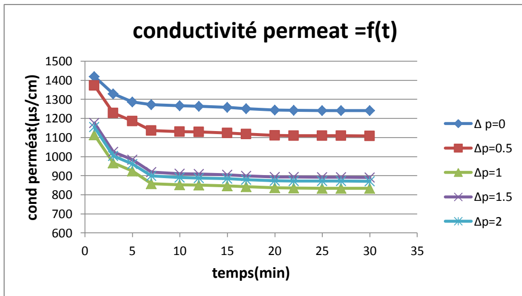
Figure VI. 9: La variation de la conductivité de perméat en fonction du temps ( P_{\text{entrée}}=5.5\text{ bar} ; \Delta P= 0; 0.5; 1 ; 2 ; C=3\text{g/L} ).
