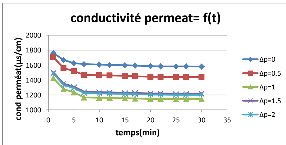
Figure VI.37: La variation de la conductivité de perméat en fonction du temps (P entrée =10.5 bar ; ΔP= 0; 0.5; 1; 1.5 ; 2 ; C=5g/L).
