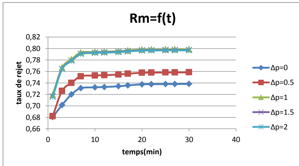
Figure VI.8: La variation de taux de rejet en fonction du temps ( P_{\text{entrée}}= 5.5 bar ; \Delta P= 0; 0.5;1;2 ; C=2\text{g/L} ).
