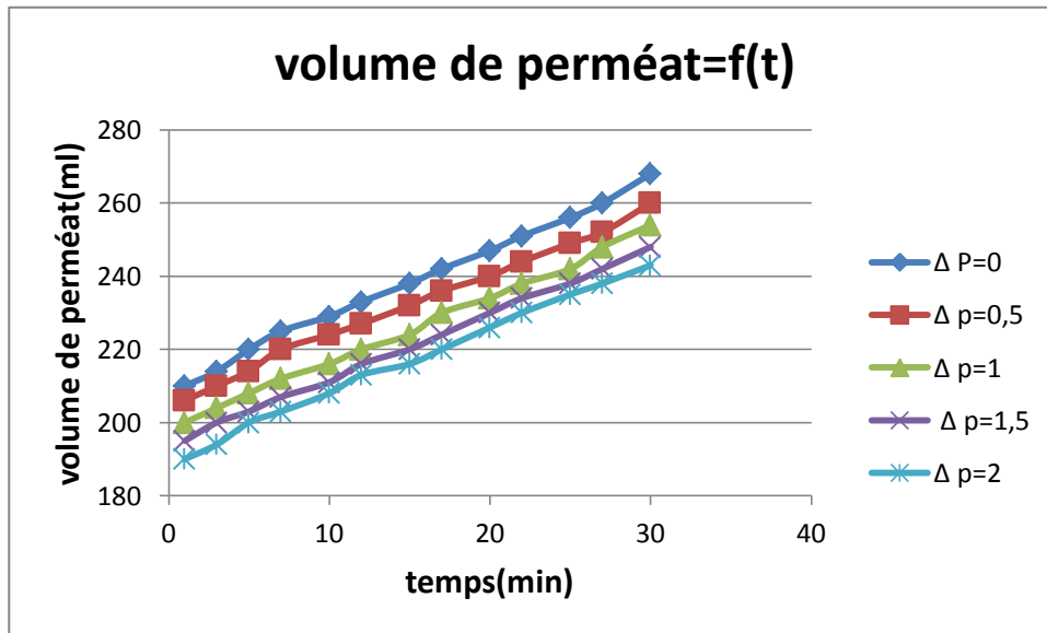
Figure VI.27: La variation de volume de perméat en fonction du temps ( P_{\text{entrée}}=10.5 bar ; \Delta P= 0; 0.5; 1; 1.5; 2 ; C=4g/L ).
