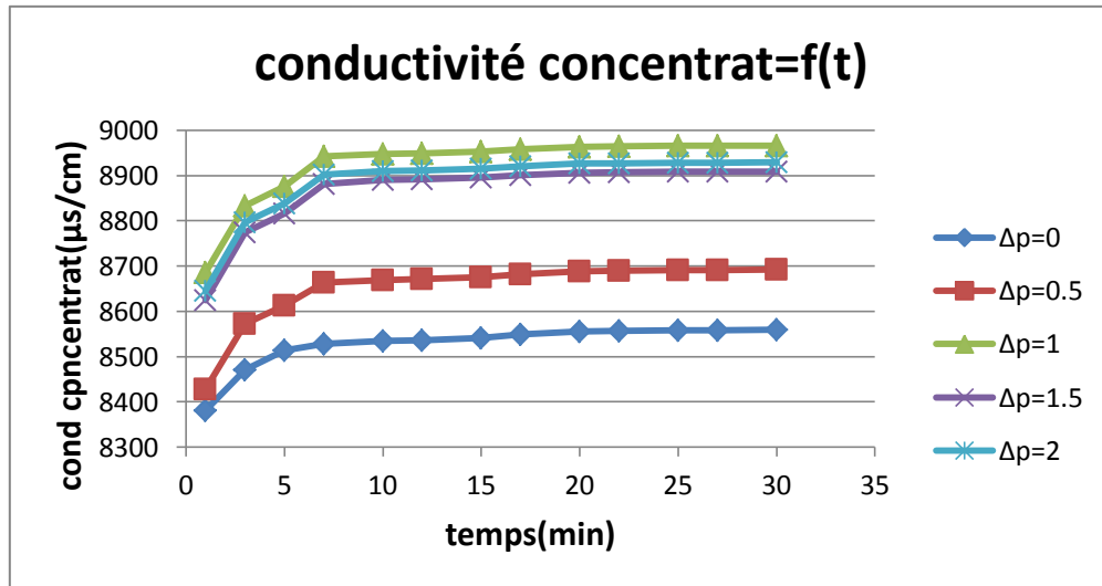
Figure VI.10 : La variation de la conductivité de concentrât en fonction du temps (Pentrée=5.5 bar ; ΔP= 0; 0.5;1 ; 2 ; C=3g/L).
