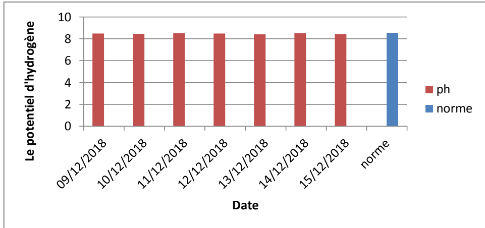
Figure IV.22: Comparaison des valeurs de pH avec la norme Algérienne.
