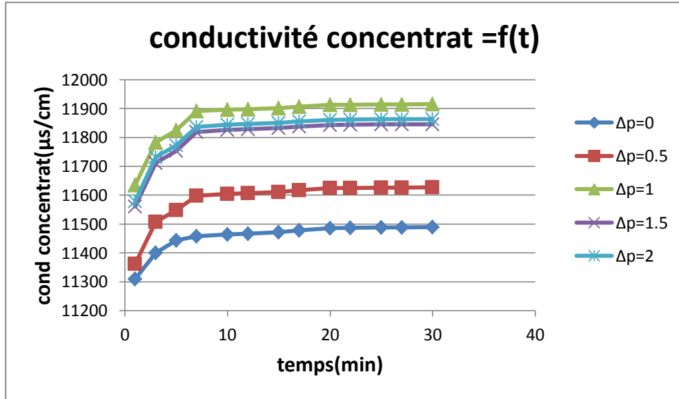
Figure VI.26: La variation de la conductivité de concentrât en fonction du temps ( P_{\text{entrée}}=10.5 bar ; \Delta P= 0; 0.5; 1; 1.5; 2 ; C=4g/L ).
