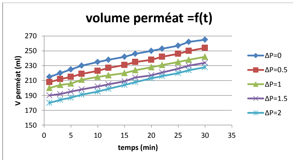
Figure VI.55: La variation du volume du perméat en fonction du temps ( P_{\text{entrée}}=10.5 bar ; \Delta P= 0 ; 0.5 ; 1 ; 2 ; C=5g/L )
