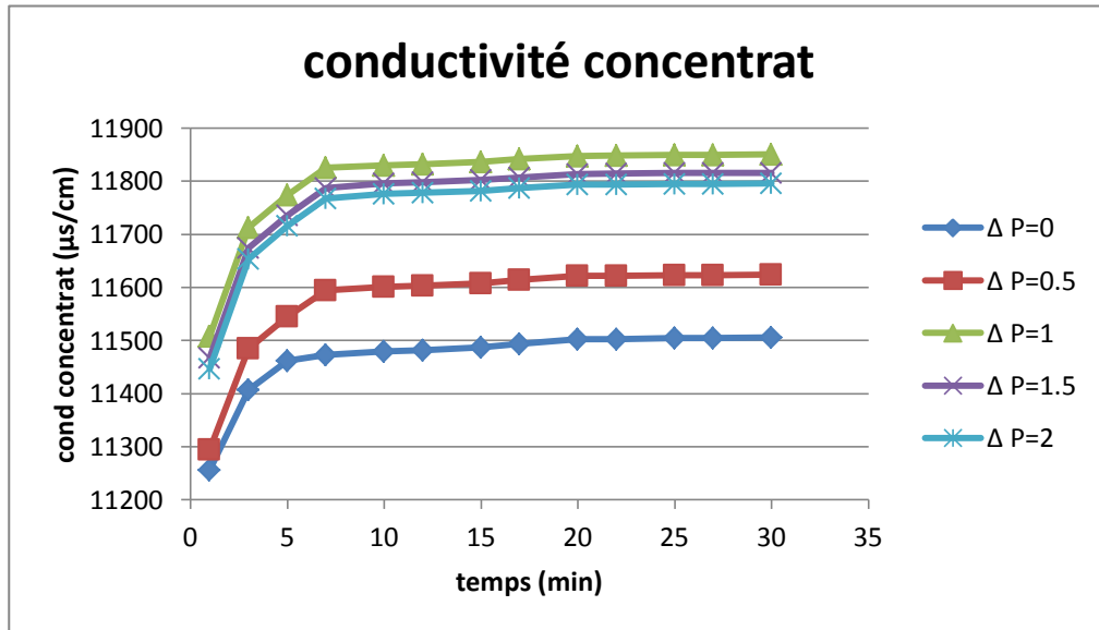
Figure VI.18: La variation de la conductivité de concentrât en fonction du temps ( P_{\text{entrée}}=5.5 bar ; \Delta P= 0; 0.5; 1 ; 1.5 ; 2 ; C=4g/L ).
