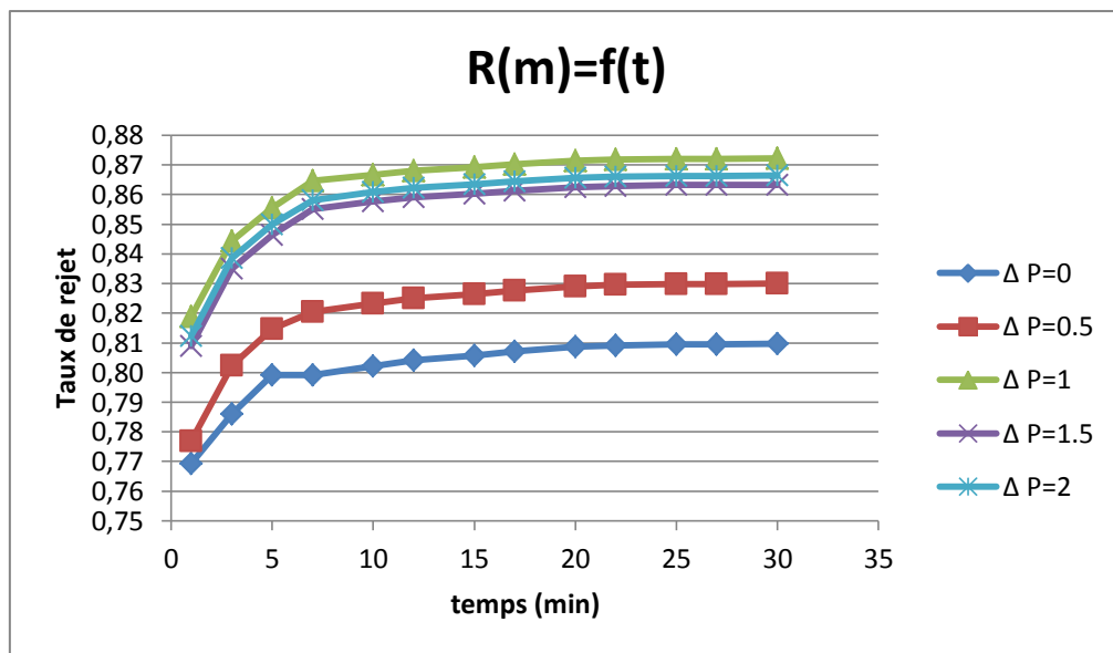
Figure VI.44: La variation du taux de rejet en fonction du temps ( P_{\text{entrée}}=5.5 \text{ bar} ; \Delta P= 0; 0.5;1;1.5 ; 2 ; C=3\text{g/L} ).
