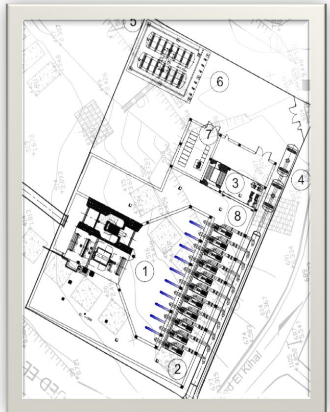
Figure IV. 3: plan de bâtiment de captage [57].
