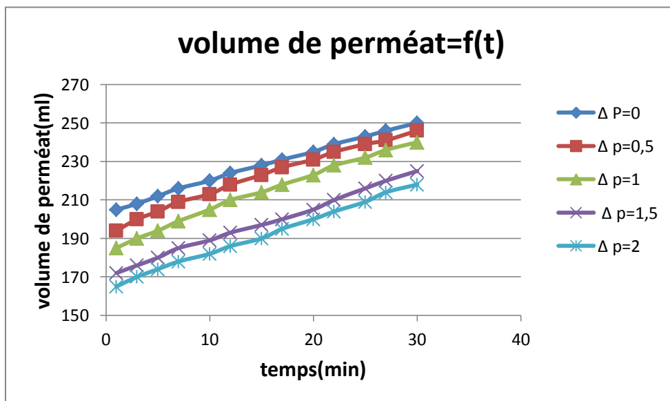
Figure VI.35: La variation de volume du perméat en fonction du temps ( P_{\text{entrée}}=8.5 bar ; \Delta P= 0; 0.5;1;1.5 ; 2 ; C=5g/L ).
