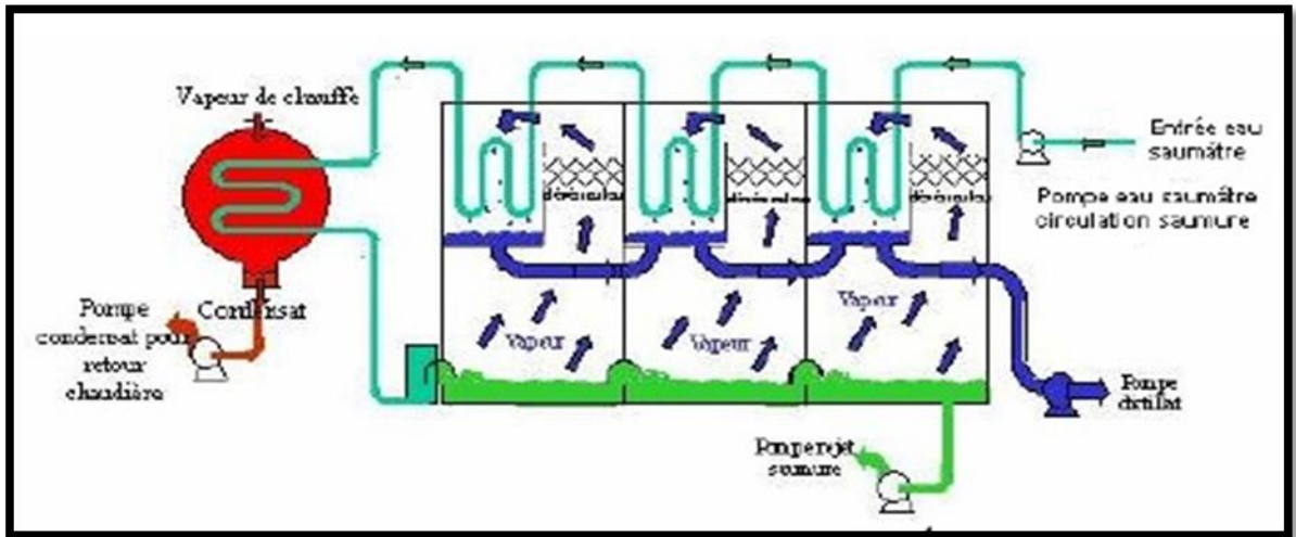
Figure II.5 : Schéma de principe d'un système de distillation par détentes successives [E].
