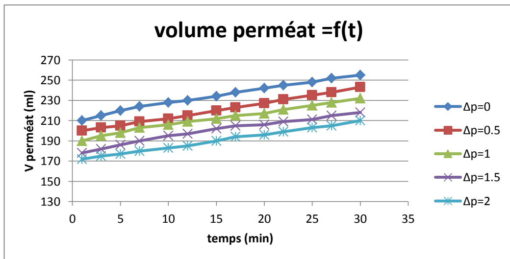
Figure VI.43: La variation du volume du perméat en fonction du temps ( P_{\text{entrée}}=5.5 bar ; \Delta P= 0; 0.5; 1; C=3\text{g/L} ).
