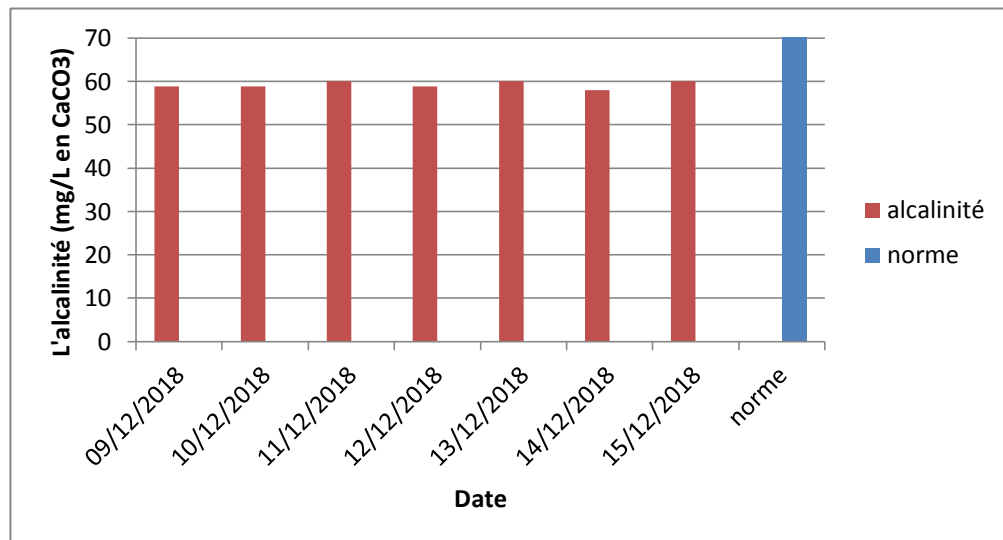
Figure IV.17: Comparaison de valeurs d'alcalinité avec la norme algérienne.
