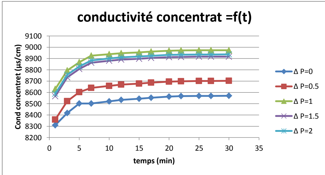
Figure VI.42: La variation de la conductivité du concentrât en fonction du temps ( P_{\text{entrée}}=5.5 bar ; \Delta P= 0; 0.5; 1 ; 1.5 ; 2; C=3\text{g/L} ).
