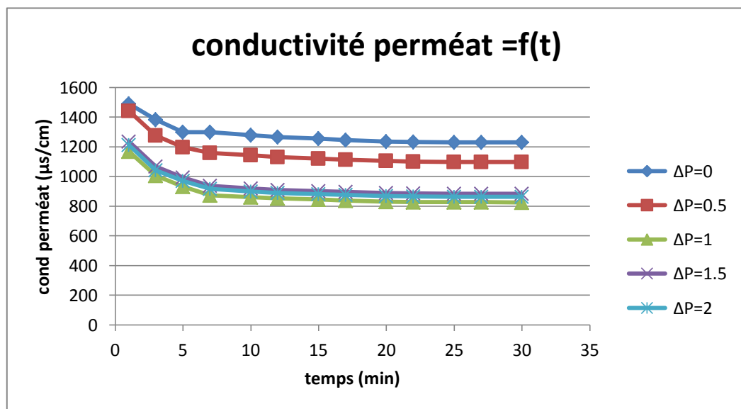
Figure VI.41: La variation de la conductivité du perméat en fonction du temps ( P_{\text{entrée}}=5.5\text{ bar} ; \Delta P= 0; 0.5; 1; 1.5 ; 2 ; C=3\text{g/L} ).
