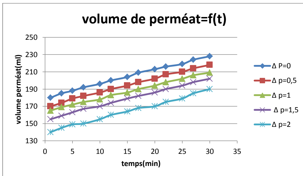
Figure VI.19 : La variation de volume de perméat en fonction du temps ( P_{\text{entrée}}=5.5 bar ; \Delta P= 0; 0.5; 1 ; 1.5 ; 2 ; C=4g/L ).
