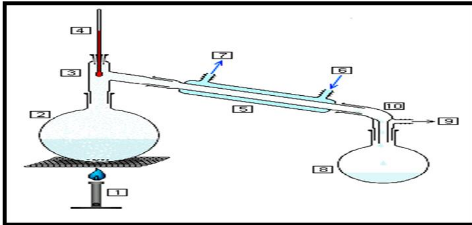
Figure II.2 : schéma de principe de distillation [B].
