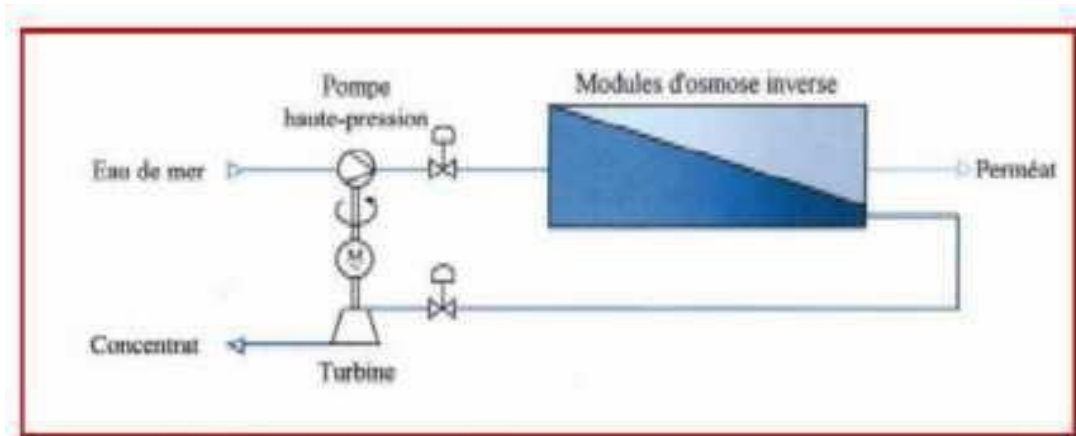
Figure II.15 : Récupération de l'énergie du concentrât par turbin Pelton [13].
