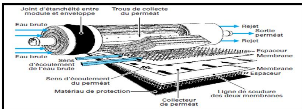
Figure II.12 : Représentation d'un module spirale [32].
