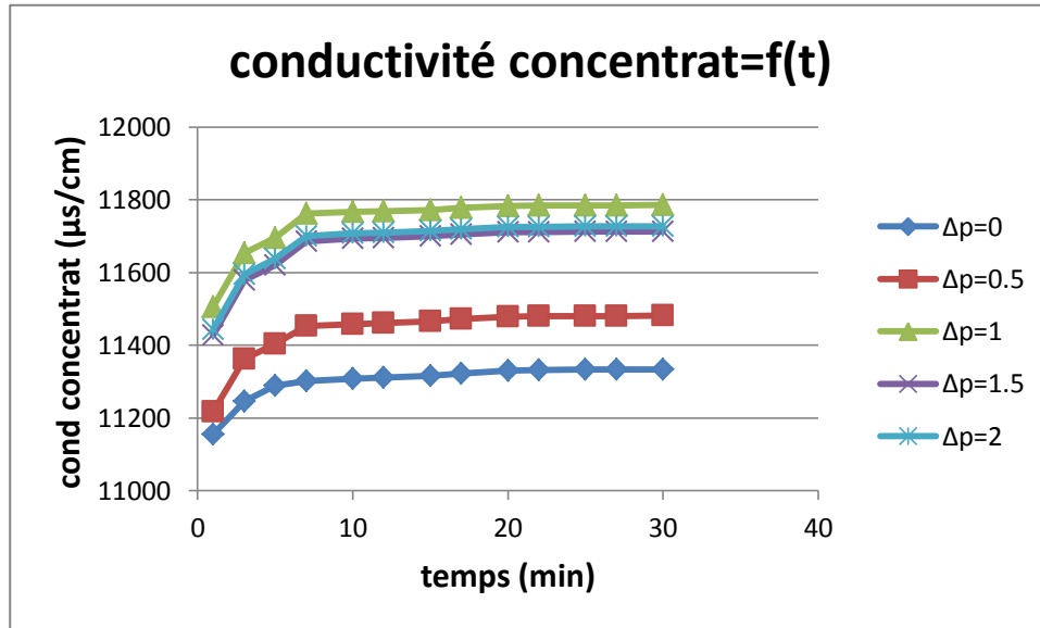
Figure VI.30: La variation de la conductivité de concentrât en fonction du temps (P entrée =5.5 bar ; ΔP= 0; 0.5;1;1.5 ; 2 ; C=5g/L).
