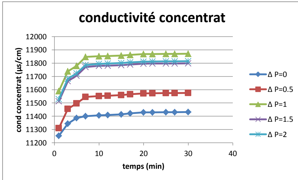
Figure VI.34: La variation de la conductivité de concentrât en fonction du temps ( P_{\text{entrée}}=8.5 bar ; \Delta P= 0; 0.5;1;1.5 ; 2 ; C=5g/L ).
