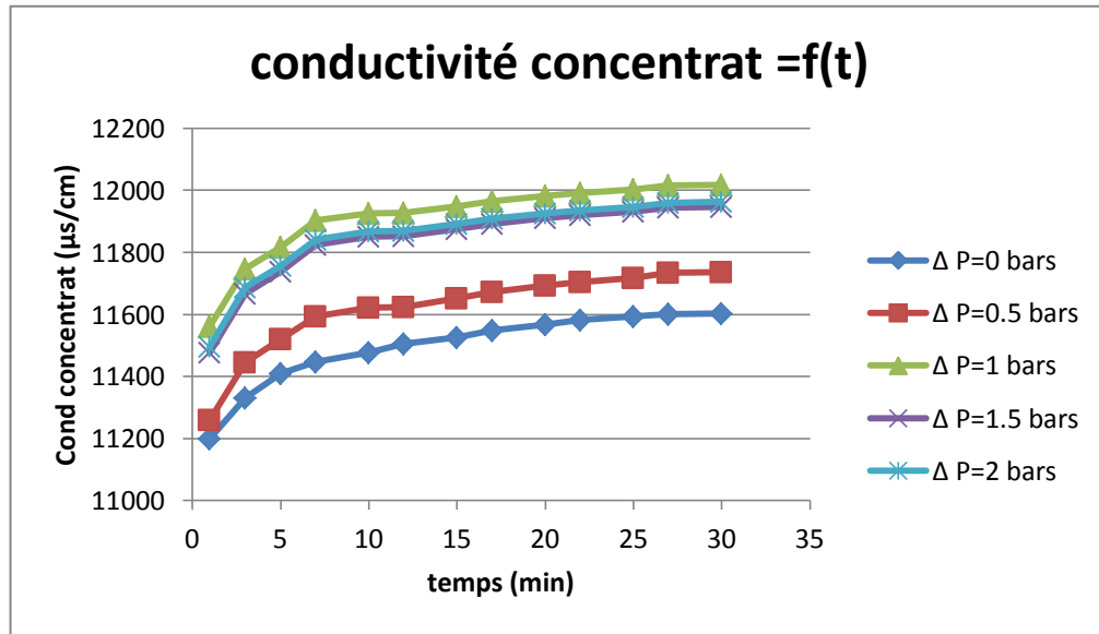
Figure VI.54: La variation de la conductivité du concentrât en fonction du temps ( P_{\text{entrée}}=10,5 bar ; \Delta P = 0 ; 0.5 ; 1 ; 1.5 ; 2 ; C=5g/L ).
