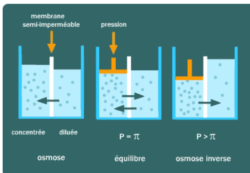
Figure II.8: Principe des phénomènes d'osmose et d'osmose inverse [28].
