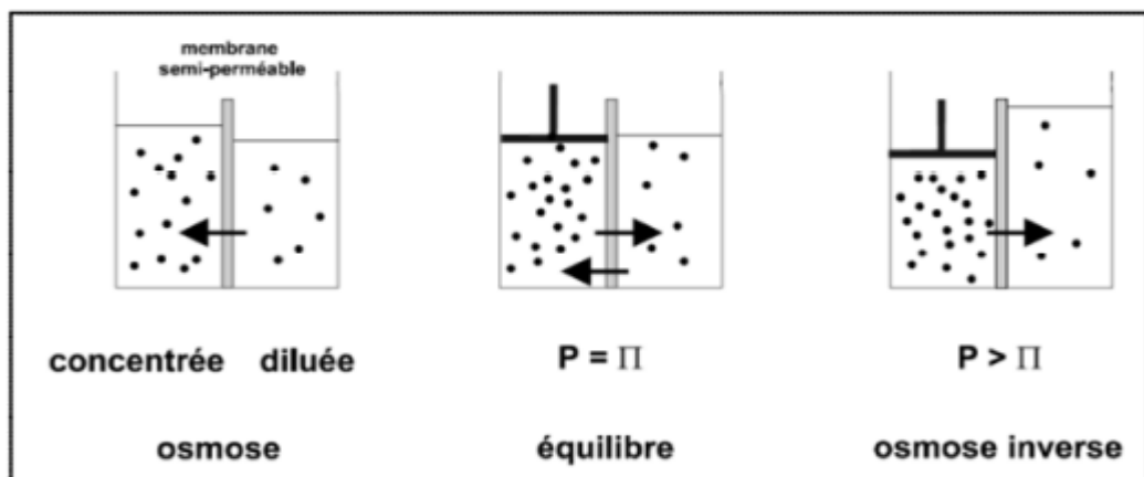
Figure II.9 : Représentation de la pression osmotique [24].
