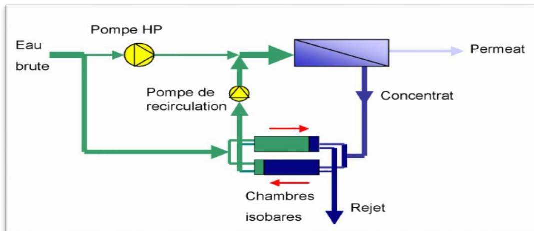
Figure II.16 : schéma récupération d'énergie par échangeurs de pression [6].
