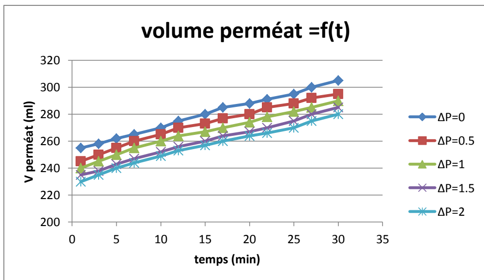
Figure VI.47: La variation du volume du perméat en fonction du temps (P entrée =8.5 bar ; ΔP= 0; 0.5;1; C=3g/L).
