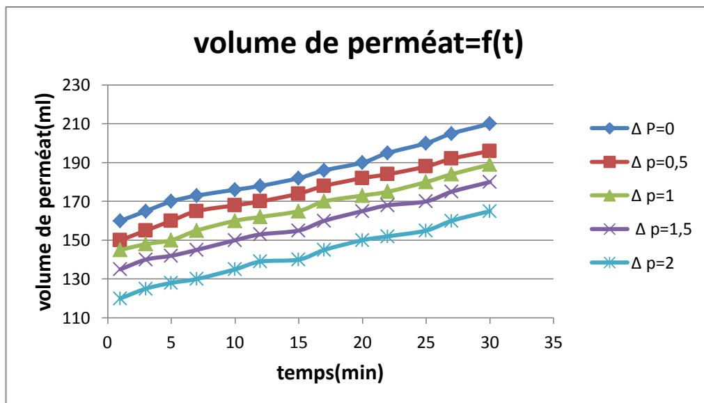
Figure VI.31: La variation de volume du perméat en fonction du temps (P entrée =5.5 bar ; ΔP= 0; 0.5;1;1.5 ; 2 ; C=5g/L).
