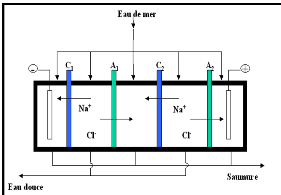
Figure II.7 : Principe de l'électrodialyse [25].
