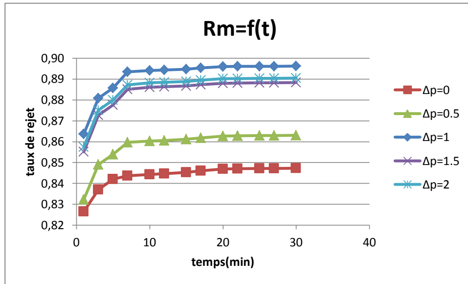
Figure VI.24: La variation de taux de rejet en fonction du temps ( P_{\text{entrée}}=8.5 bar ; \Delta P= 0; 0.5; 1 ; 1.5; 2 ; C=4\text{g/L} ).
