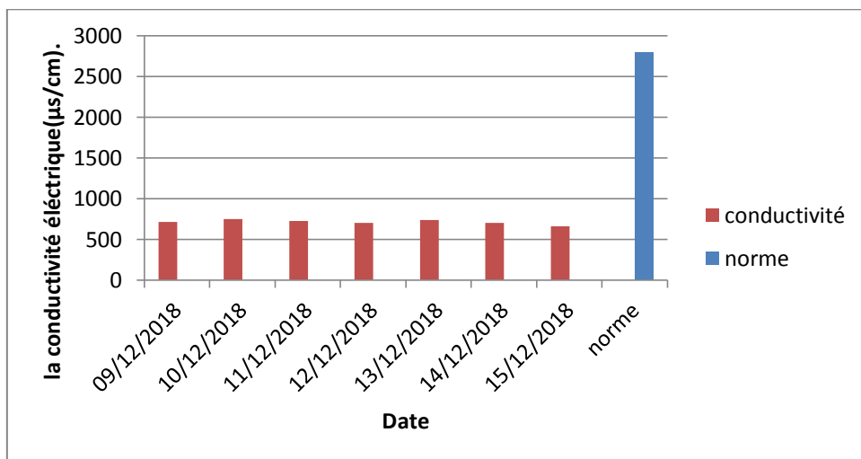
Figure IV.25: Comparaison des résultats de la conductivité avec la norme Algérienne.
