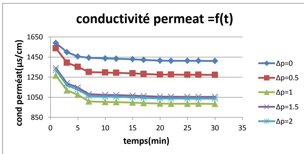
Figure VI.25: La variation de la conductivité de perméat en fonction du temps ( P_{\text{entrée}}=10.5 bar ; \Delta P= 0; 0.5;1 ; 1.5 ; 2 ; C=4\text{g}/\text{L} )
