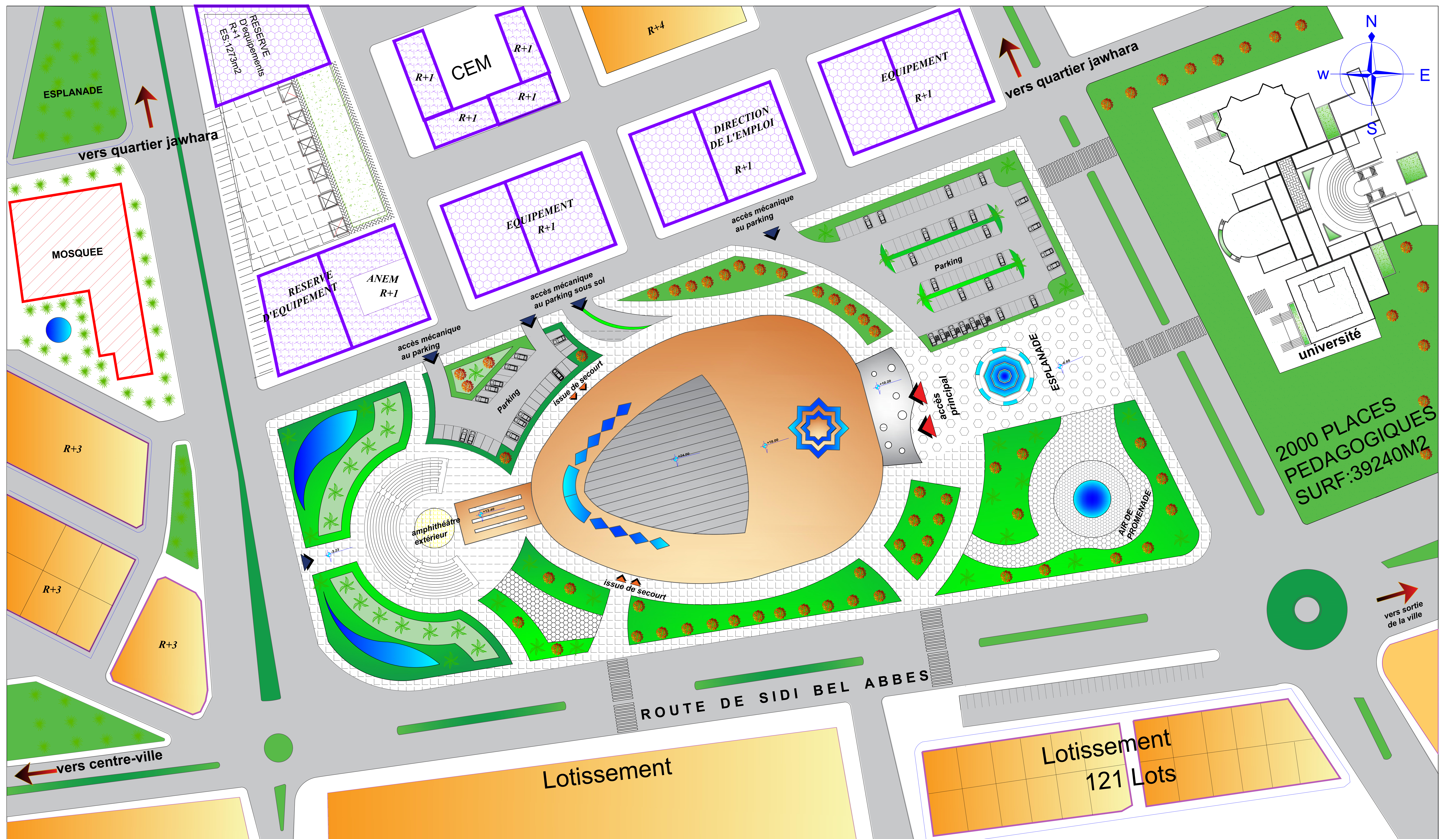
PLAN DE MASSE ECH: 1/400
