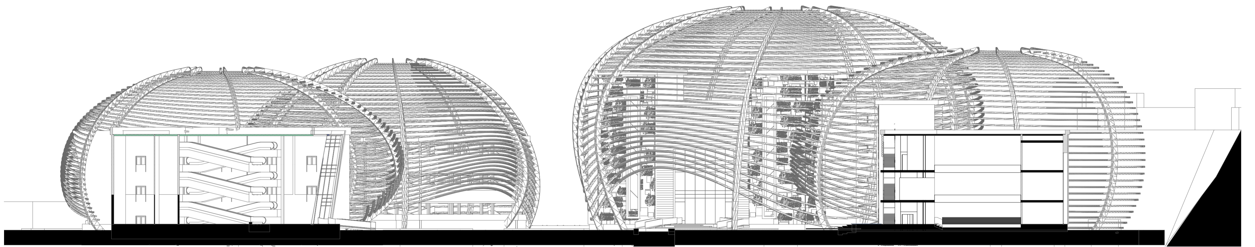
Coupe BB 1/200
