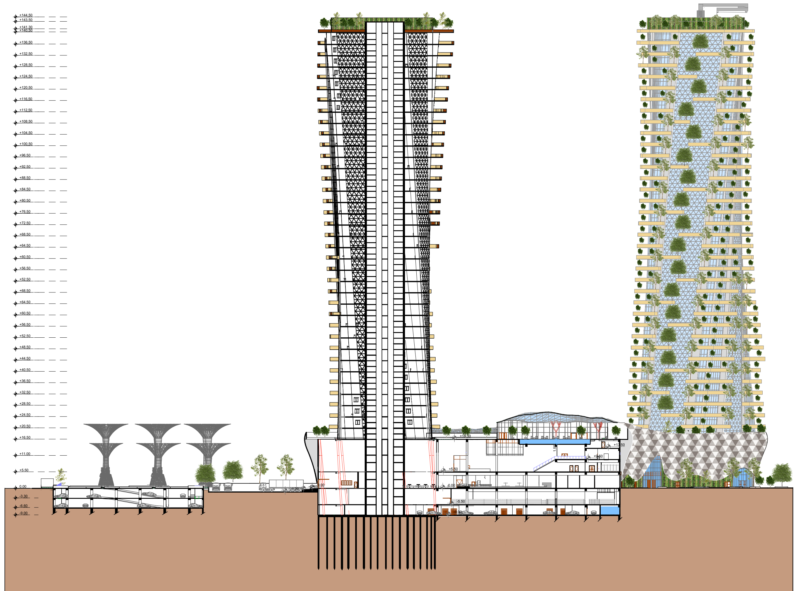
COUPE A-A
