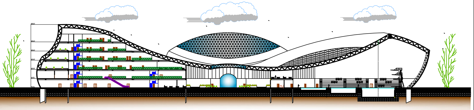
COUPE A-A
