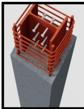
Figure 137. Exemple d'un profilé métallique enrobé
