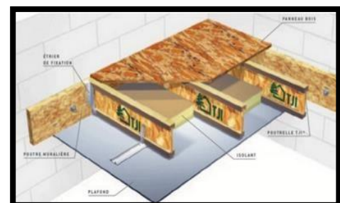
Figure 10. Structure mixte bois-métal
