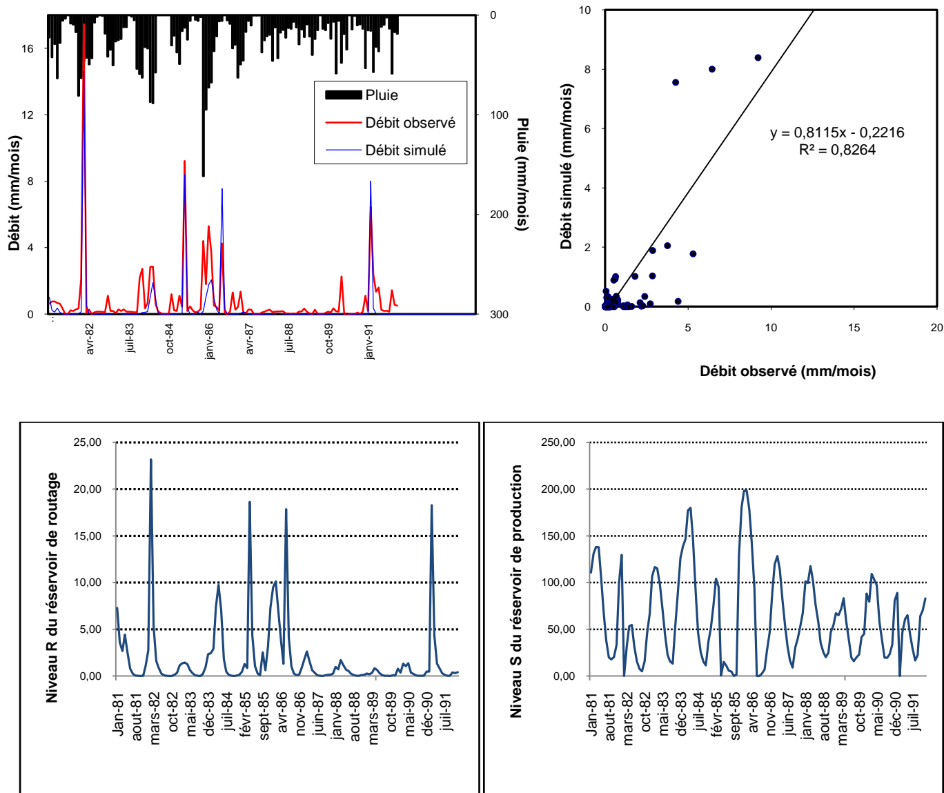
Figure III.8 Calage du modèle GR2M, précipitations moyennes de stations (Saida + Sidi-Boubkeur)
