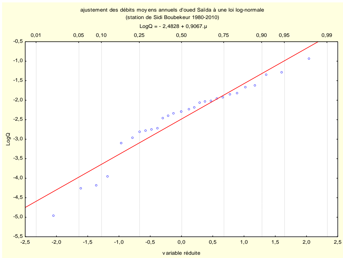
Figure II.11 Ajustement des débits moyens annuels à une loi Log-normal
