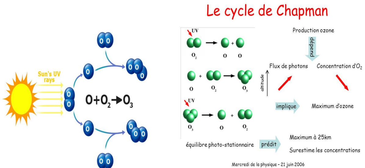
Figure I-16 : Cycles de Production Naturelle de l'Ozone- Cycle de Chapman [46], (47).
