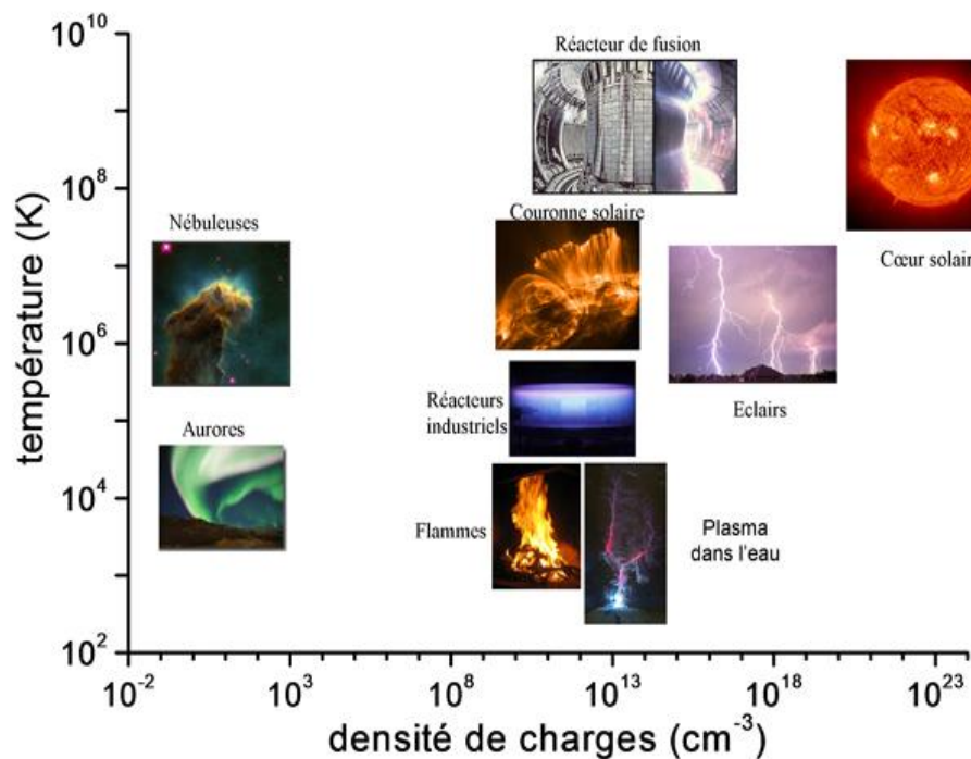
Figure I-2 : Classification des Plasmas Naturels et de Laboratoire dans un Diagramme Logarithmique Densité de Charges/Température [5].
