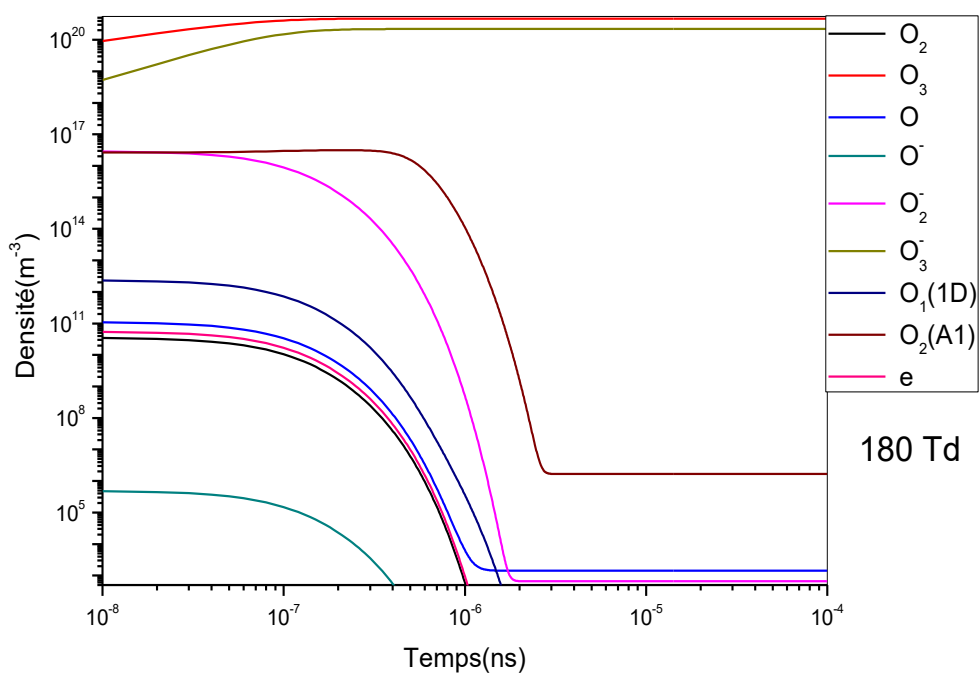
Figure III-12 : Evolution Temporelle de la Densité des Espèces à 180Td.
