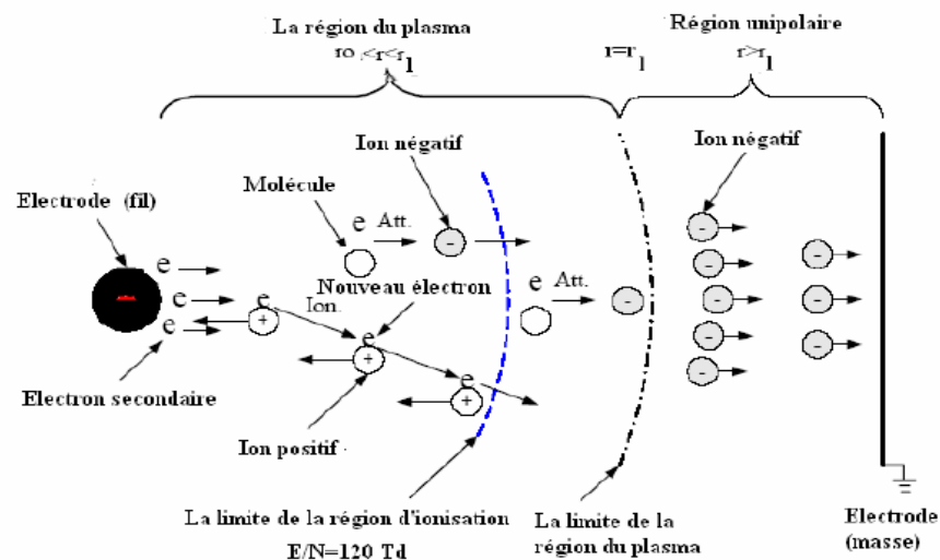
Figure I-14 : Processus d'Une Décharge Electrique Couronne Négative [30].
