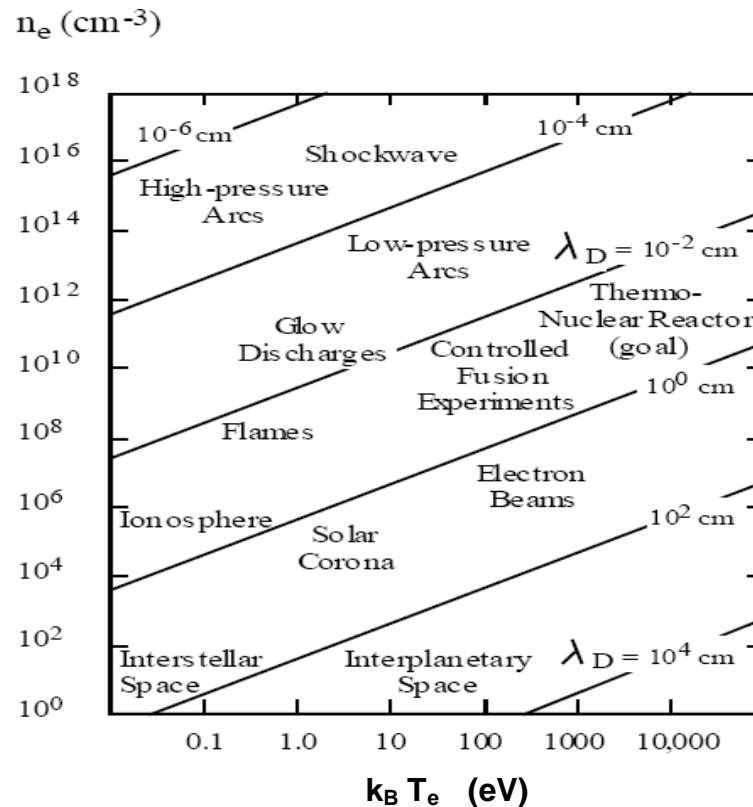
Figure I-7 : Classification des Plasmas Selon leur Energie Electronique k_B T_e , leur Densité Electronique n_e et leur longueur de Debye \lambda_D (cm) [12].
