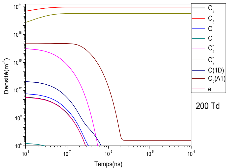
Figure III-13 : Evolution Temporelle de la Densité des Espèces à 200Td.
