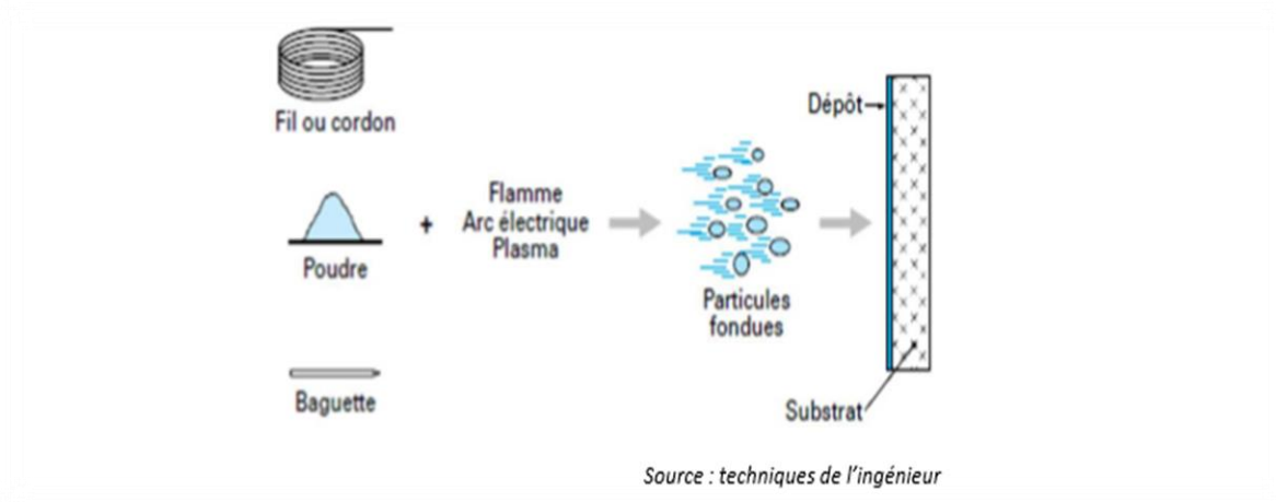
Figure 2.1 : principe de projection thermique
