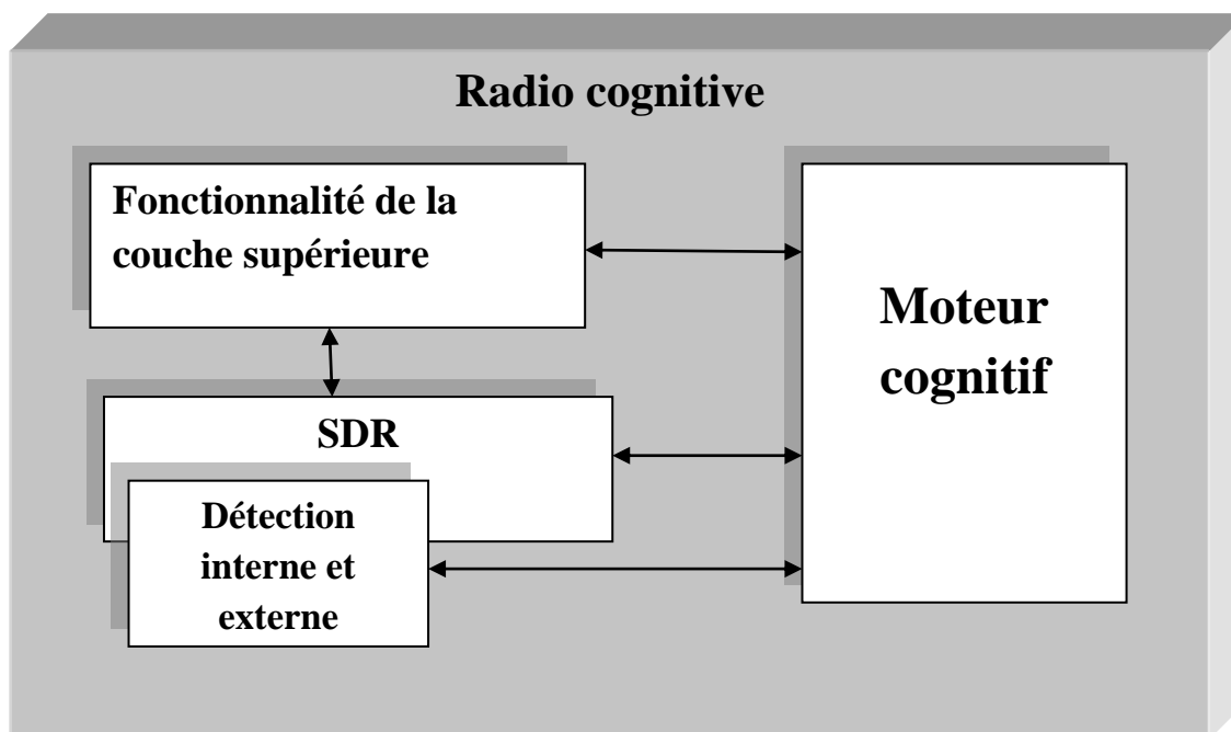
Figure I. 1 : Relation entre la radio cognitive et la radio logicielle restreinte [4]
