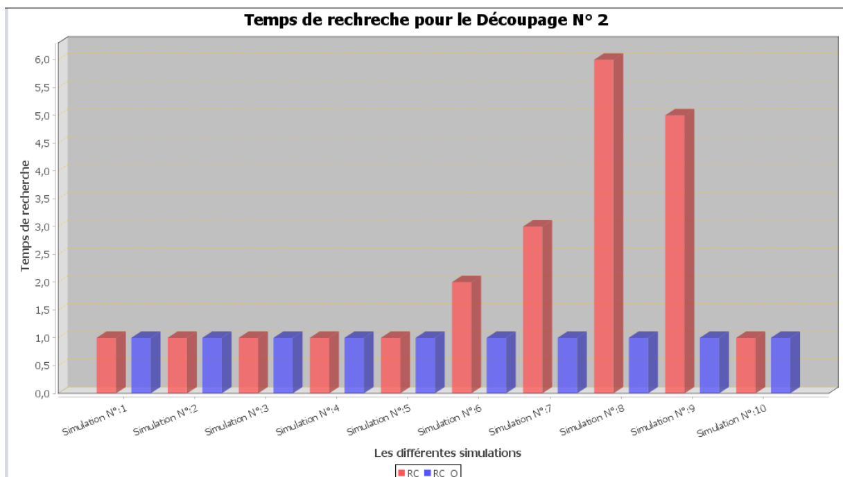
Figure III. 13: Temps de recherche pour le découpage N°2 (RC vs RC_Q)
