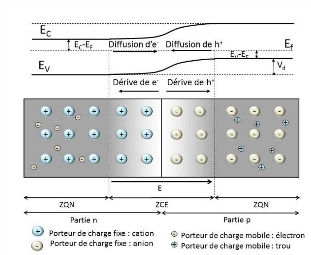
Figure I. 4 : Jonction p-n dans une cellule photovoltaïque.
