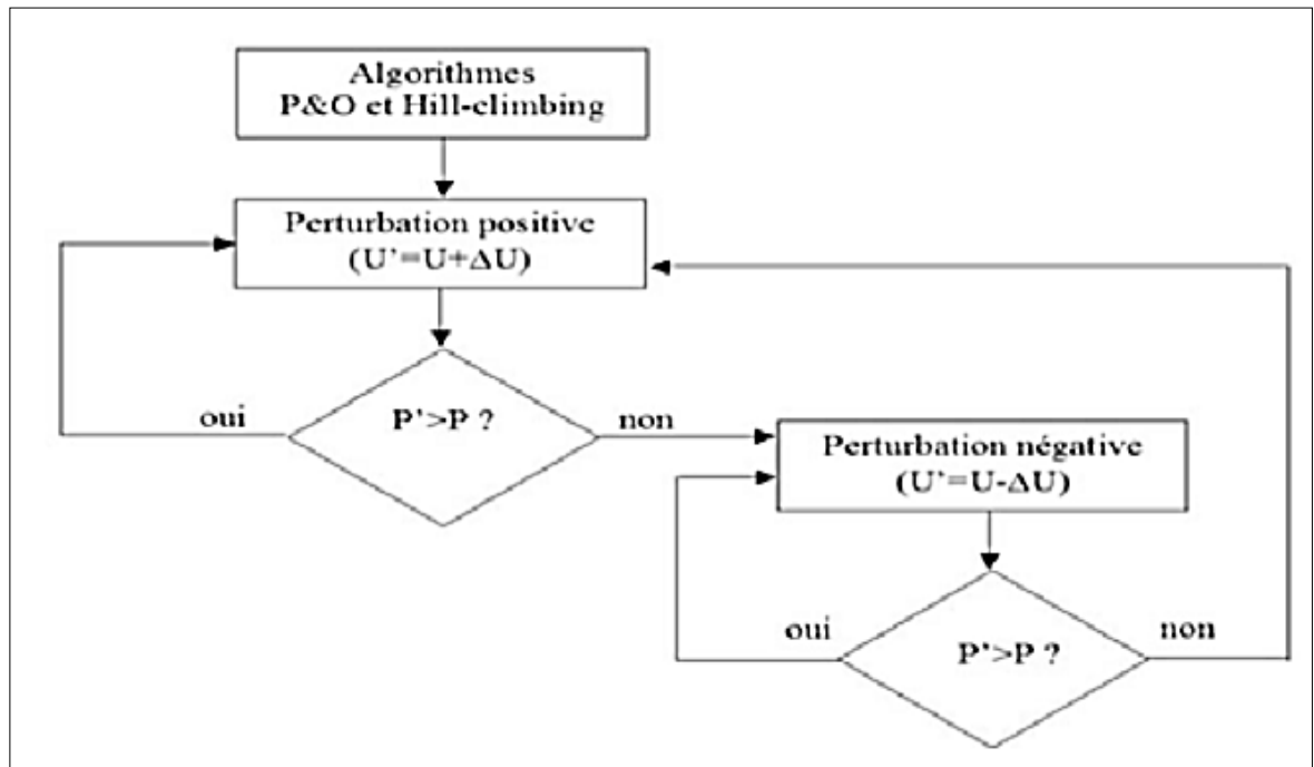
Figure II. 12: Principe d’algorithme de deux méthodes de Hill climbing et P&O
