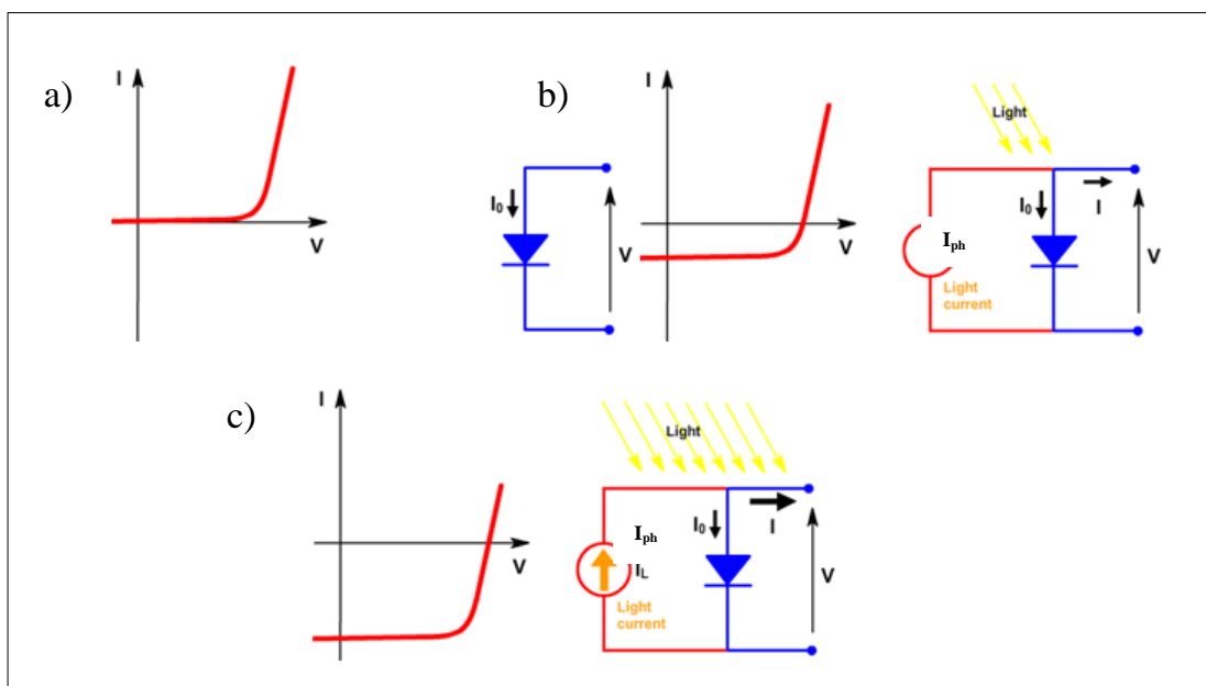
Figure I. 5 : Schéma équivalent de la cellule photovoltaïque à jonction PN
