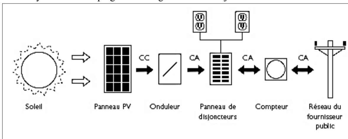
Figure II. 9: Agencement d'une installation PV raccordée au réseau.
