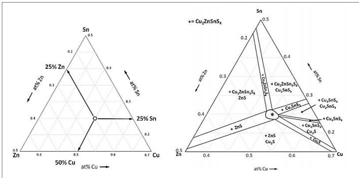
Figure V. 4 : Diagramme ternaire du CZTS pur
