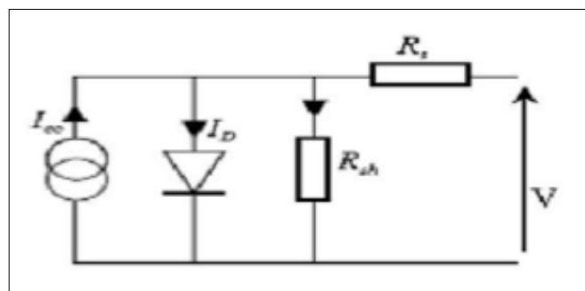
Figure I. 6:Circuit équivalent d'une cellule solaire
