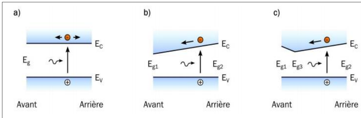
Figure V. 7: Principaux types de gradients de bande interdite rencontrés dans les couches de CIGS : a) Bandes plates, b) Simple gradient, c) Double gradient avec présence d'un notch [28].
