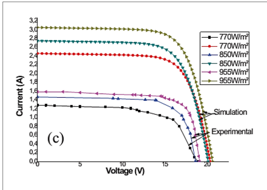
Figure III. 8: Superposition des caractéristiques J-V du panneau PV en fonction de l'éclairement à une température fixée à 45 °C
