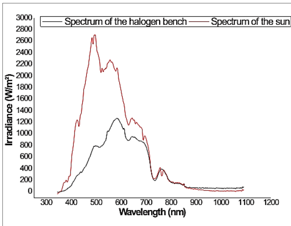
Figure III. 4: Distribution spectrale du soleil et du banc constitué de 6 lampes halogène mesuré en utilisant un détecteur de spectre K-MAC.
