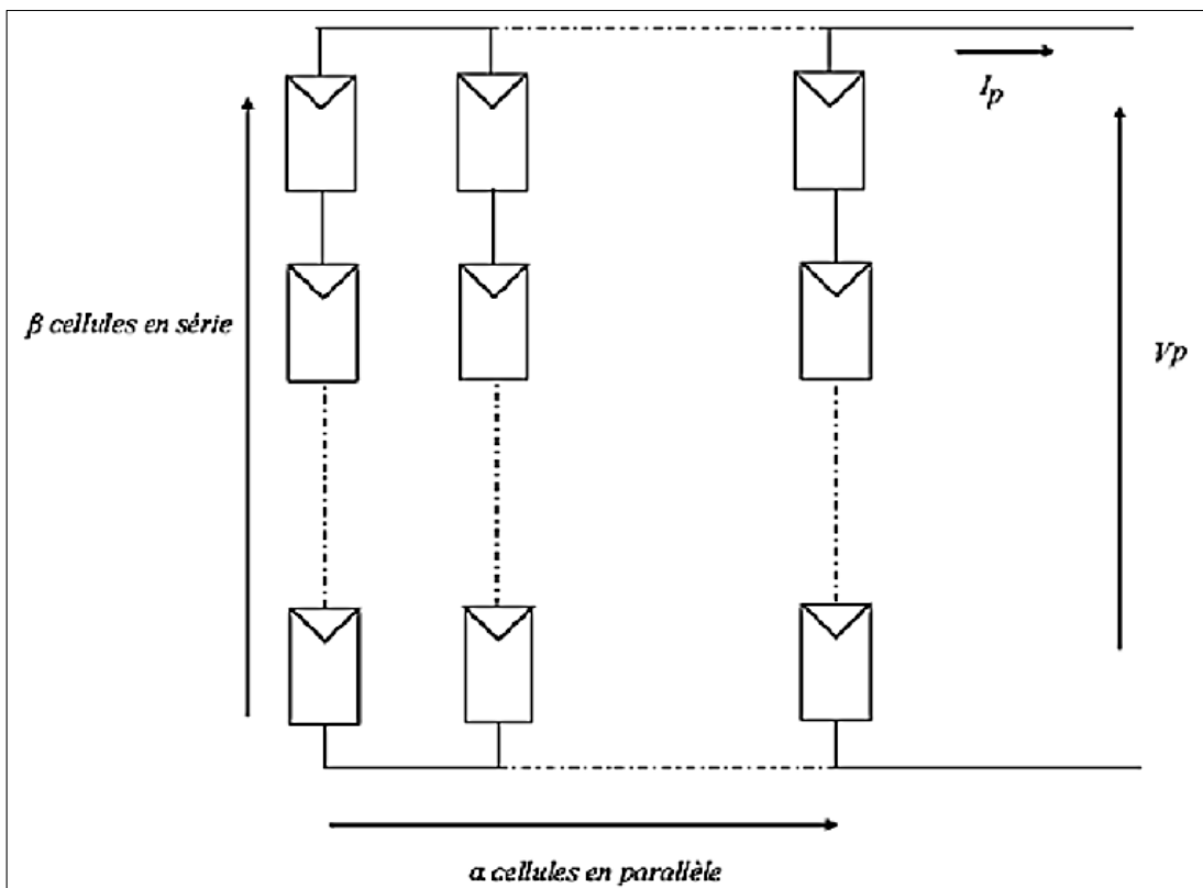
Figure II. 2: Association \alpha cellules en séries et \beta cellules en Parallèles
