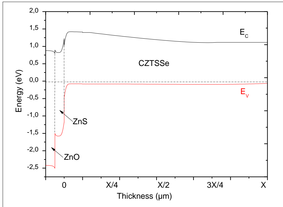
Figure VI. 8: Diagramme de bande de la cellule PV. (X = 0 correspondant à l'interface tampon / absorbeur).
