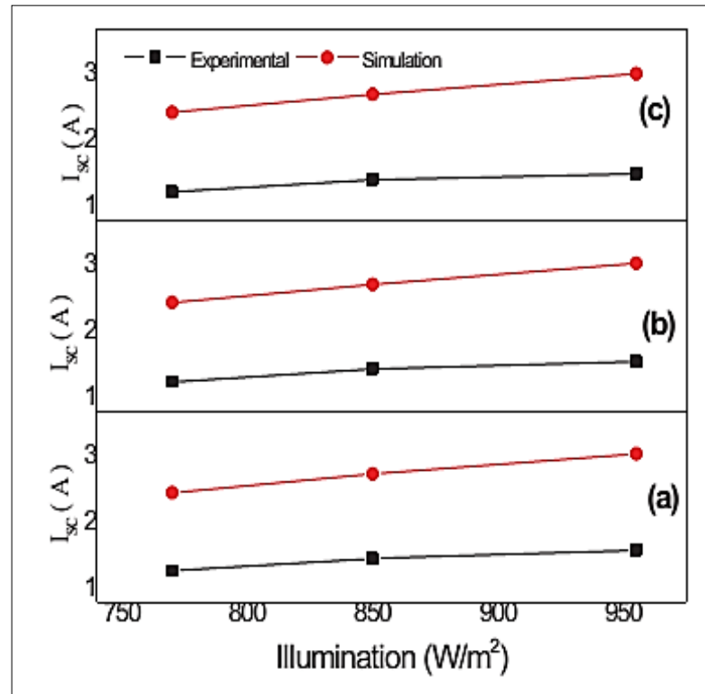
Figure III. 9: Comportement du courant de court-circuit ( J_{SC}=I_{SC} ) en fonction de l'éclairement à différentes températures.
