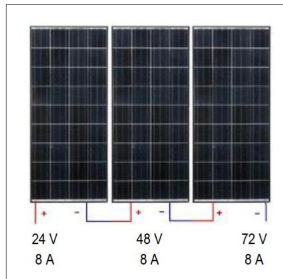
Figure II. 6: Assemblage en série des modules photovoltaïques
