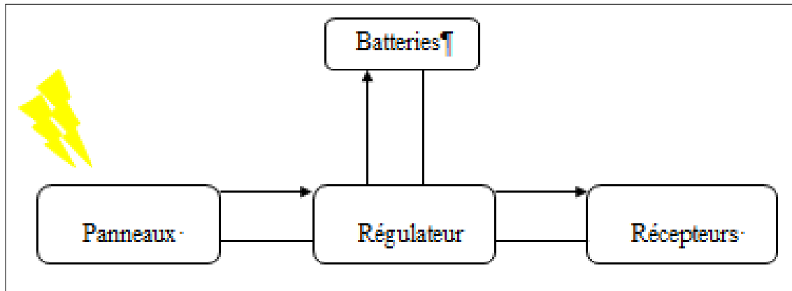
Figure II. 1 : la chaîne énergétique des constituants qui composent un générateur PV isolé.
