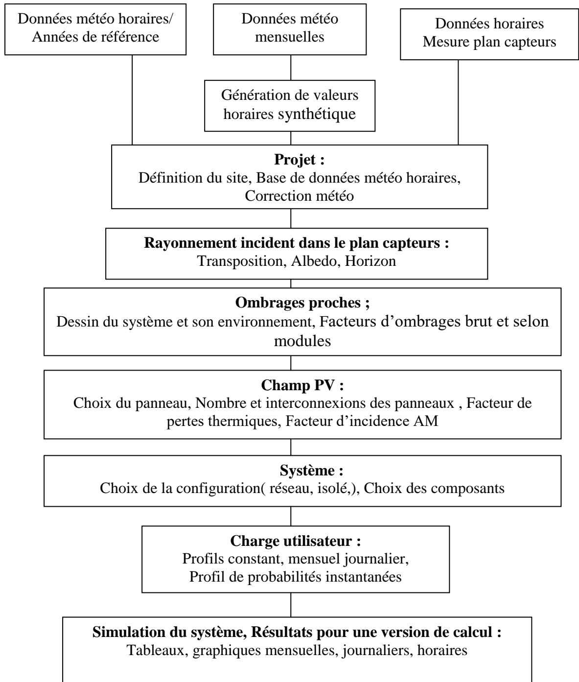
Figure IV. 2: Diagramme de principe du logiciel PVSyst. [1,2 et 3]
