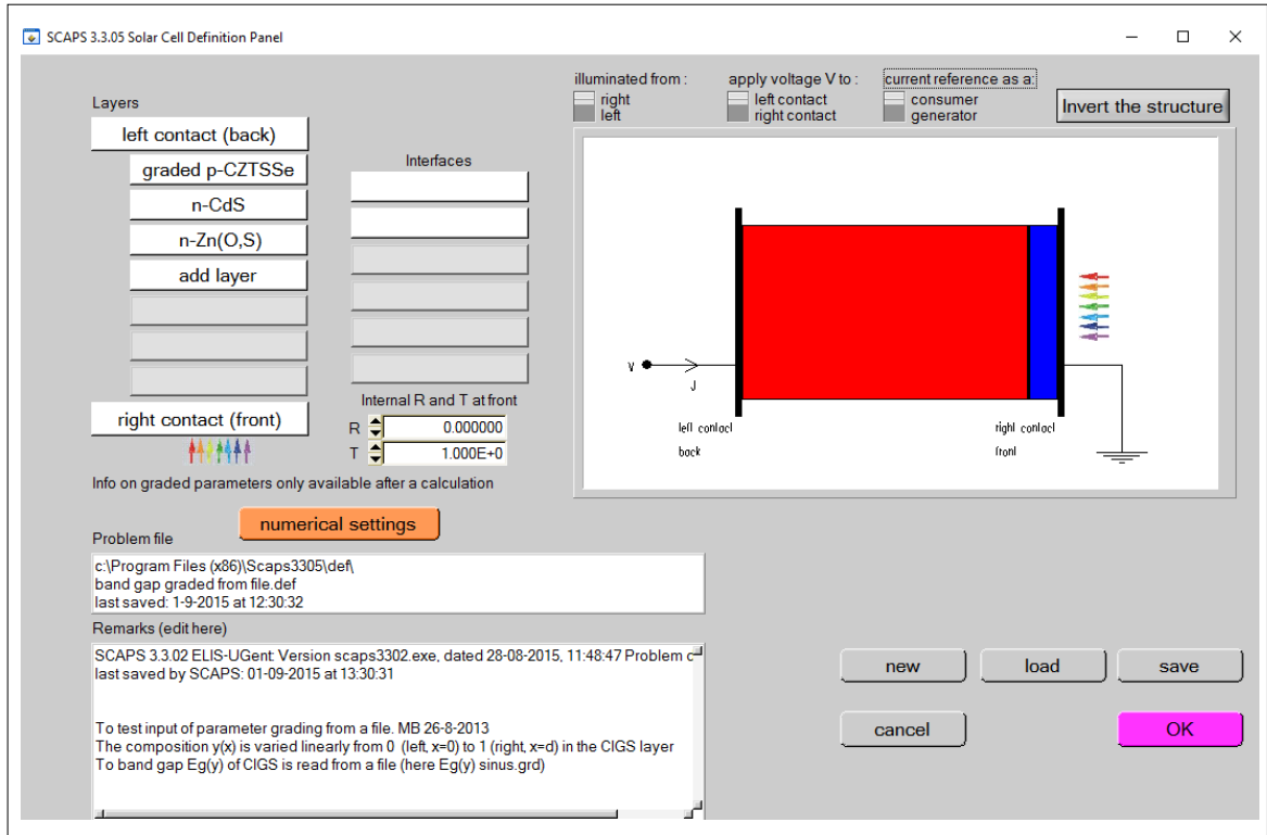
Figure VI. 2 : La page fenêtre de programme SCAPS.
