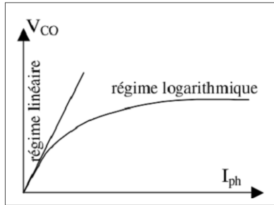
Figure I. 7 : Différents régimes selon la puissance d'éclairement.
