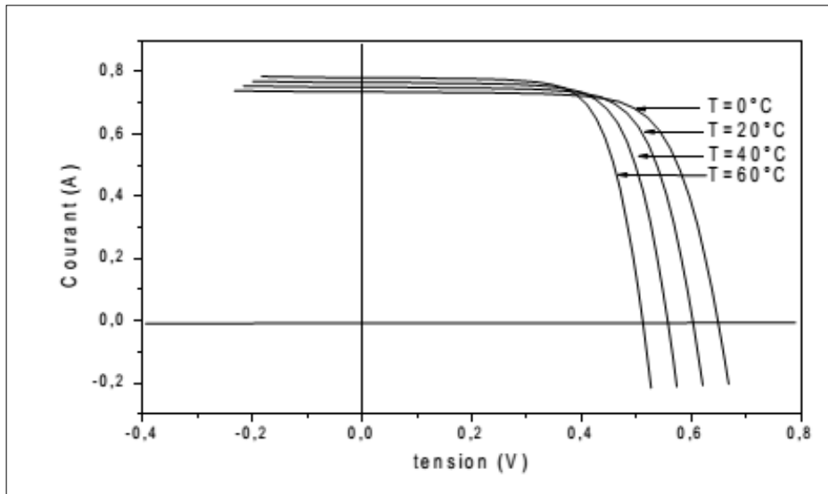
Figure I. 9 : Evolution de la caractéristique J(V) en fonction de la température.
