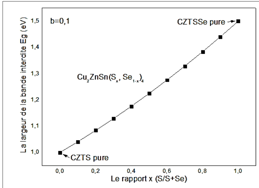
Figure V. 6: la variation de E_g en fonction de taux de composition ( x=S/(S+ Se) ).
