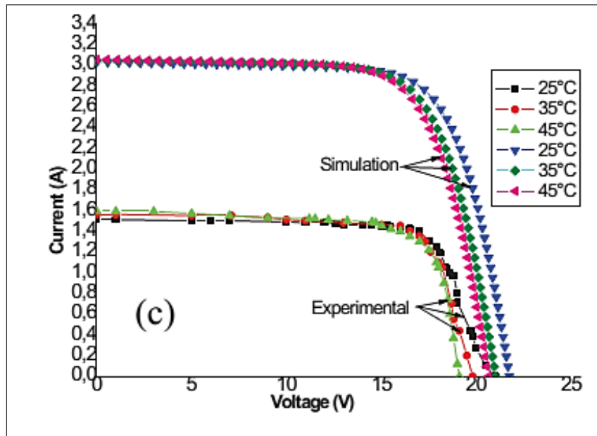
Figure III. 12: Caractéristiques J(V) d'un panneau en fonction de différentes températures où l'intensité de rayonnement égale à 955 \text{ W/m}^2
