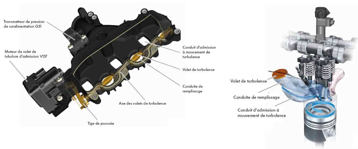
Figure I.18 La tubulure d'admission avec volets de turbulence (moteur TDI)
