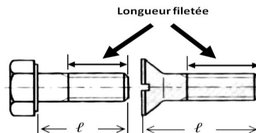
Figure II.2 : Longueur sous tête d'une vis
