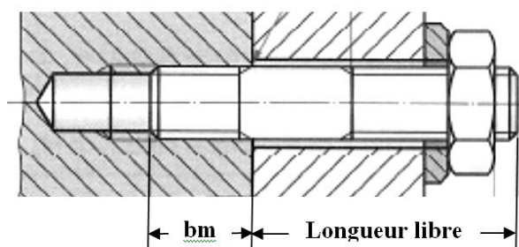
Figure II.6 : Implantation du goujon
