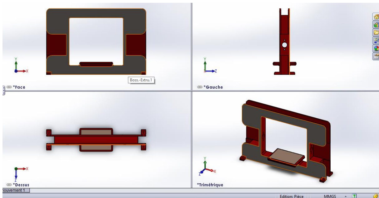
Figure III.3: mise en plan solidworks du banc d'essai en dimensions réelles
