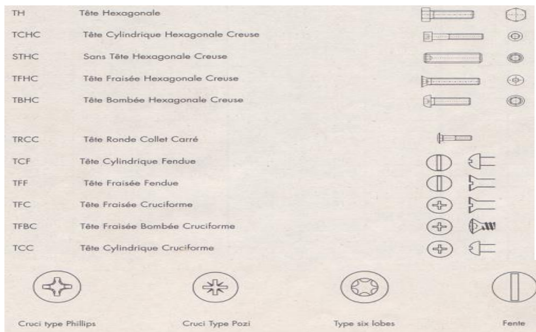
Figure I.3 : Les différents types de vis
