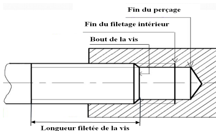
Figure II.5 : Montage d'une vis dans une pièce taraudée
