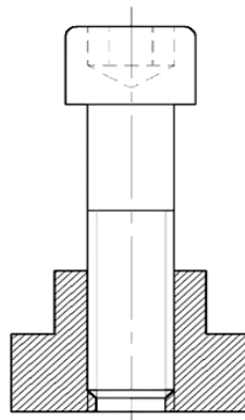
Figure II.4 Montage d'une vis CHC dans une pièce taraudée
