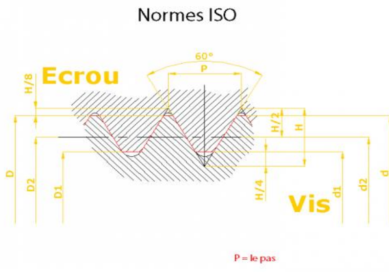
Figure I.2 : les normes ISO
