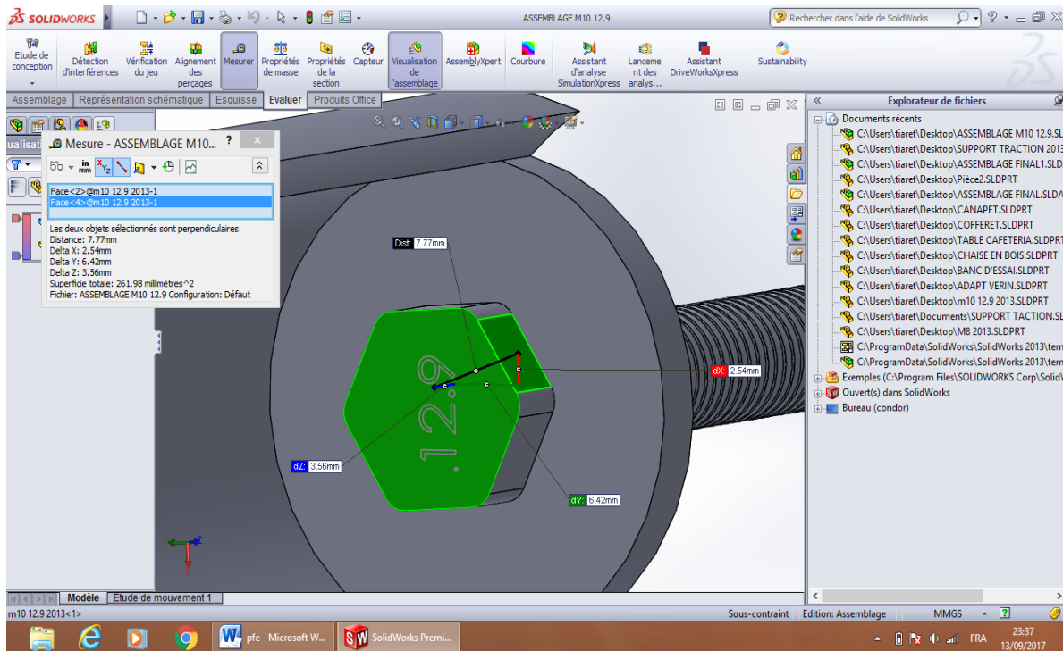
FigureIII.10 : Vue coté tête après fixation
