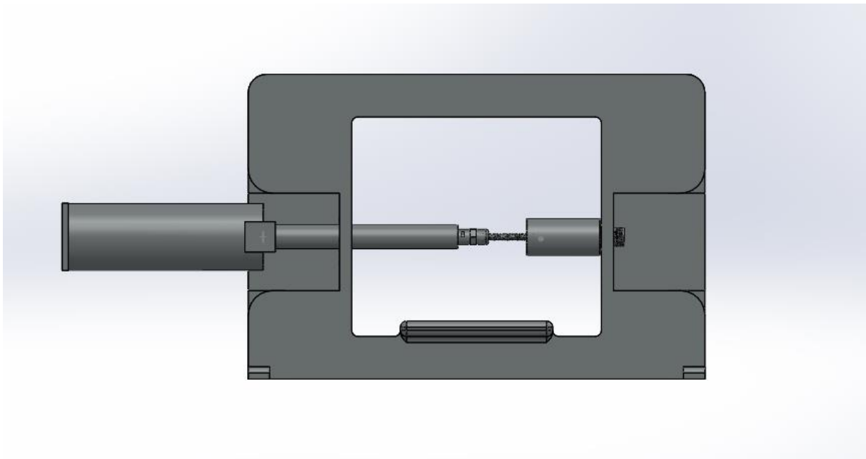
FigureIII.14 : Vue de face assemblage final
