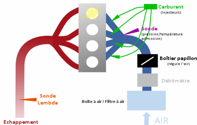
Figure II.47: Moteur essence moderne atmosphérique injection indirecte
