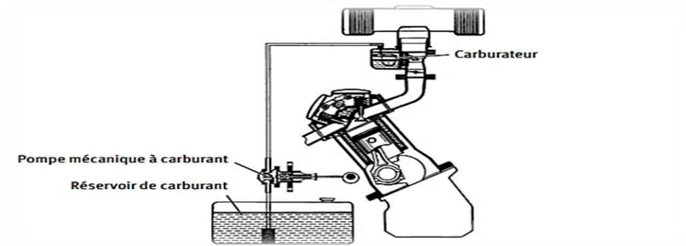
Figure II.19 : Alimentation en carburant d'un moteur à carburateur (jusqu'à env. 1976)
