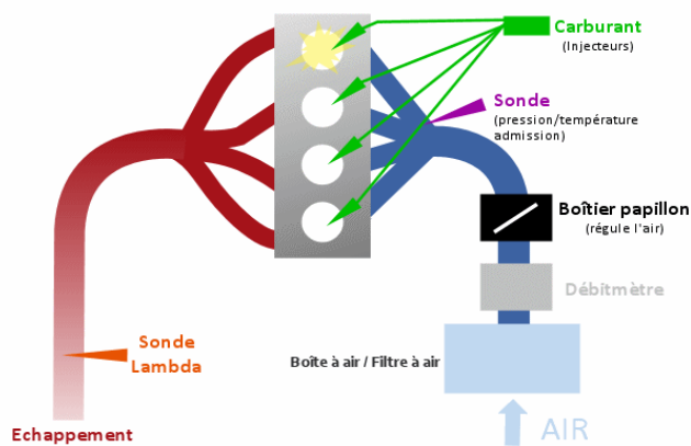
Figure II.48: Moteur essence moderne atmosphérique injection directe
