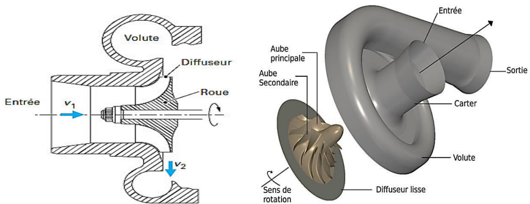
Figure III.14 : schéma Compresseur centrifuge
