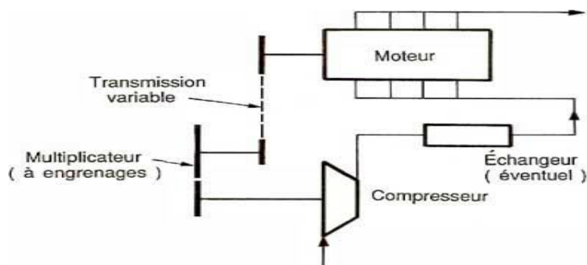
Figure III.2: Schéma d'installation d'un moteur suralimenté par compresseur centrifuge
