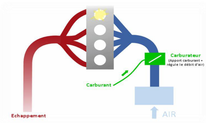
Figure II.45: circuit d'ancienne moteur essence atmosphérique à carburateur
