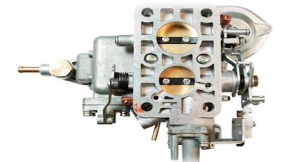
Figure II.31 : carburateur
