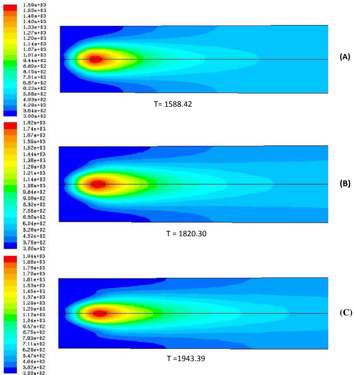
Figure IV.3 : influence de pression sur la température de flamme
