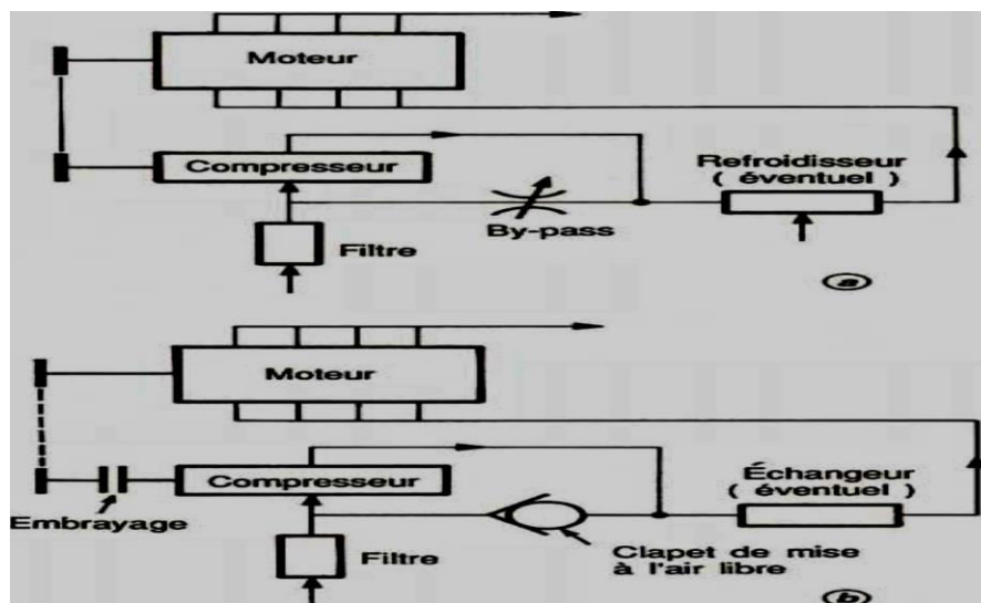
Figure III.1 Schémas d'installation d'un moteur suralimenté par compresseur volumétrique
