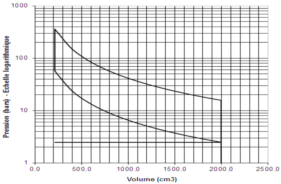
Figure IV.12 cycle de beau de rochas pour une pression P=2.5 bar
