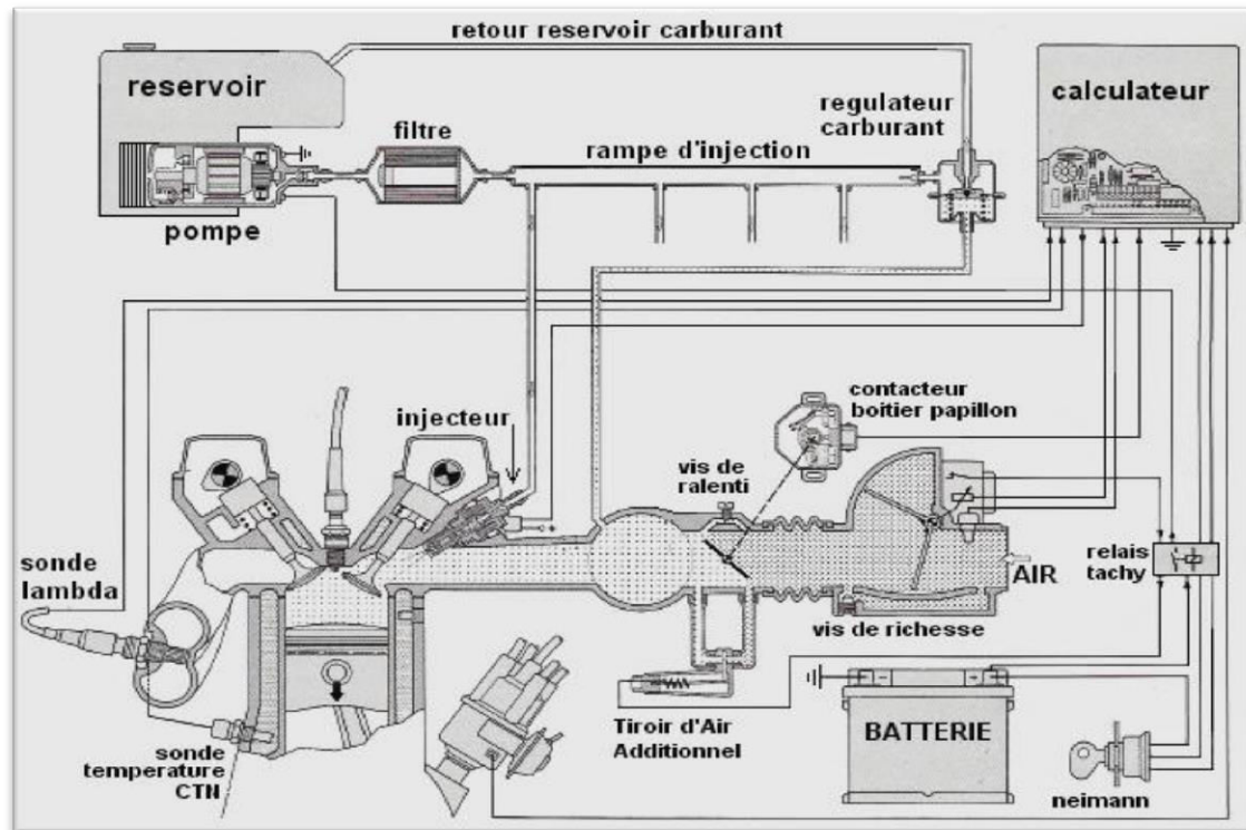
Figure II.39 : Schéma du système L-Jetronic
