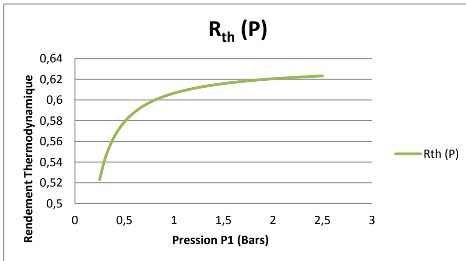
Figure IV.17 : Le rendement Thermodynamique
