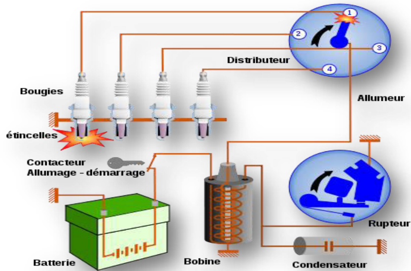
Figure II.15 : L'allumage par batterie
