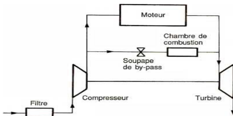
Figure III.3:Schéma d'installation d'un moteur suralimenté
