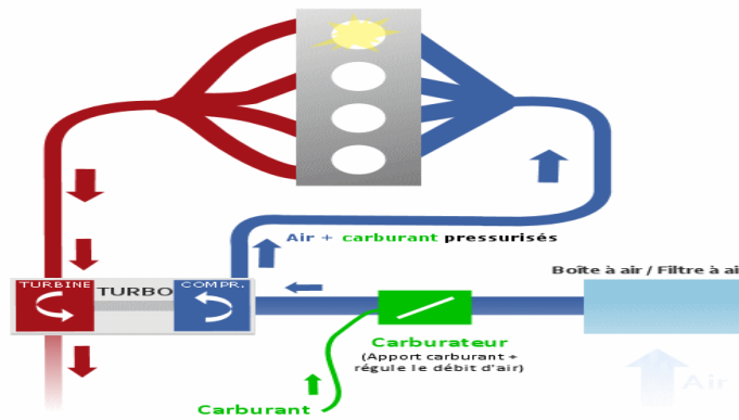
Figure II.46: Ancien moteur essence turbo à carburateur
