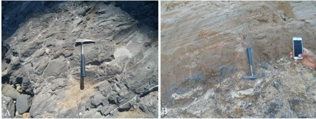
Figure.20 : A affleurement de la 1 ère coulée, b affleurement de la partie scoriacée
