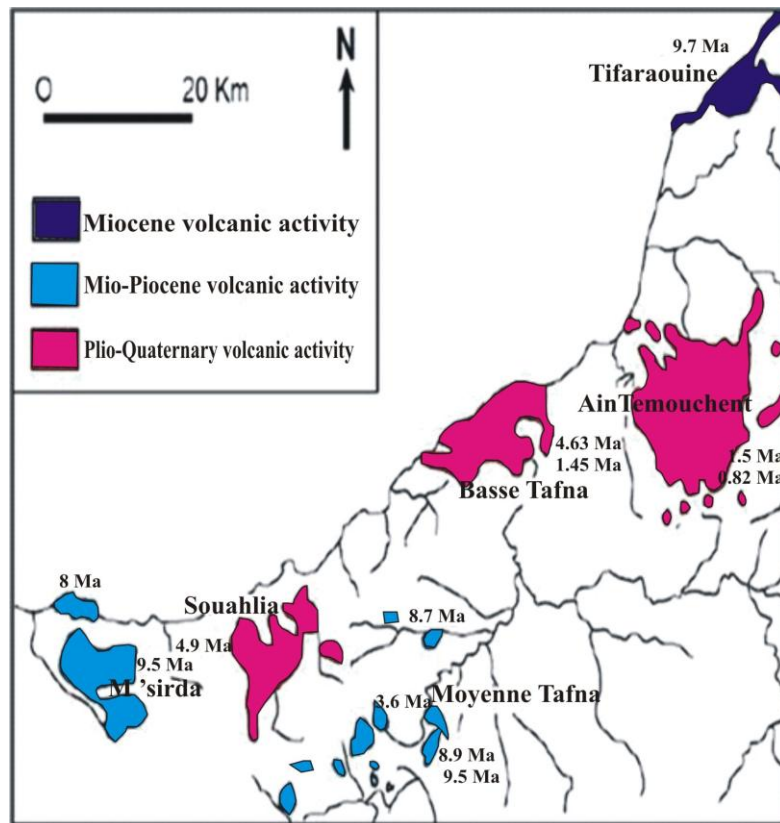
Fig.4. Localisation et âge du volcanisme Mio-Plio-Quaternaire de l'Algérie Nord-occidentale (Megartsi, 1985).modifie
