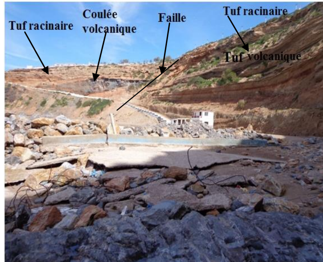
Figure.26 : vue panoramique de la 4 ème coulée
