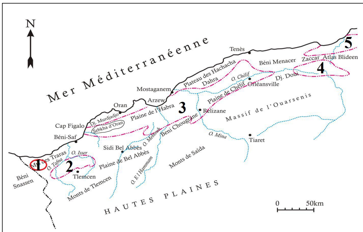
Fig.1 : Esquisse géographique des bassins néogènes sublittoraux de l'Algérie occidentale (D'après Perrodon, 1957 ; modifiée)
