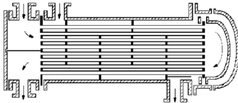
Figure 2.34. Refroidisseur d'huile
