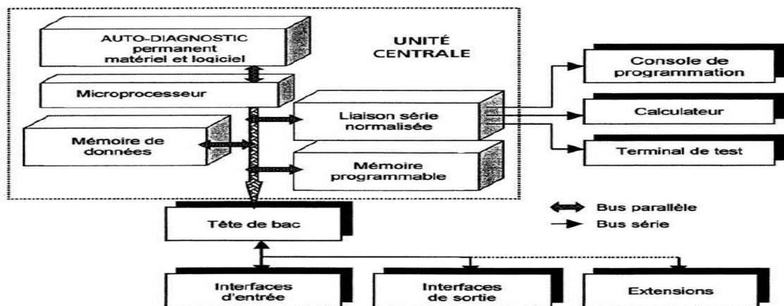
Figure 2.11. Structure de l'automate programmable de la presse MTRIX HS 550L
