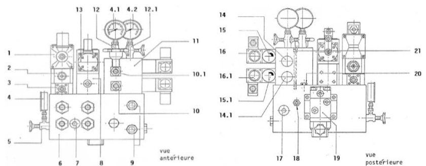
Figure 2.16. Bloc DHK tiroir
