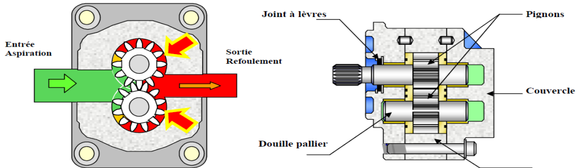
Figure 2.25. Pompe à engrenage à denture extérieure [5].
