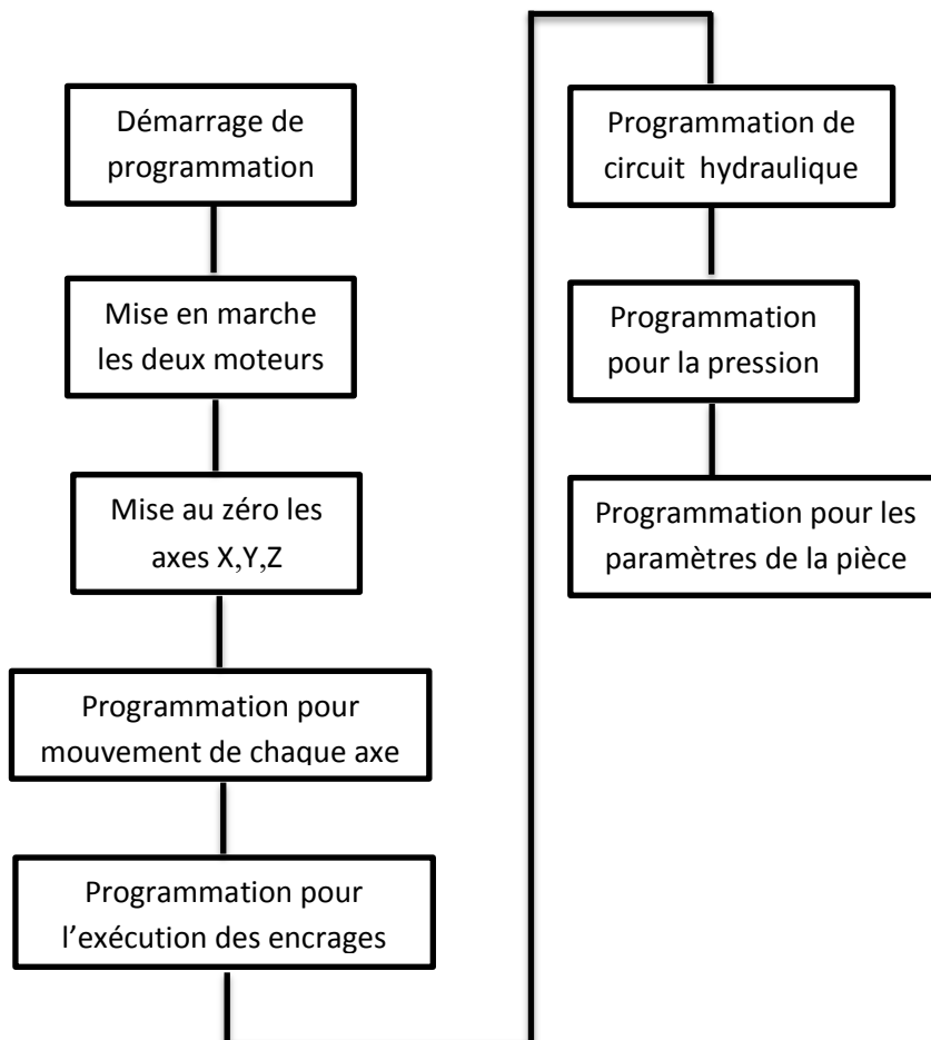
Figure 2.15. Organigramme présente les programmes de la presse
