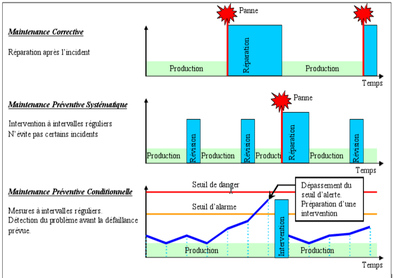
Figure 3.3. Comparaison entre les types de maintenance [10].
