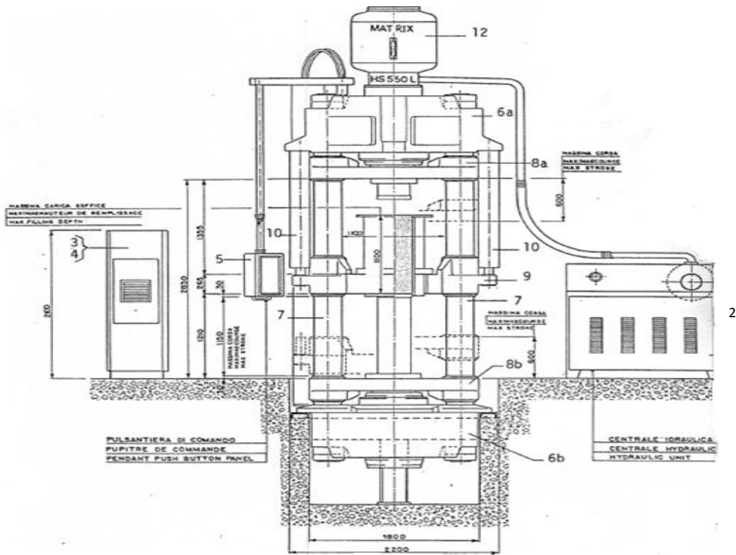
Figure 2.3. Vue de face de la presse MATRIX HS 550L [3].
