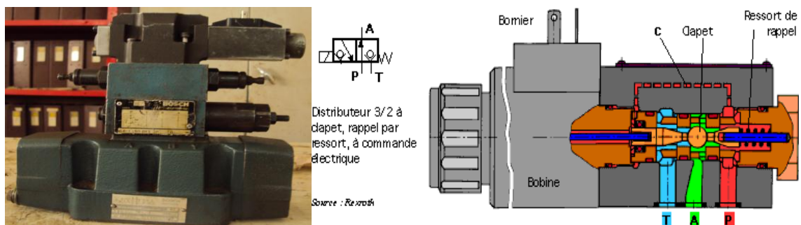
Figure 2.31. Distributeur à clapet commande électrique
