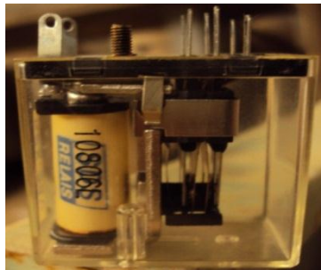
Figure 3.10. Un relai de la presse
