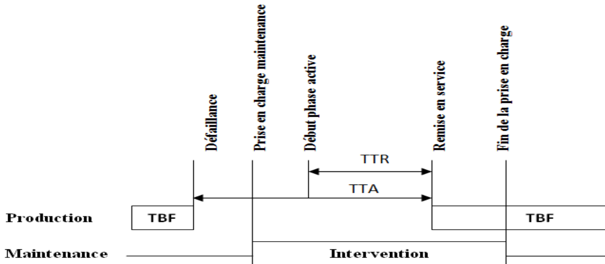
Figure 3.1. Temps caractéristiques lors d'une intervention [9].
