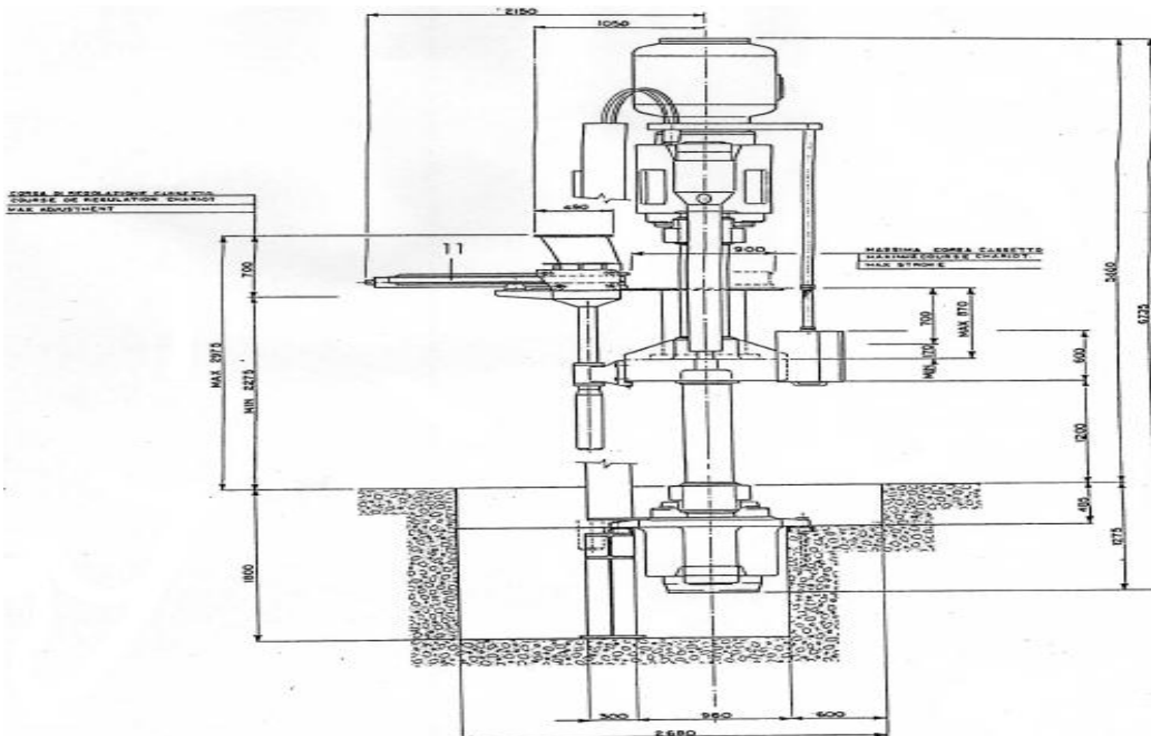
Figure 2.3. Vue de face de la presse MATRIX HS 550L [3].
