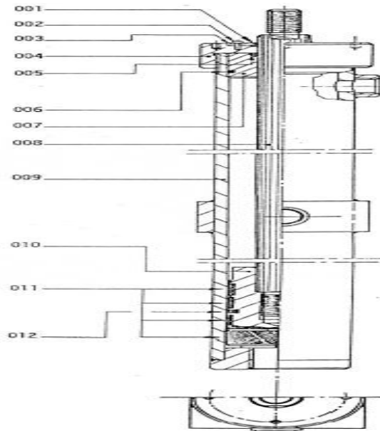
Figure 4.4. Vérin hydraulique de chariot de chargement [3].
