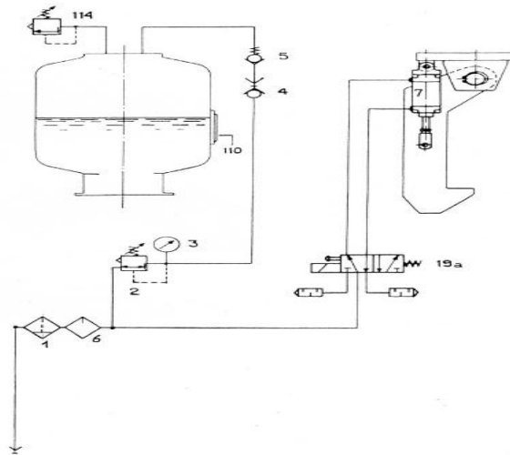
Figure 10. Schéma pneumatique
