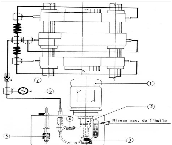
Figure 2.35. Lubrification centralisée [3].
