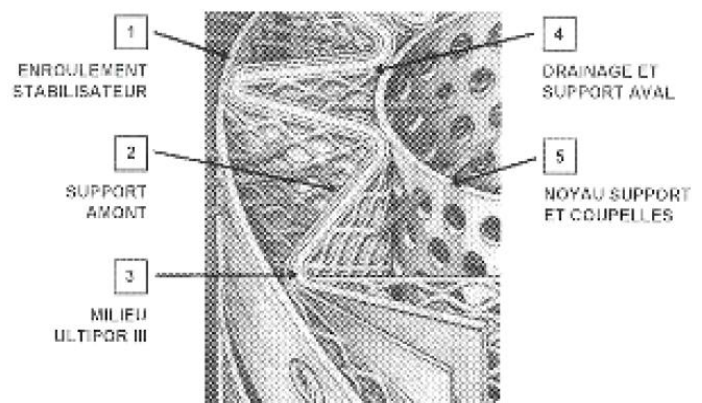
Figure 2.23. Constitution d'un filtre [5].
