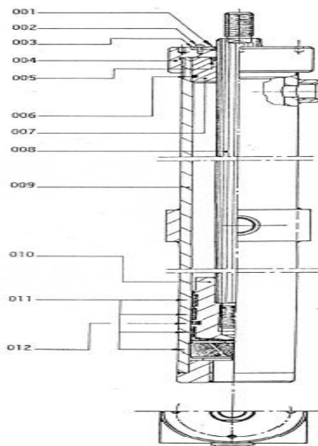
Figure 3. Vérin hydraulique de la presse
