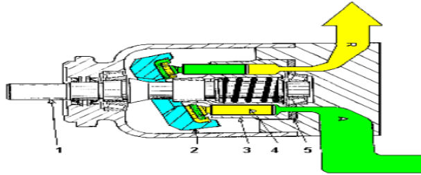
Figure 2.24. Pompe à piston à débit variable [6].
