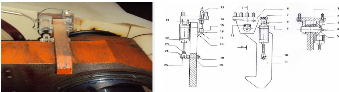
Figure 2.36. Ancrage de sécurité
