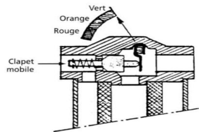
Figure 4.1. Indicateur de colmatage [4].
