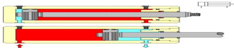
Figure 2.28. Vérin à double effet [6].
