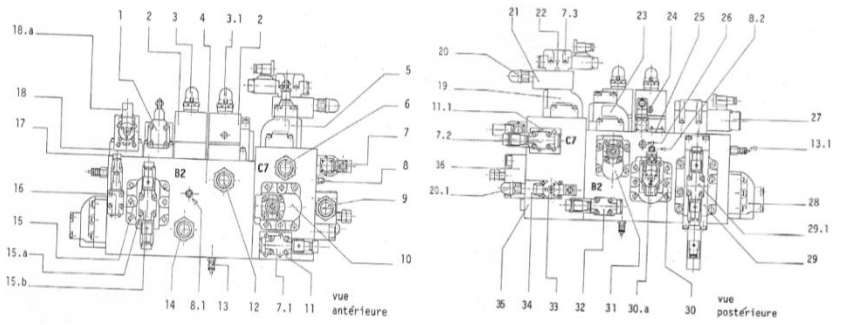
Figure 2.18. Bloc « B2 » et bloc « C7 »
