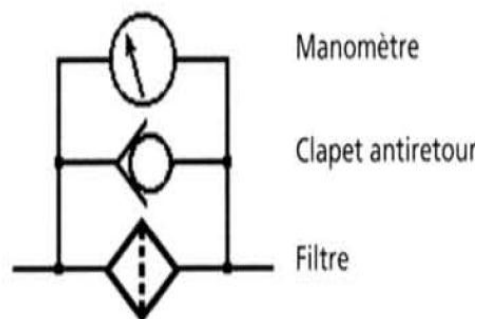
Figure 4.2. Manomètre différentiel [4].
