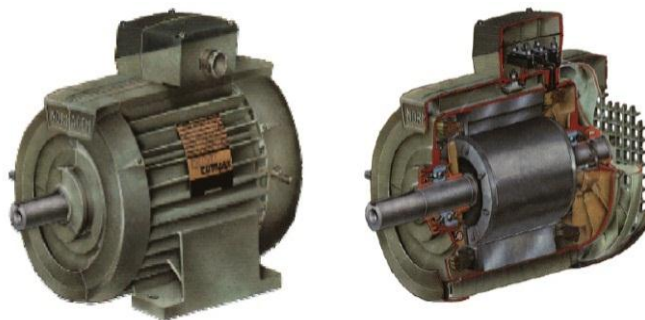
Figure 2.30. Moteur électrique triphasé
