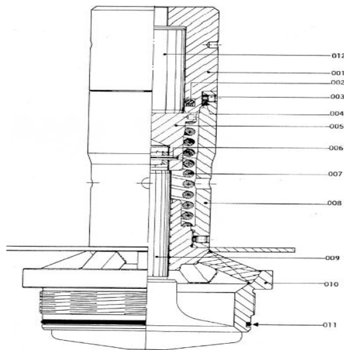
Figure 4. Soupape de remplissage rapide
