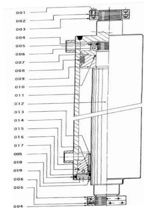
Figure 2. Vérin d'extraction
