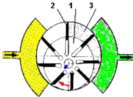
Figure 2.26. Pompe à palette [5].
