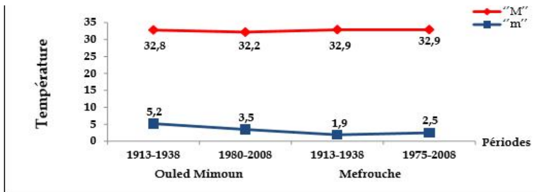
Figure 13: Températures moyennes des minima du mois le plus froid et Températures moyennes des maxima du mois le plus chaud
