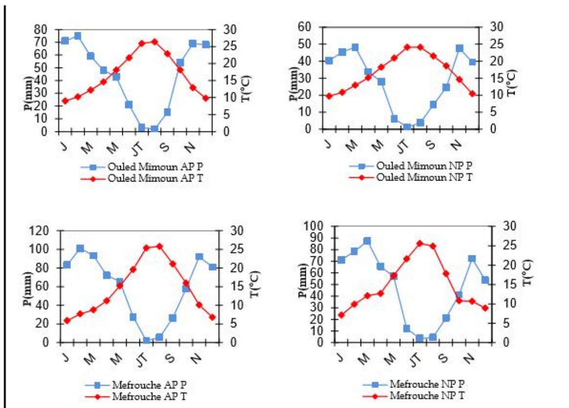
Figure 14: Diagrammes ombrothermiques de Bagnouls et Gausson
