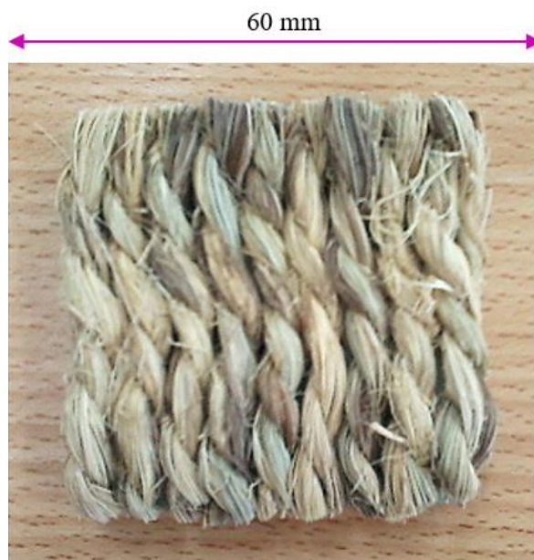
Figure 3.10 Photo type des fibres d'alfa tressées collées sur le support de cisaillement
