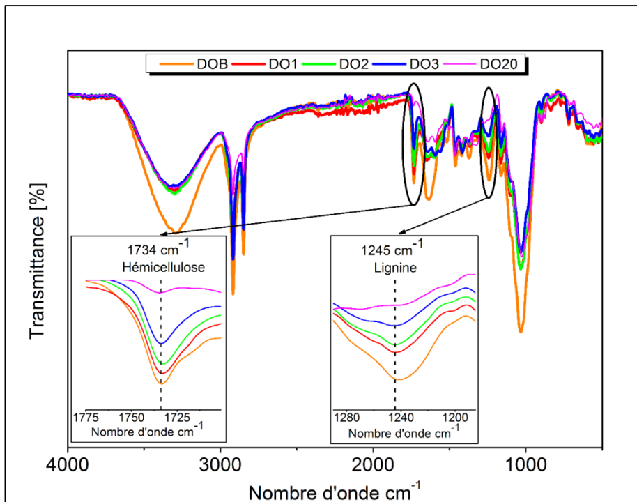
Figure 4.2 : Spectre infrarouge des fibres de Doum brutes et traitées.
