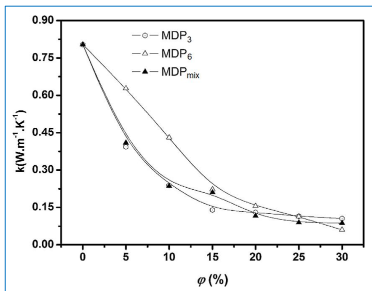
Figure 2.13 : Conductivité thermique des mortiers cimentaires renforcés par des fibres de palmier dattier de 3 mm (MDP3), 6 mm (MDP6) et le mélange de deux diamètres (MDPmix) [BEN 14].
