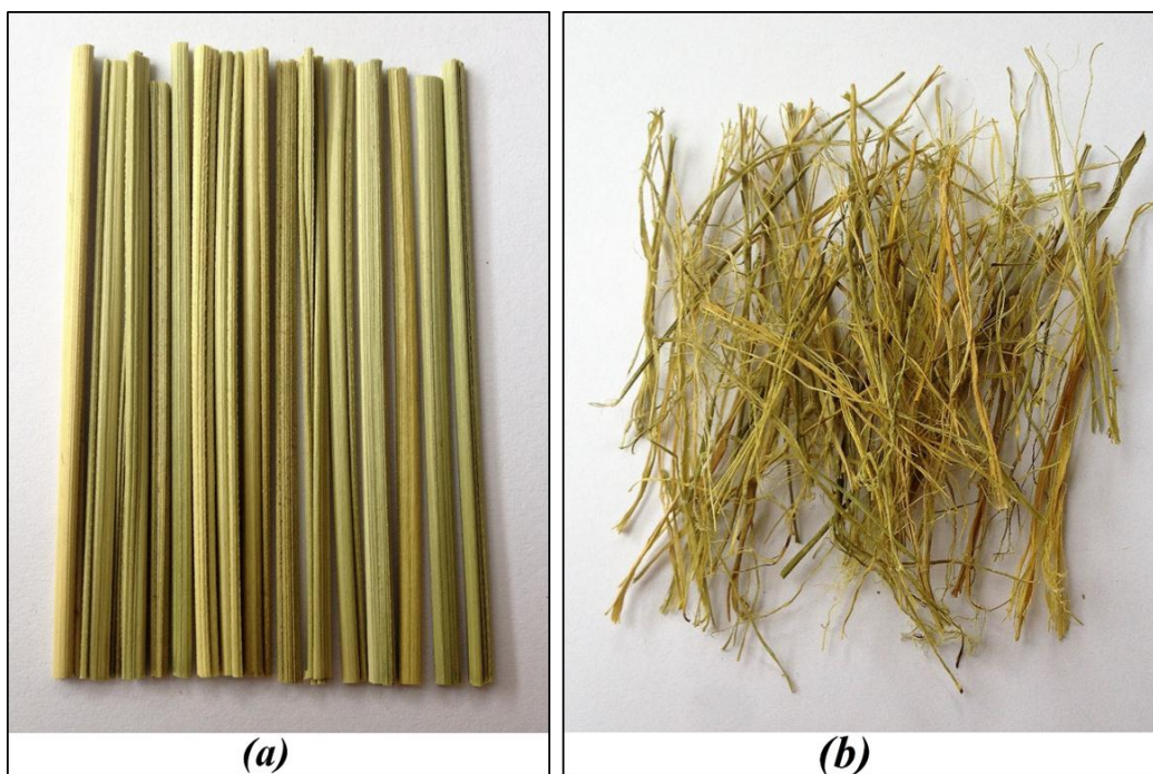
Figure 3.5 : Fibres de Diss (a) brutes et (b) traitées à forte concentration de NaOH.
