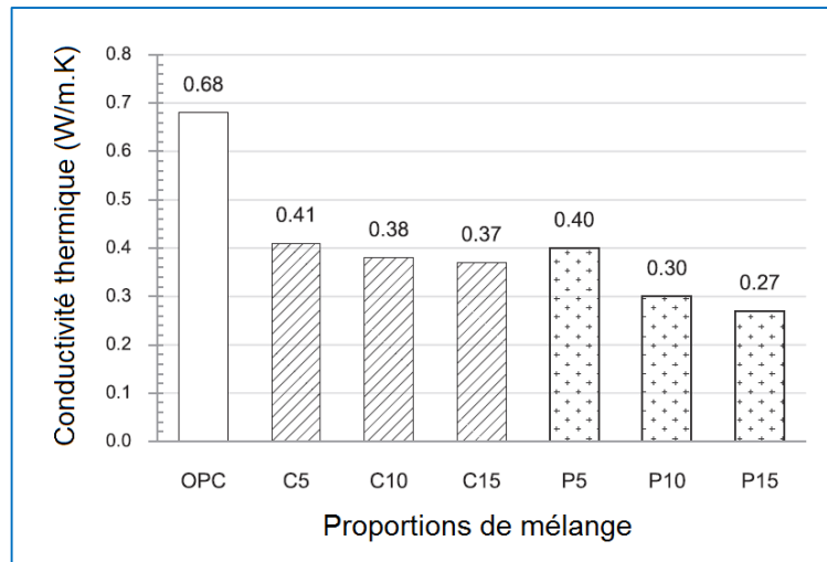
Figure 2.12 : Conductivité thermique des mortiers renforcés avec les fibres végétales de la noix de coco (C(X)) et du palmier à huile (P(X)) [LER 15].
