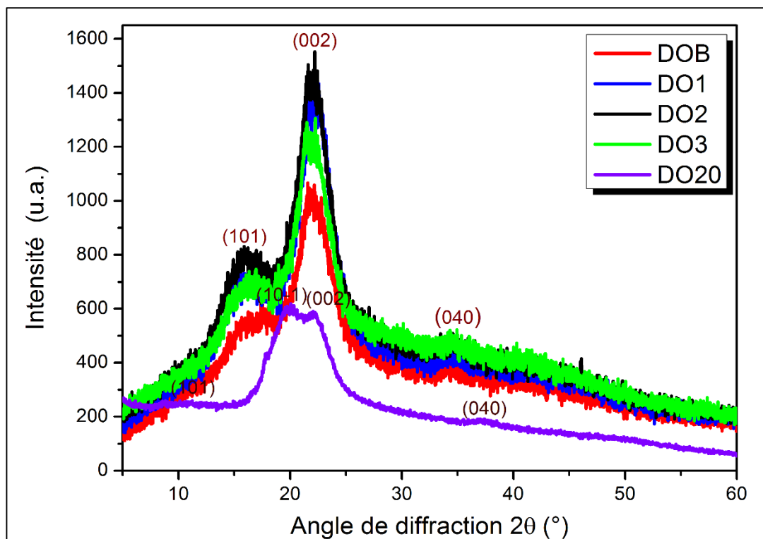
Figure 4.4 : Diffractogrammes des fibres de Doum brutes et traitées.
