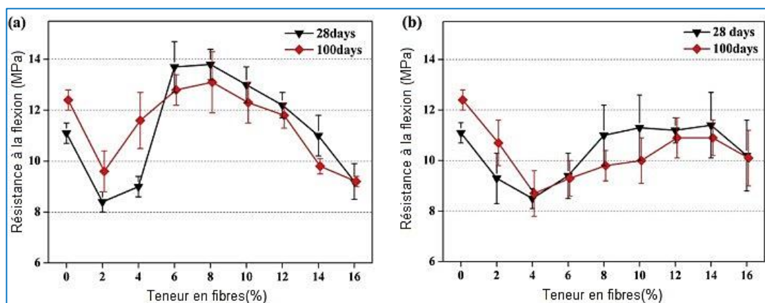
Figure 2.8 : Résistances à la flexion en fonction de la teneur en fibres pour les composites renforcés avec : (a) fibres de riz et (b) fibres de bambou à 28 et 100 jours.
