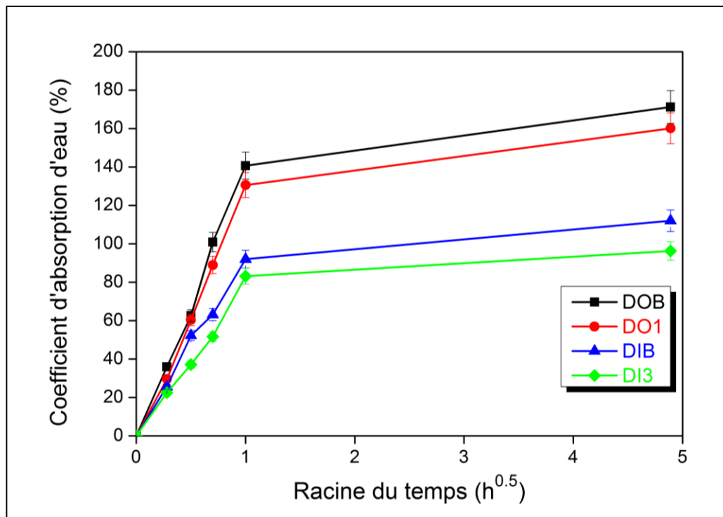
Figure 4.7 : Cinétique d'absorption de l'eau des fibres végétales de Doum (brutes et traitées à 1% de NaOH) et de Diss (brutes et traitées à 3% de NaOH).
