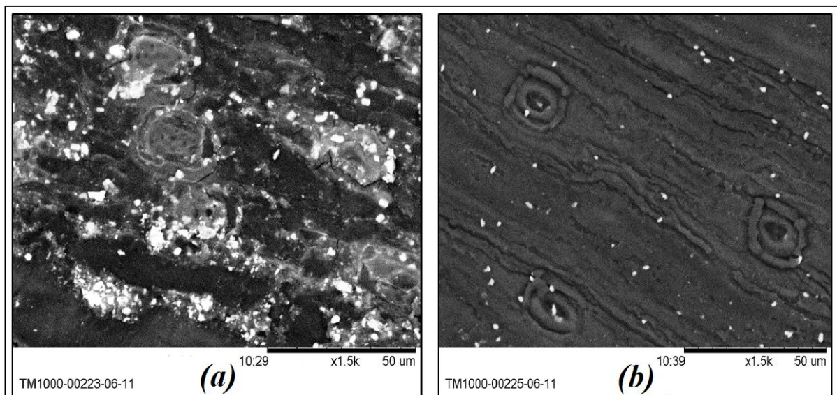
Figure 4.5 : Micrographie de la fibre de Doum : (a) brute et (b) traitée avec 1% de NaOH.
