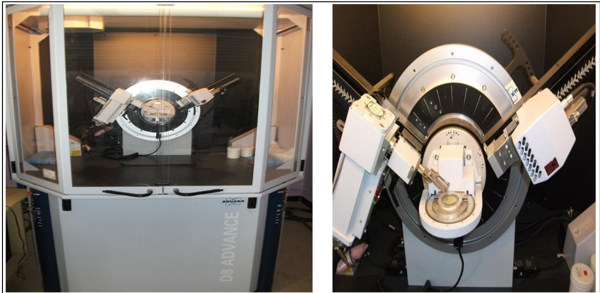
Figure 3.9 : Diffractomètre à rayons X type Bruker AXS D8 Advance (Laboratoire de Chimie Des Polymères-LCP-Université d'Oran, Algérie).
