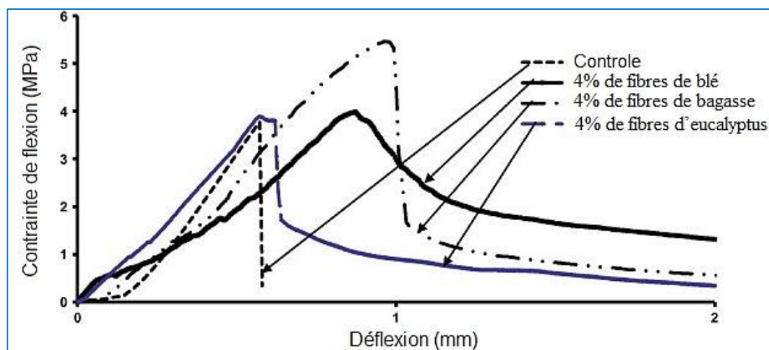
Figure 2.10 : Résistances à la flexion des composites renforcés avec 4% de fibres végétales comparativement aux échantillons de référence.
