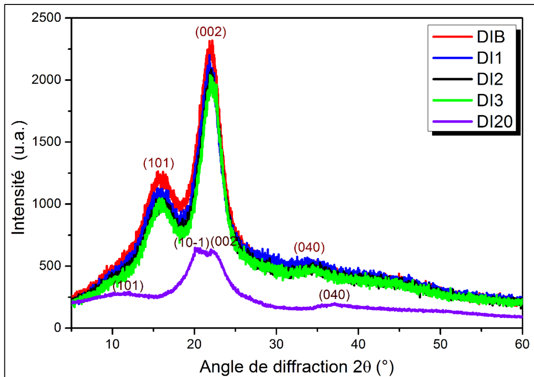
Figure 4.3 : Diffractogrammes des fibres de Diss brutes et traitées.
