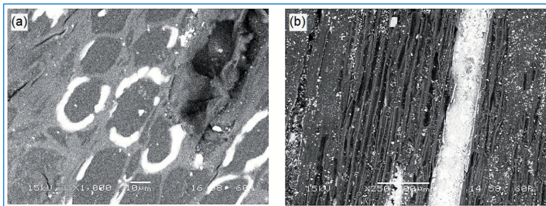
Figure 2.18 : Observations au MEB en vide partiel en mode électrons rétrodiffusés (a) d'une section transversale (x1000) et (b) longitudinale (x250) de chènevotte extraite d'un composite âgé de 2 ans et demi [MAG 11].
