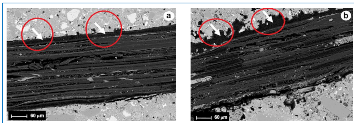
Figures 2.15 : Images des électrons rétrodiffusés (BSE) de l'interface entre la fibre et la matrice des tuiles âgées de 14 ans : (a) conservées aux conditions du laboratoire et (b) en vieillissement naturel [TON 11].
