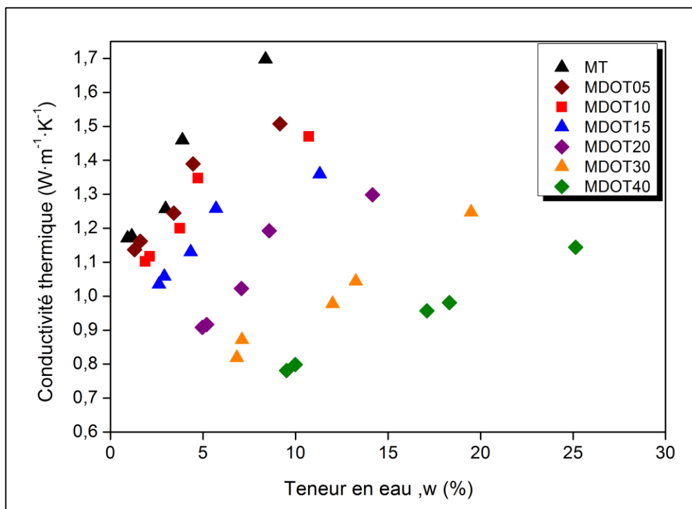
Figure 4.19 : Variation de la conductivité thermique des mortiers renforcés de fibres de Doum traitées en fonction de la teneur en eau.
