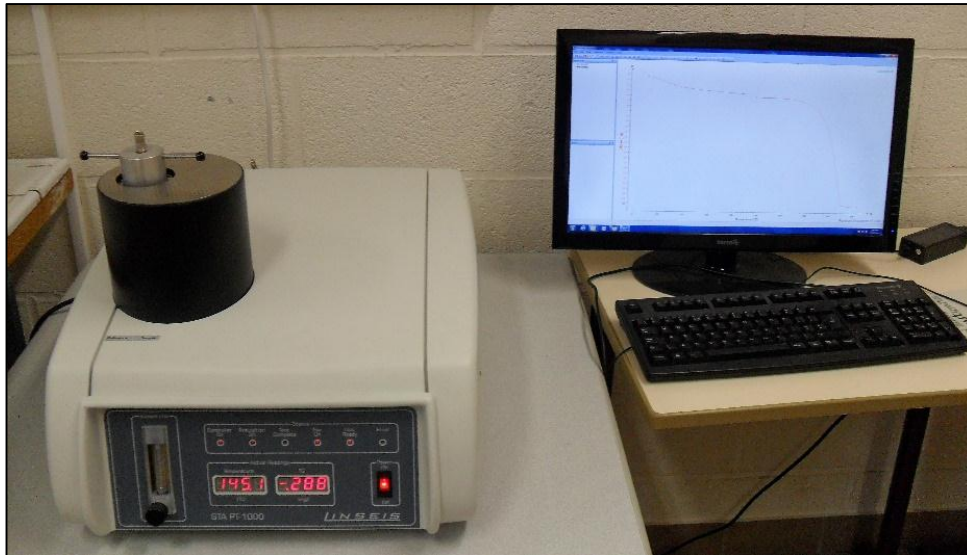
Figure 3.16 : Analyseur thermogravimétrique (TGA / DSC, LINSEIS STA PT1000) (Laboratoire PRISME, Polytech'Orléans, Université d'Orléans, France).
