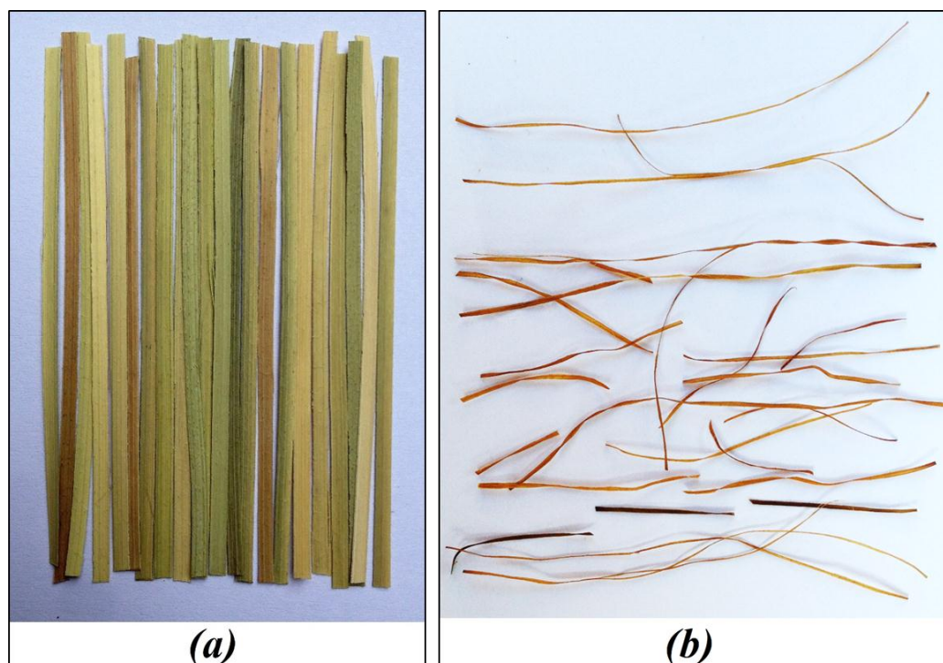
Figure 3.6 : Fibres de Doum (a) brutes et (b) traitées à forte concentration de NaOH.
