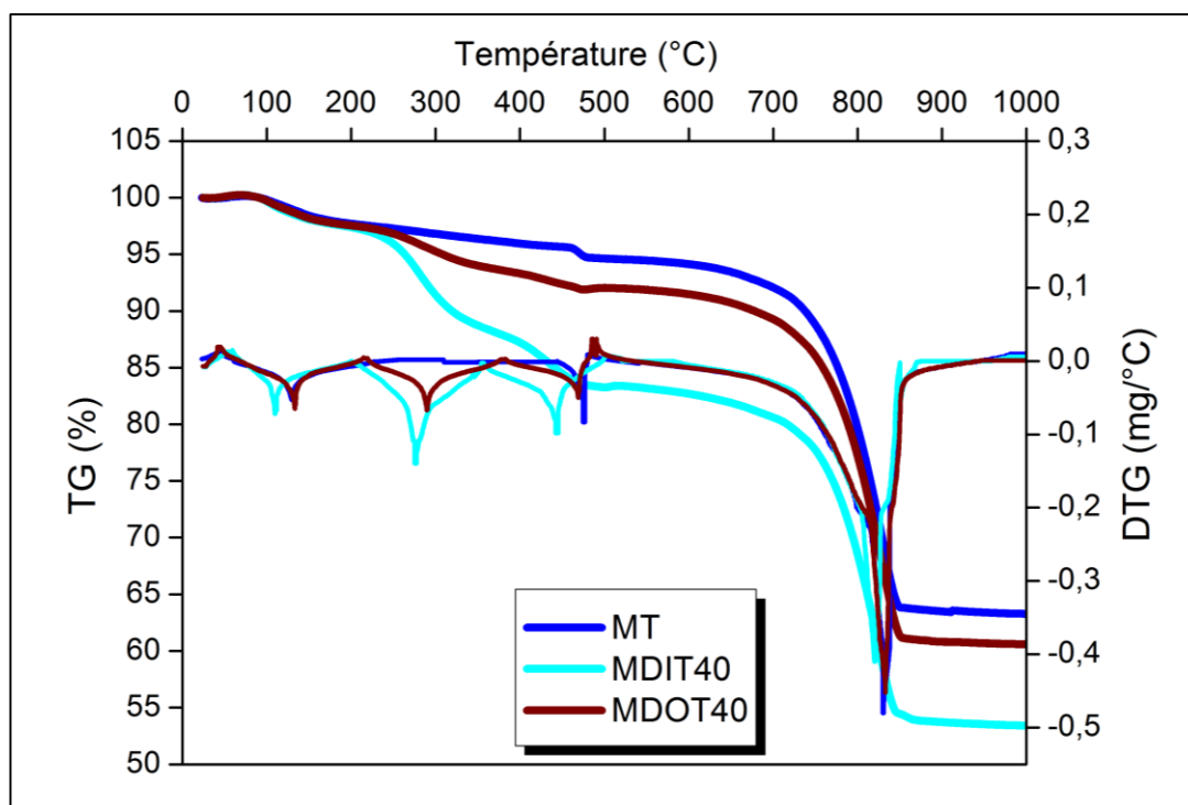
Figure 4.21 : Évolutions de TG et DTG en fonction de la température pour les composites à base de 4% de fibres de Diss et de Doum.
