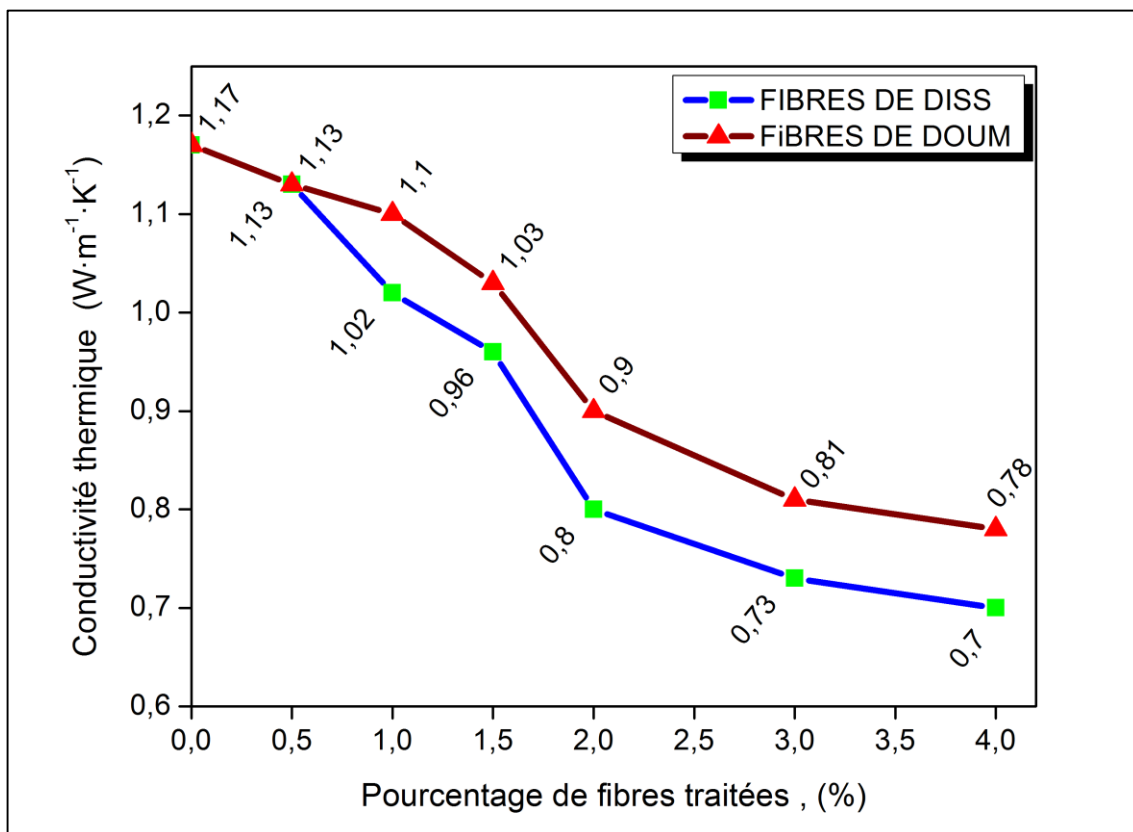
Figure 4.17 : Evolution de la conductivité thermique en fonction de la teneur en fibres après 192h de séchage.
