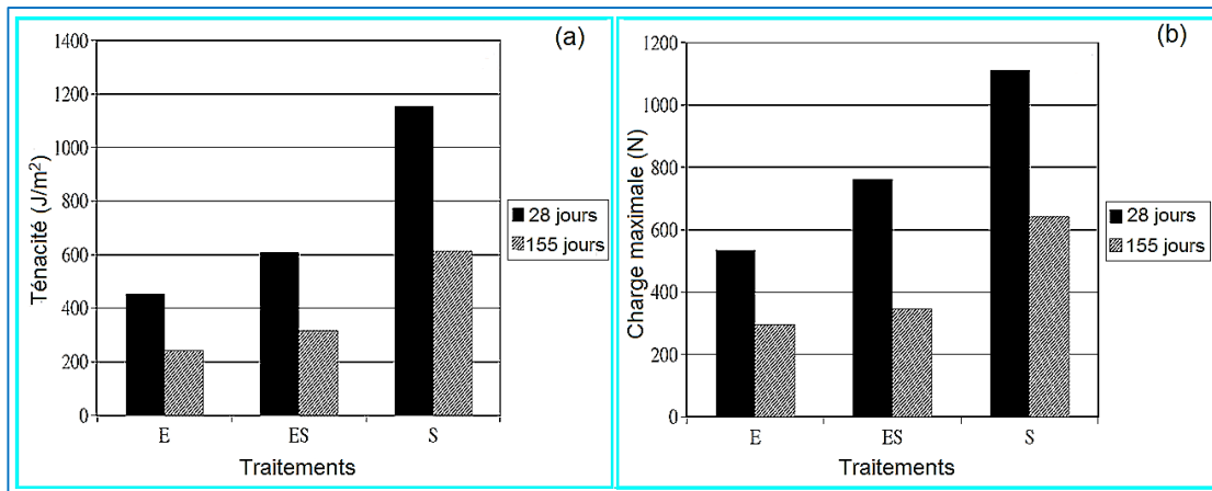
Figure 2.17 : (a) la ténacité, (b) la rigidité des carreaux de tuiles renforcés avec les fibres végétales pour différents âges et traitements [ROM 08].
