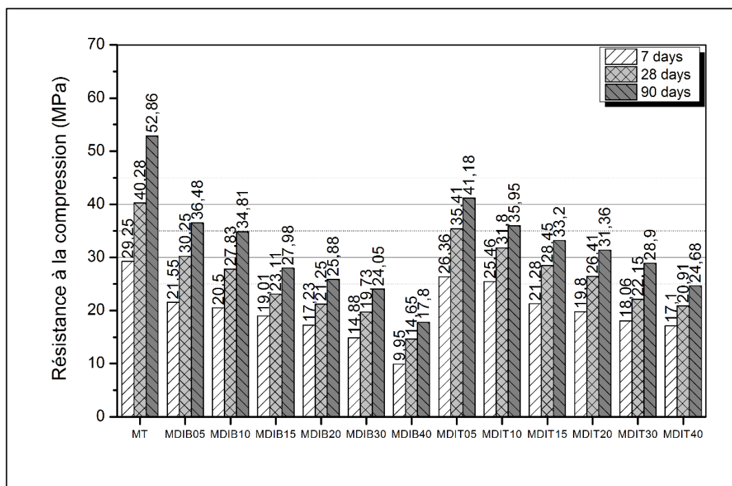
Figure 4.13 : Résistance à la compression des mortiers renforcés de fibres de Diss.
