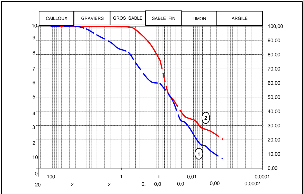
Annexe N° 01: diagrammes de l'analyse granulométriques sol 1 et le sol 2.
