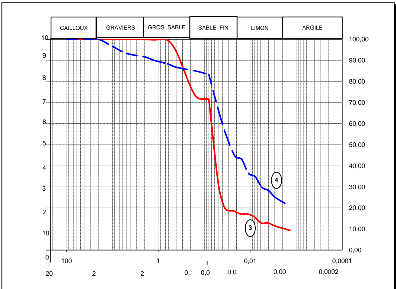
Annexe N° 04: diagrammes de l'analyse granulométriques sol 3 et le sol 4
