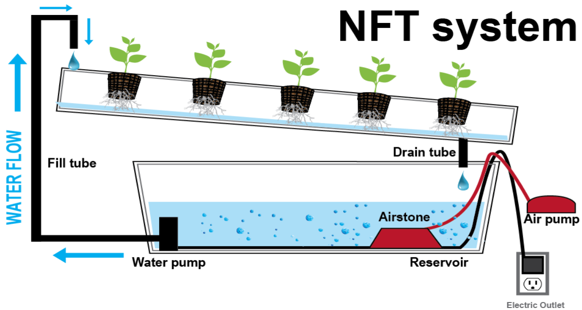
Figure 51: système NFT
